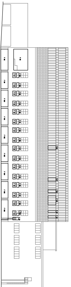
PROSPETTO OVEST
