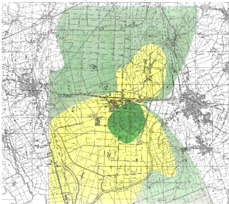
Figura 6.10 Distribuzione delle Concentrazioni Medie Annue di Mercurio in Aria, Stimate (scala arbitraria)
