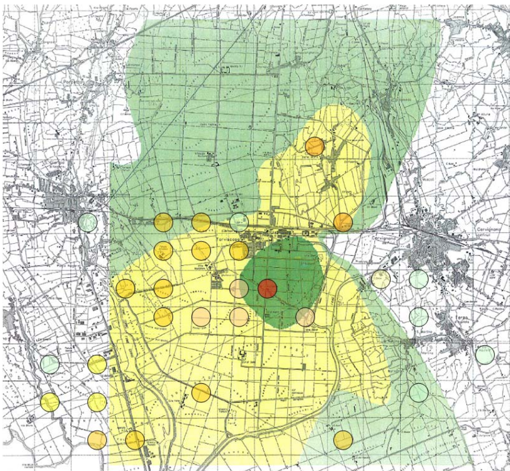
Figura 6.11 Distribuzione delle Concentrazioni di Mercurio Stimate in Atmosfera [scala arbitraria, in gradi di verde] e Misurate in Licheni Epifiti [scala arbitraria; in gradi di rosso]
