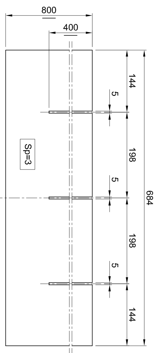
Part. "2" - Costruire N. 4 Pezzi
