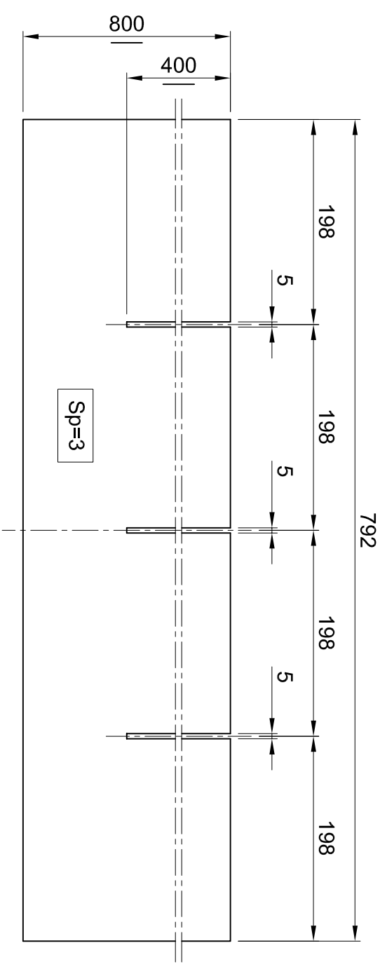
Part. "1" - Costruire N. 2 Pezzi
