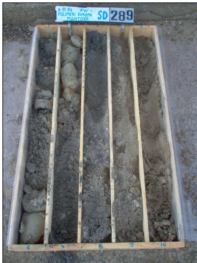
SD289: 5.00-10.00m
