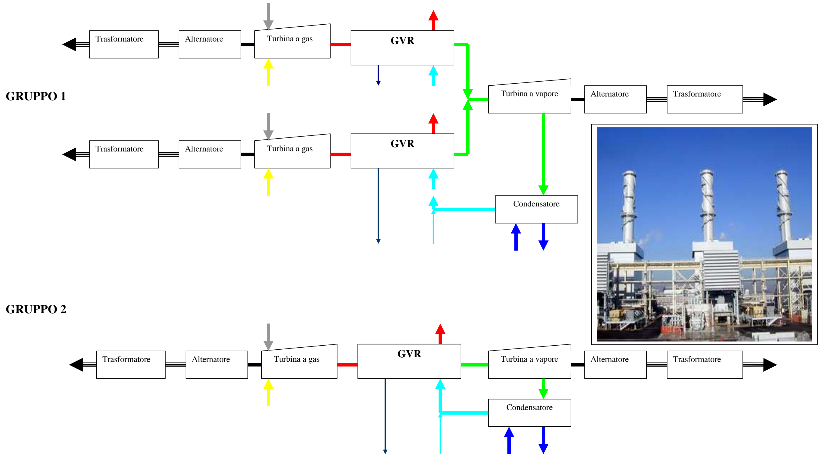
Figura 1 Schema Generale di Centrale
