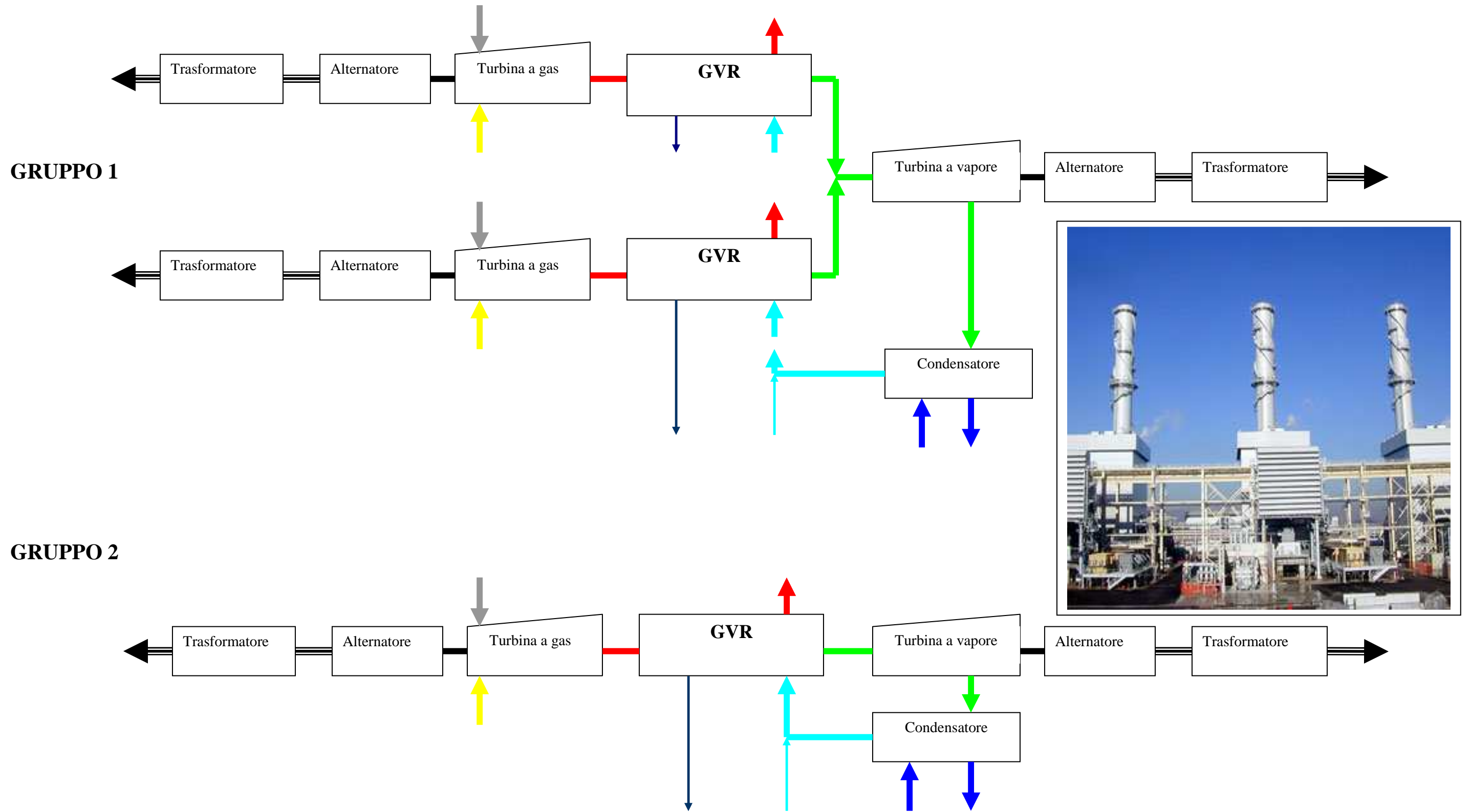
Figura 2 Schema Generale di Centrale
