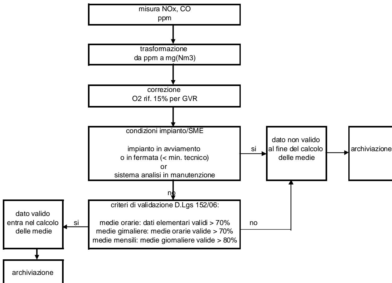
Figura 2 - Schema semplificato algoritmo elaborazione dati emissione camino turbogas (GVR)
