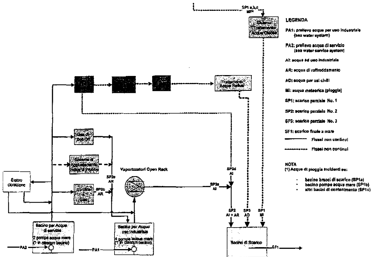
Figura 1: Approvvigionamento, Distribuzione e Scarico Acqua Mare (Rappresentazione Schematica)
