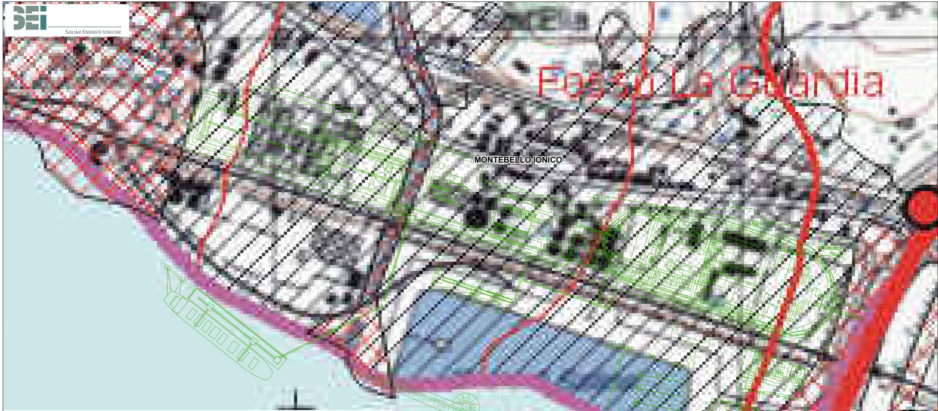
Punto 18a.5 - Piano Stralcio di Bacino per l'Assetto Idrogeologico Perimetrazione aree a rischio idraulico (estratto elaborato 14.4)
