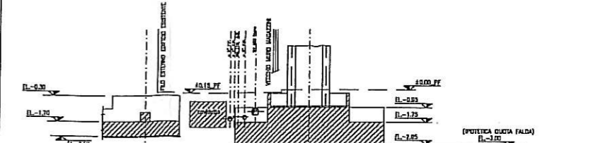
SEZIONE D-D
