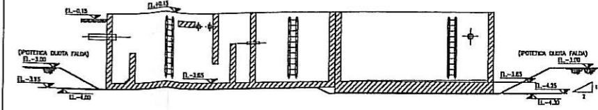
SEZIONE C-C
