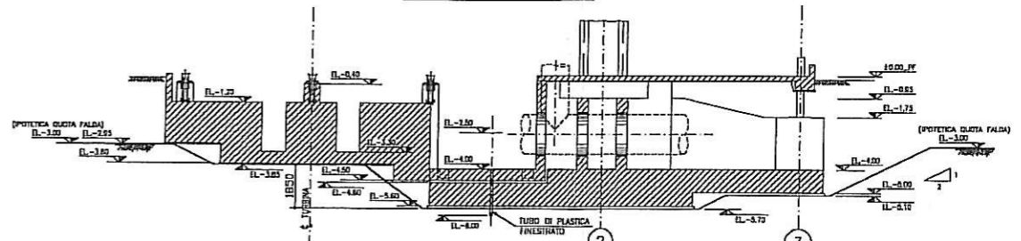
SEZIONE A-A
