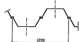
PROFILO PALANCOLA TIPO ARBED PU 16-PU 20
