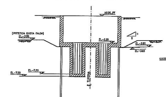
SEZIONE B-B
