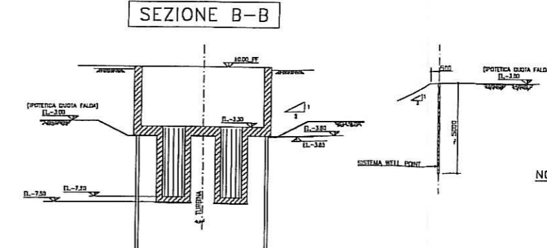
SEZIONE X-X
