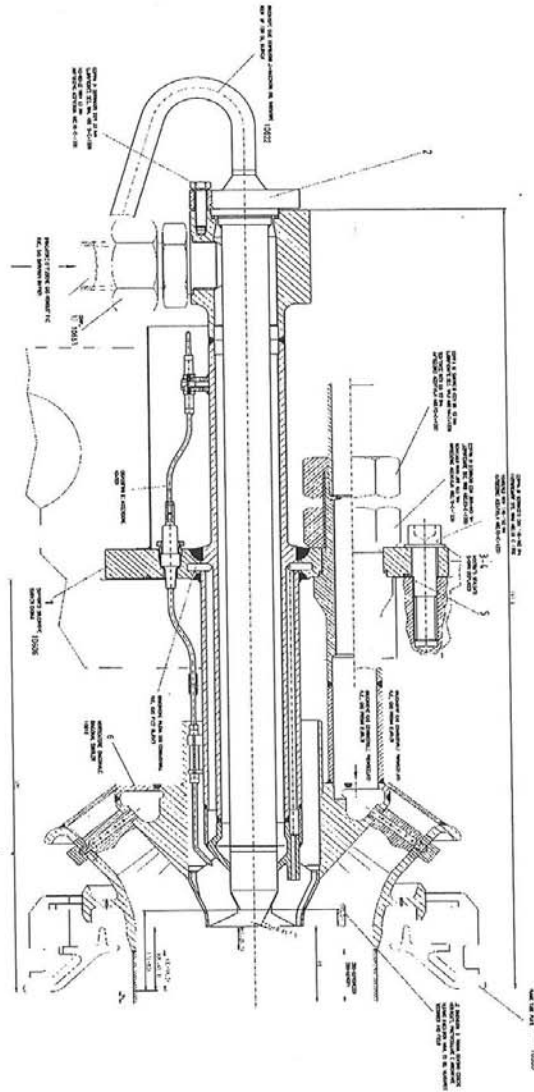
Figura 1: Assieme del Bruciatore VeLoNox
