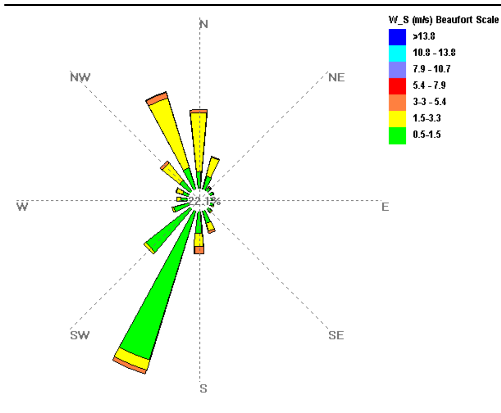
Figura 4a Rosa dei Venti, Centralina ARSSA di Gioia Tauro, Anno 2007
