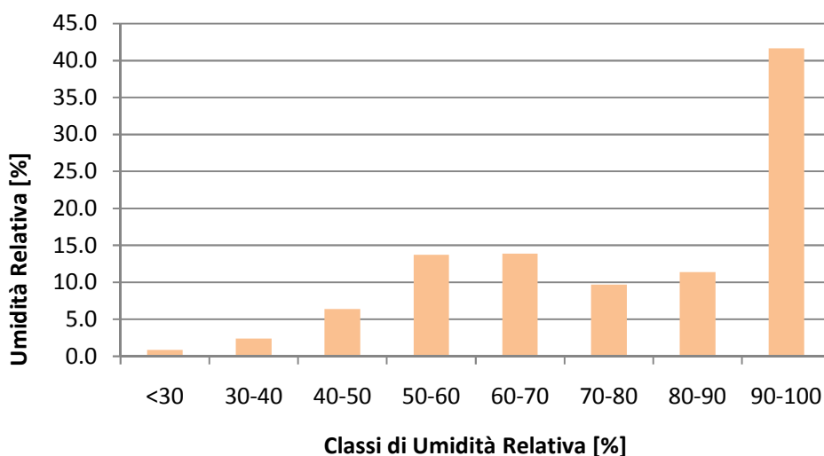
Figura 4e Distribuzione in Classi di Frequenza dei Valori di Umidità Relativa Registrati dalla Centralina ARSSA di Gioia Tauro - Anno 2007
