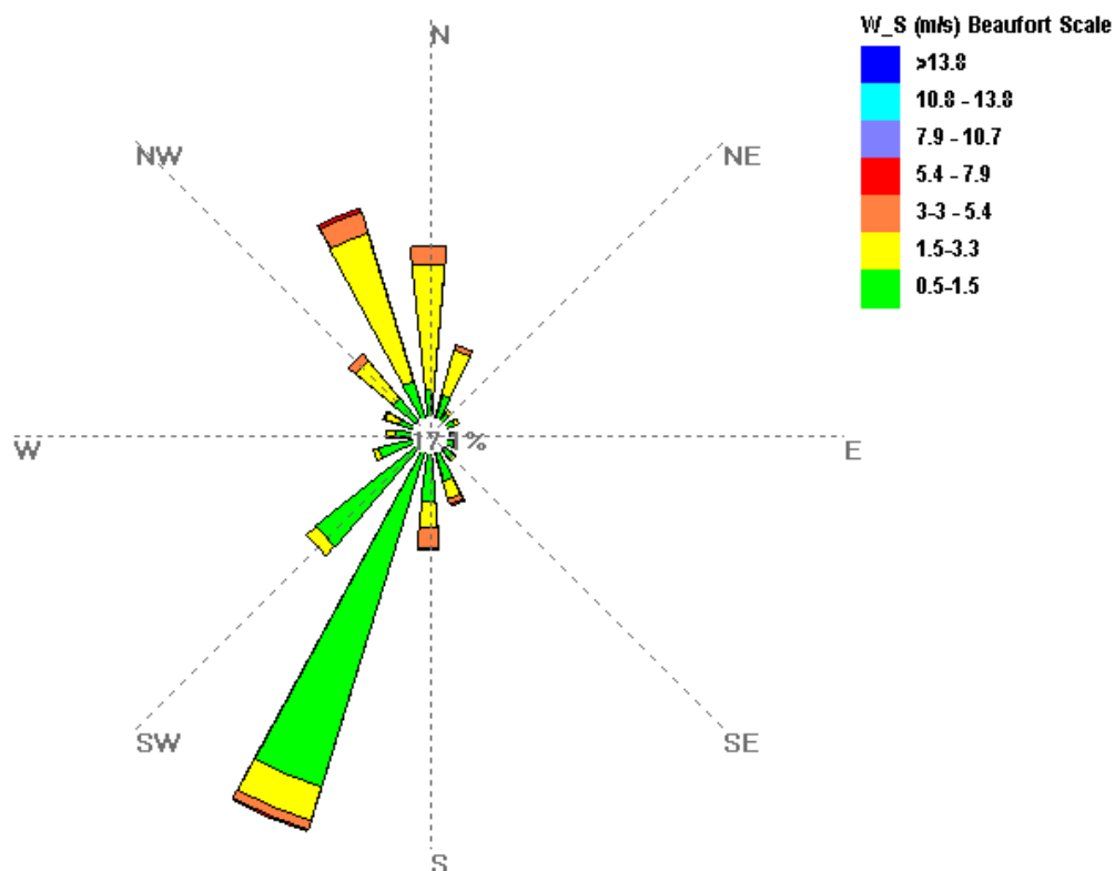
Figura 4f Rosa dei Venti Estratta dal Preprocessore Meteorologico CALMET in Corrispondenza della Centralina ARSSA di Gioia Tauro per l'Anno 2007
