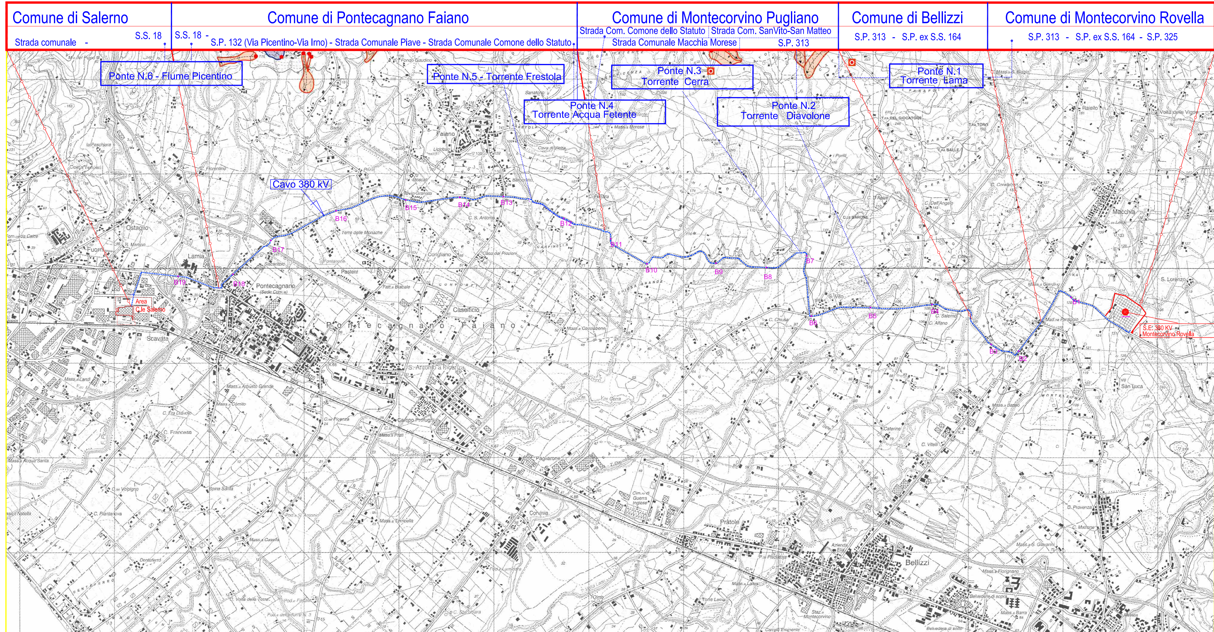
Corografia tracciato con buche giunti - Scala 1/25000
