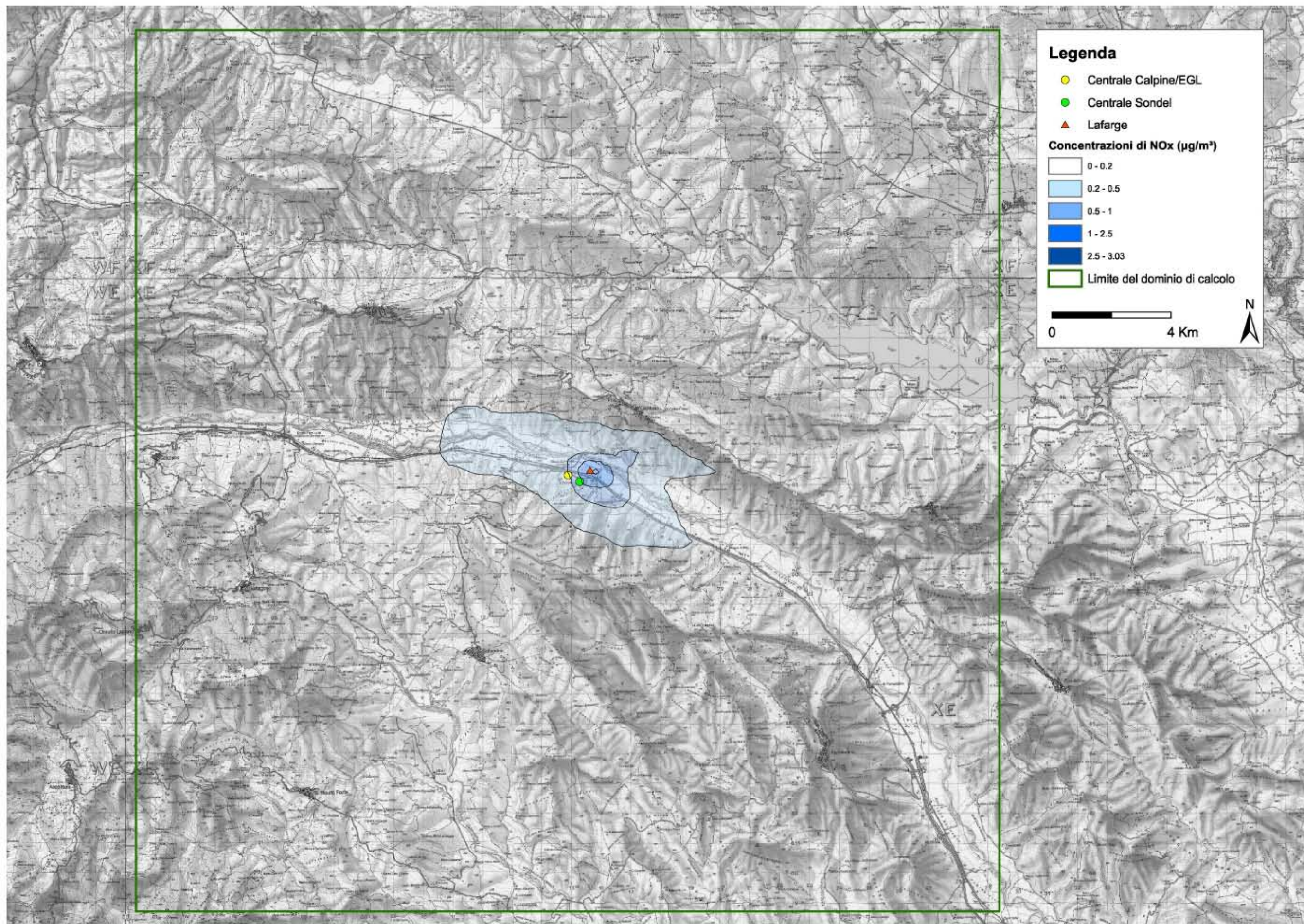
Figura 3.6.1.a Concentrazione Medie Annue ( \mu\text{g}/\text{m}^3 ); Scenario A: esercizio stabilimento Monier (ex Lafarge) – Centrale Basento Energia (ex Calpine-EGL) e Sondel non in funzione
