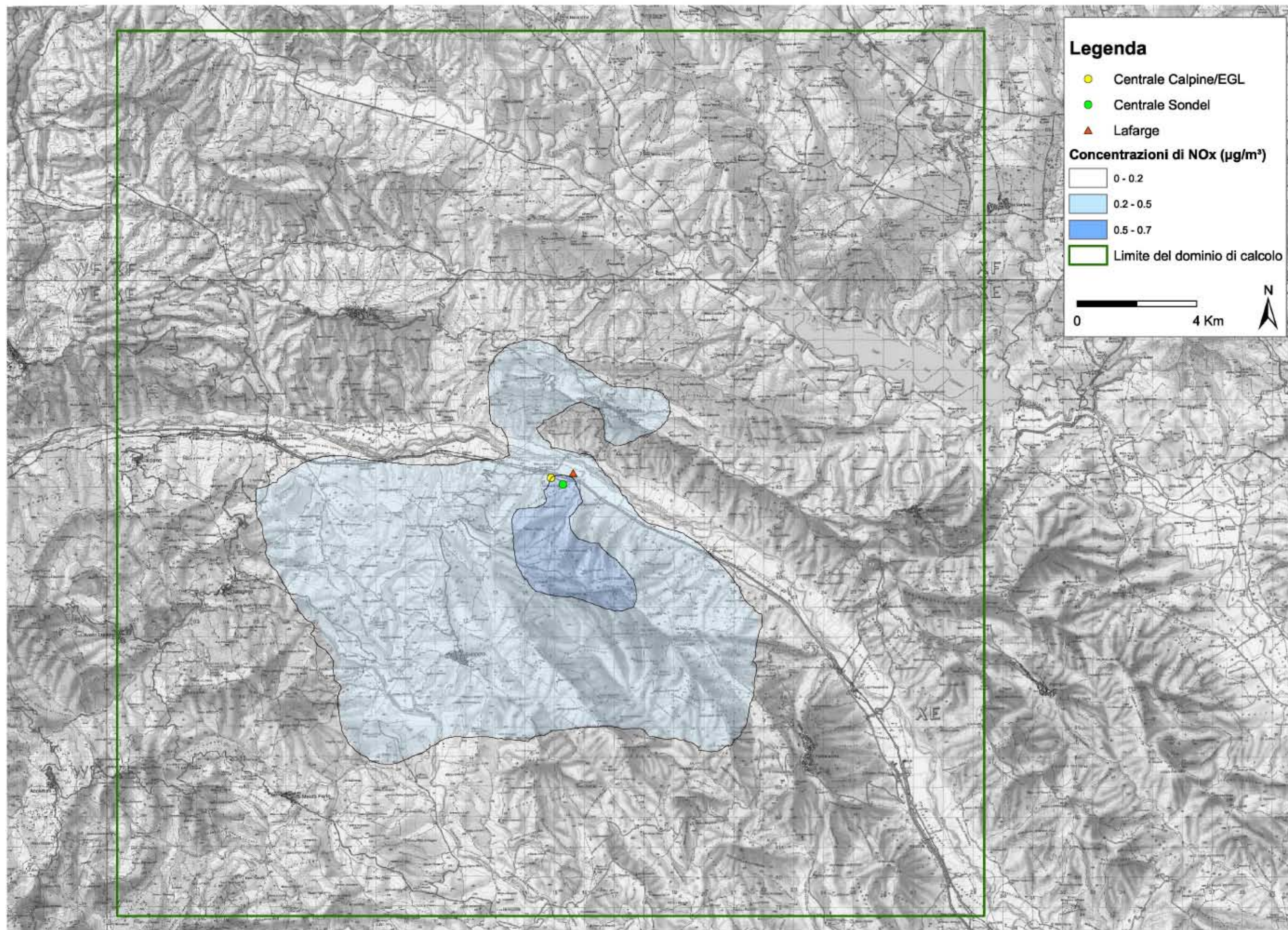
Figura 3.6.1.b Concentrazione Medie Annue ( \mu\text{g}/\text{m}^3 ); Scenario B: esercizio Centrale Basento Energia (ex Calpine-EGL) - stabilimento Monier (ex Lafarge) e centrale Sondel non in funzione
