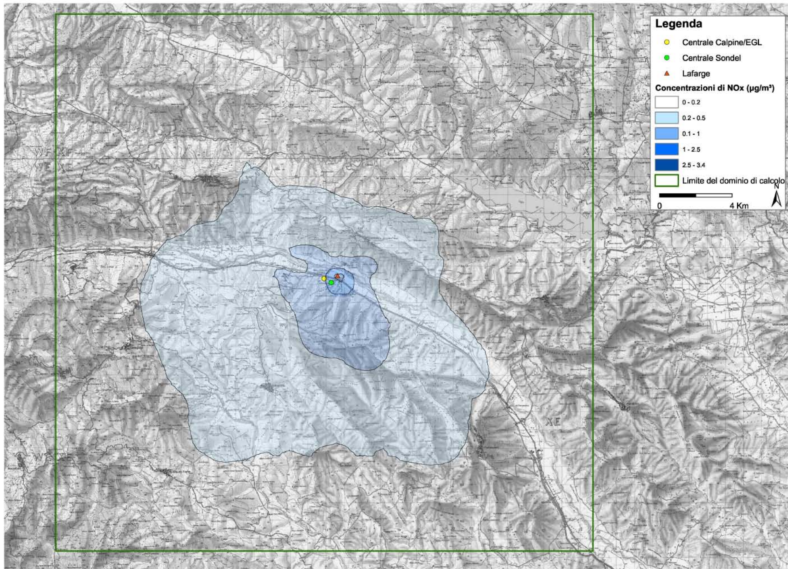
Figura 3.6.1.c Concentrazione Medie Annue ( \mu\text{g}/\text{m}^3 ); Scenario C: esercizio stabilimento Monier (ex Lafarge) e Centrale Basento Energia (ex Calpine-EGL) - Centrale Sondel non in funzione
