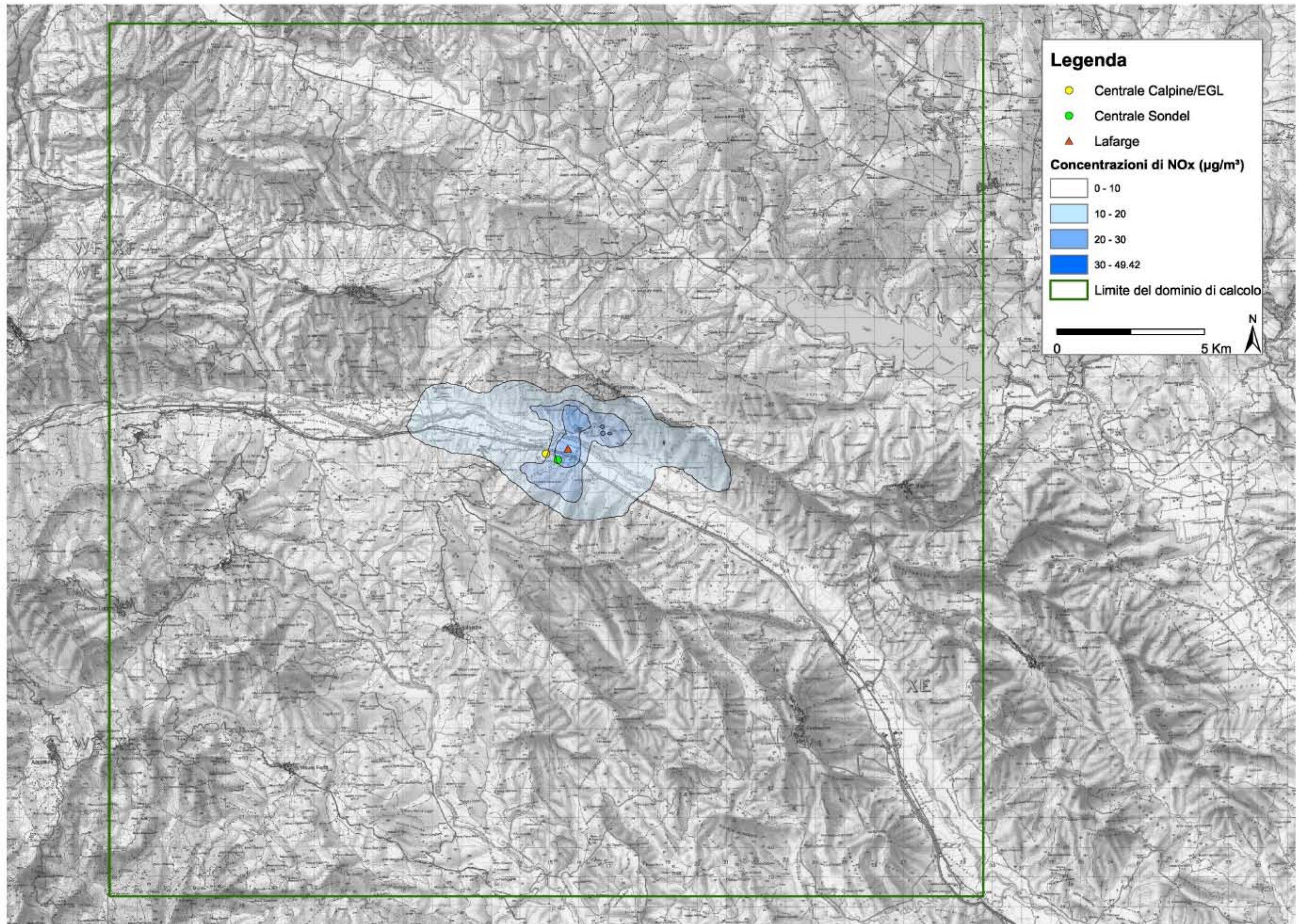
Figura 3.6.2.a 99,8°Perc. Concentrazioni Medie Orarie ( \mu\text{g}/\text{m}^3 ); Scenario A: esercizio stabilimento Monier (ex Lafarge) – Centrale Basento Energia (ex Calpine-EGL) e Sondel non in funzione
