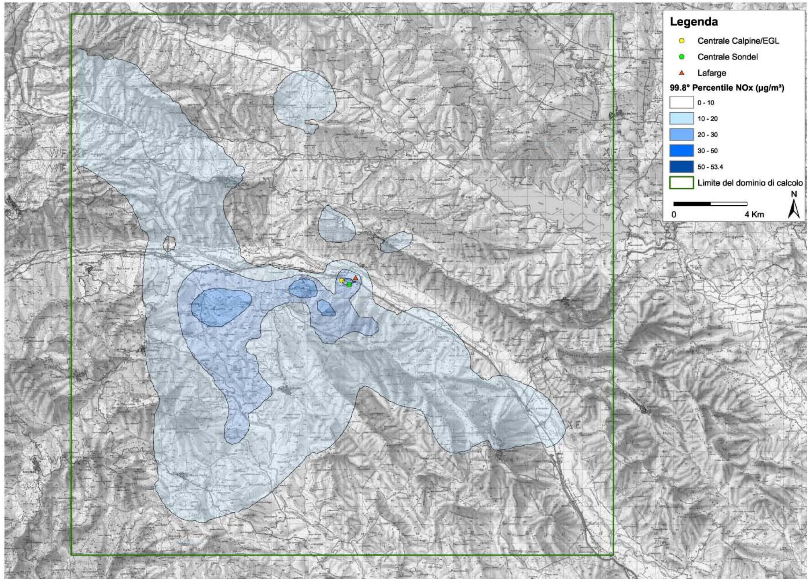
Figura 3.6.2.b 99,8°Perc. Concentraz. Medie Orarie ( \mu\text{g}/\text{m}^3 ); Scenario B: esercizio Centrale Basento Energia (ex Calpine-EGL) - stabilimento Monier (ex Lafarge) e centrale Sondel non in funzione
