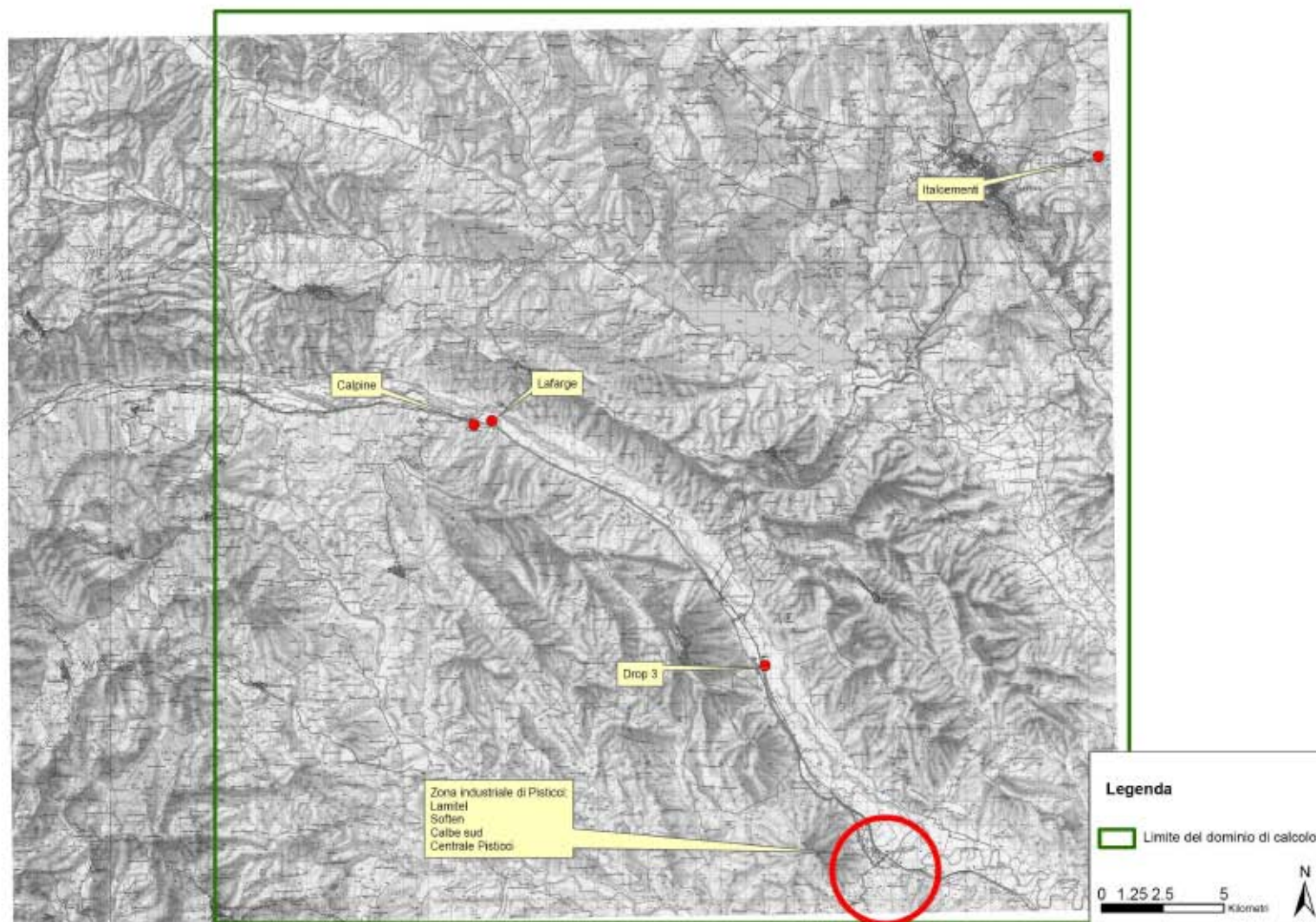
Figura 3.a Localizzazione delle sorgenti emissive significative
