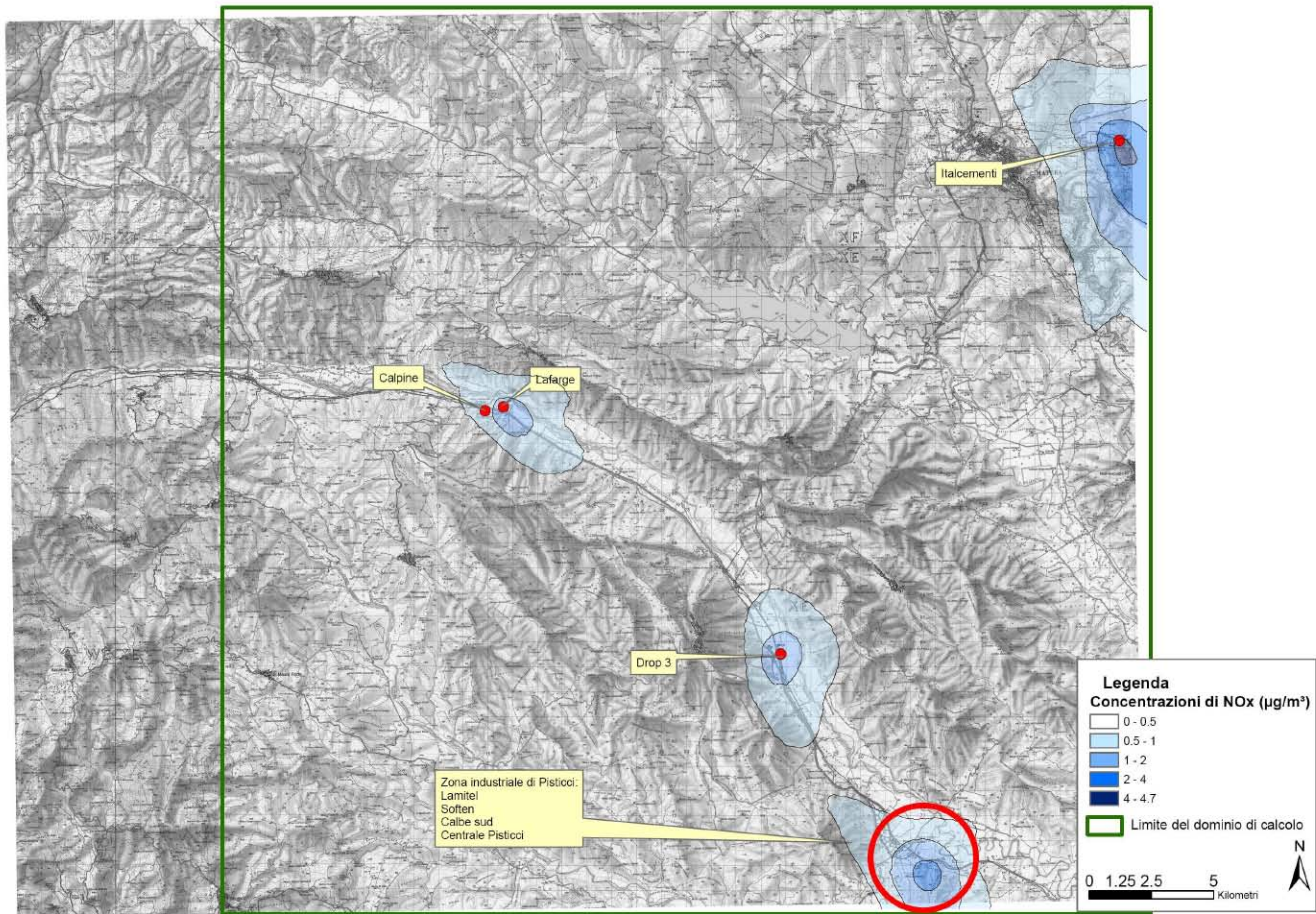
Figura 6.1.a Concentrazioni medie annue di NOx nello scenario attuale
