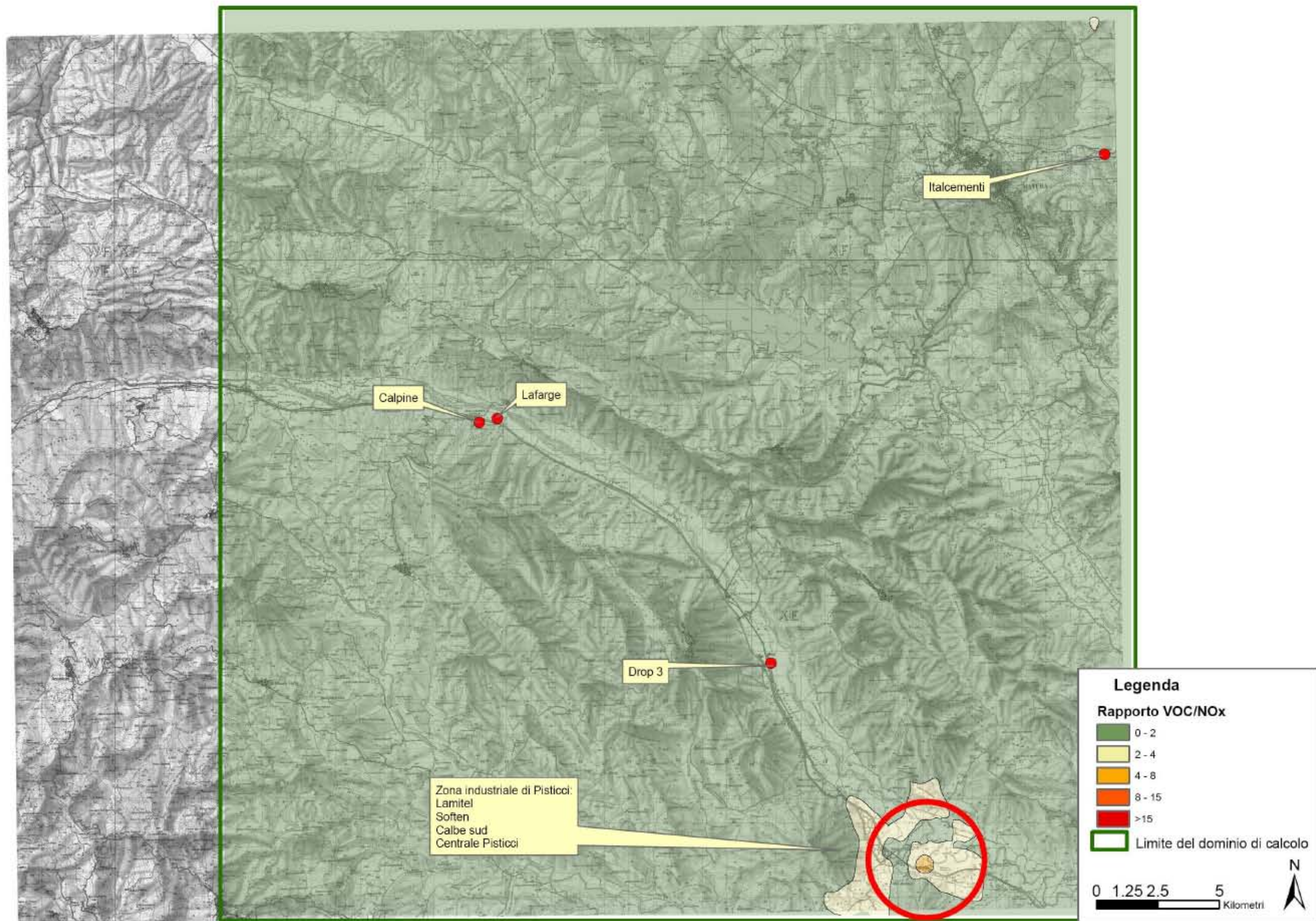
Figura 6.1.d Rapporto tra le concentrazioni medie annue di VOC e NOx nello scenario attuale
