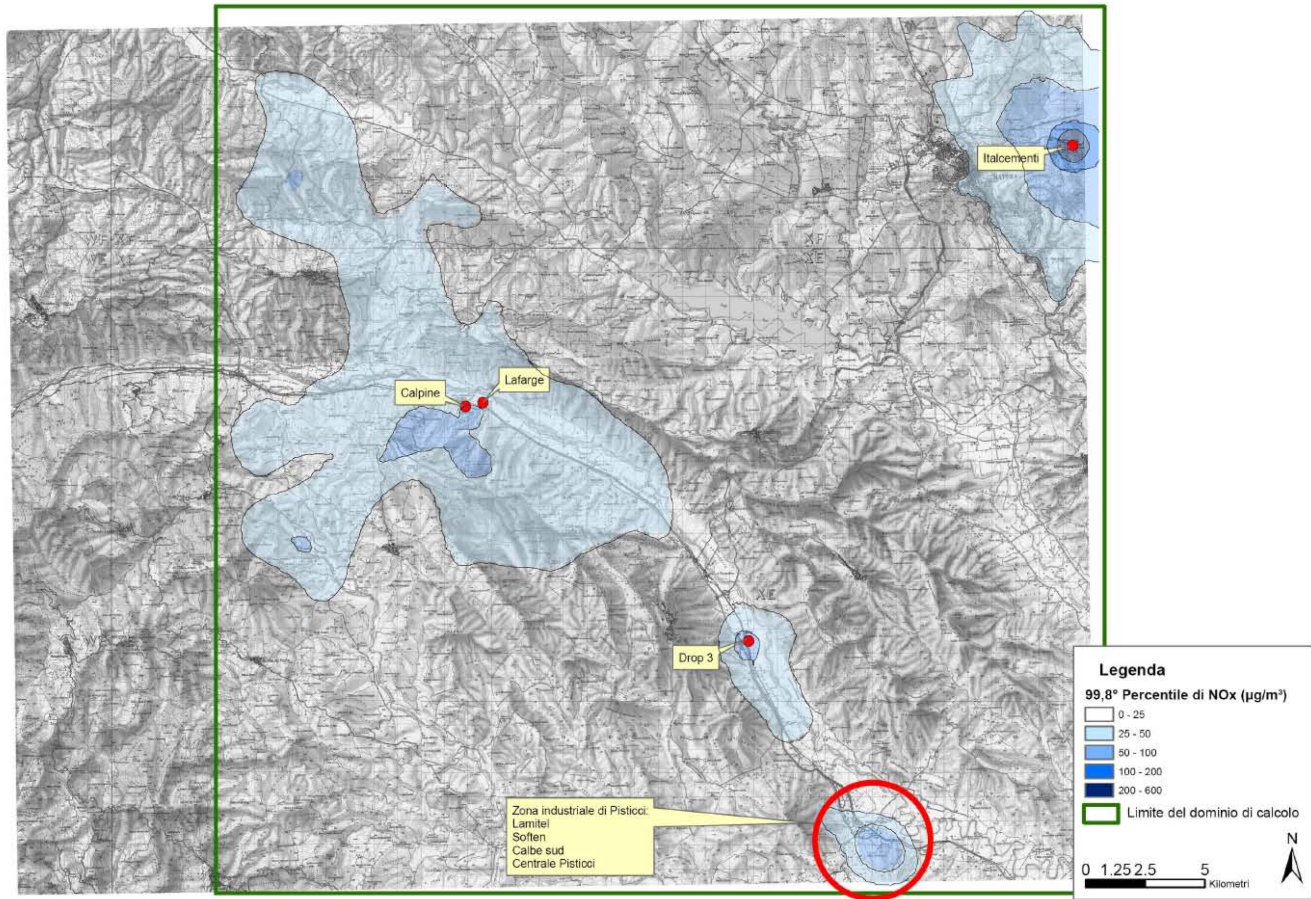
Figura 6.2.b 99,8° Percentile delle concentrazioni medie omrie di NOx nello scenario futuro
