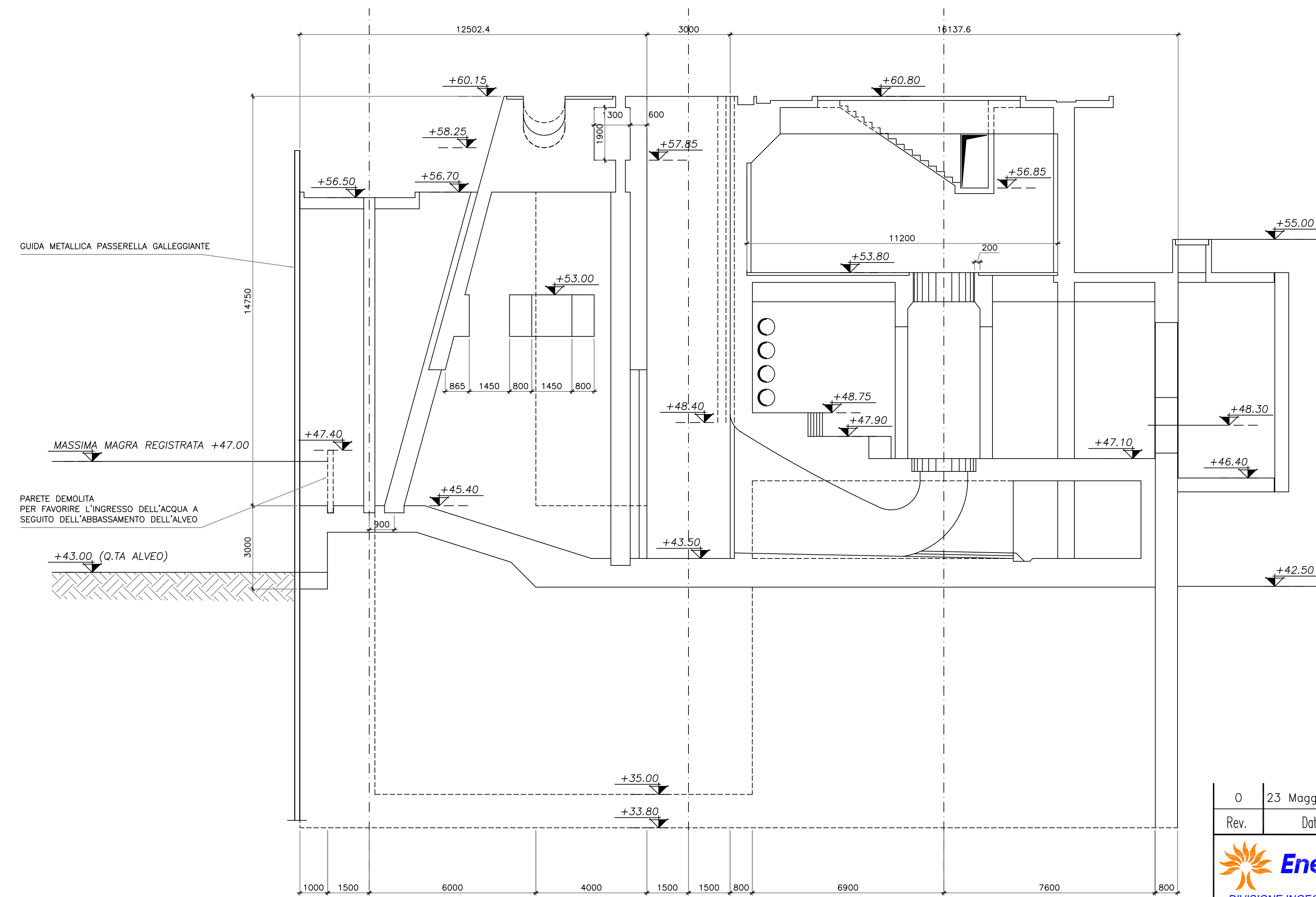
SEZIONE A-A
