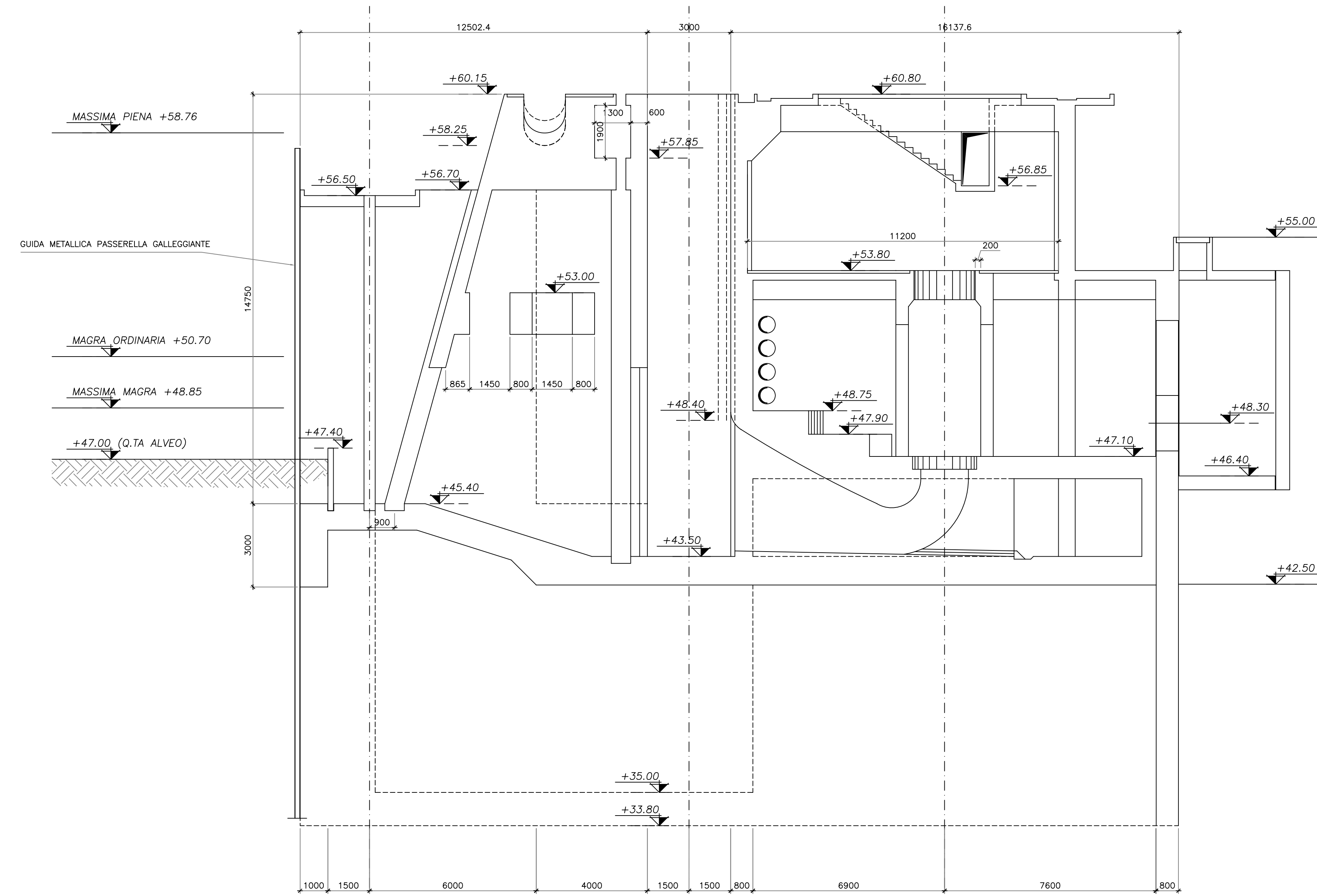
SEZIONE A-A
