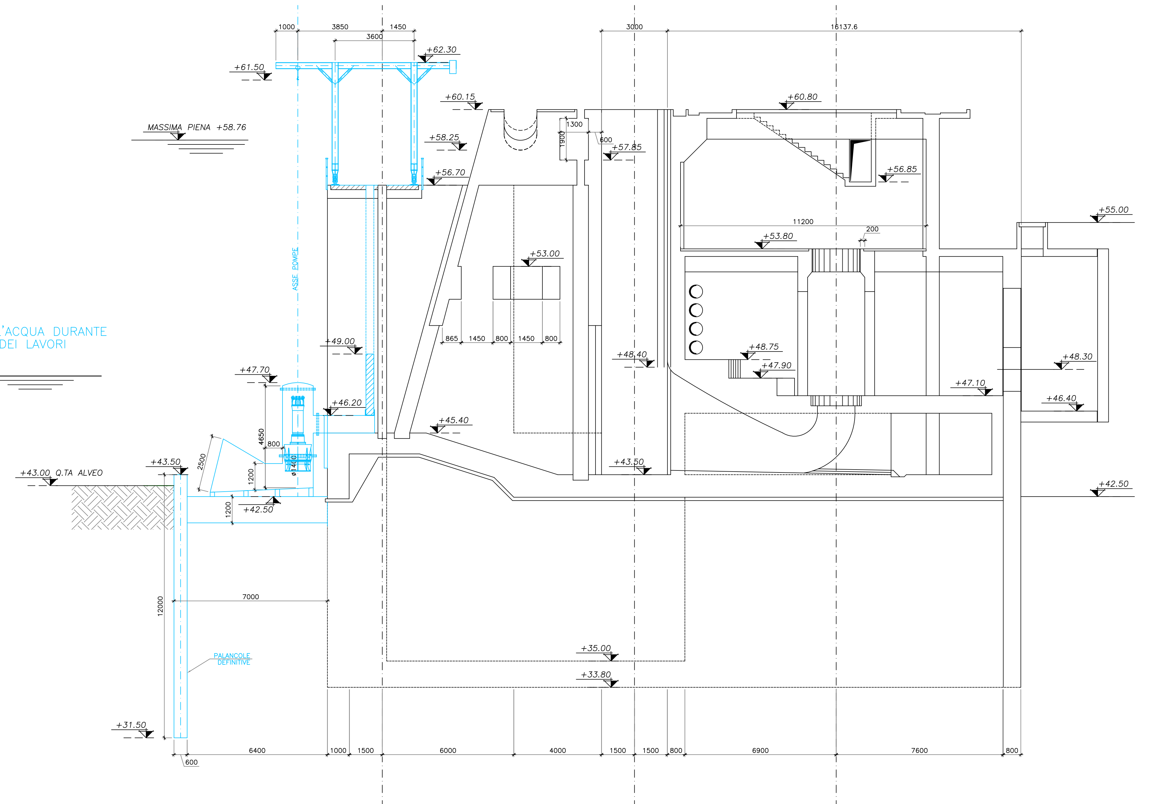
SEZIONE A-A
