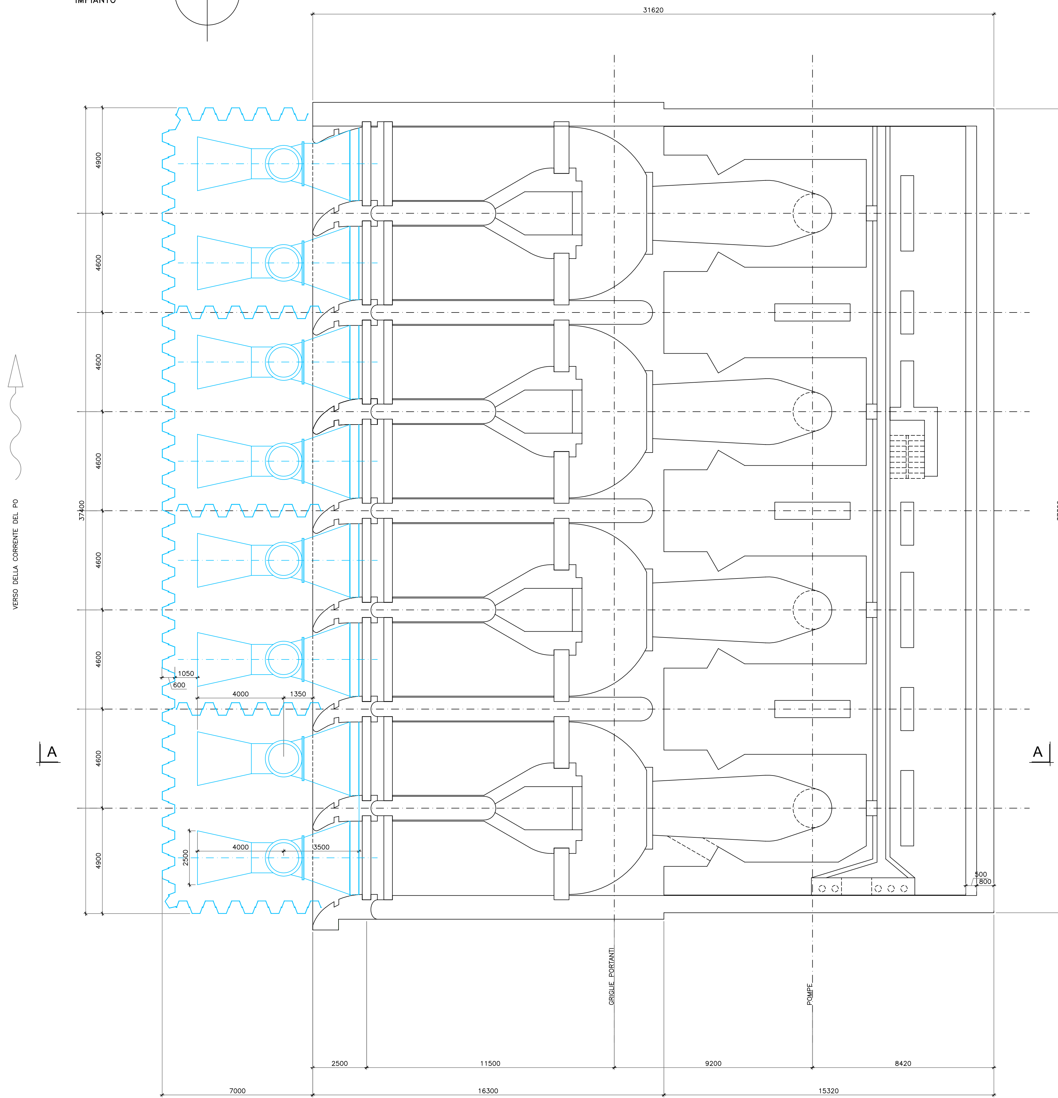
PIANTA A Q.T.A. -45.00
