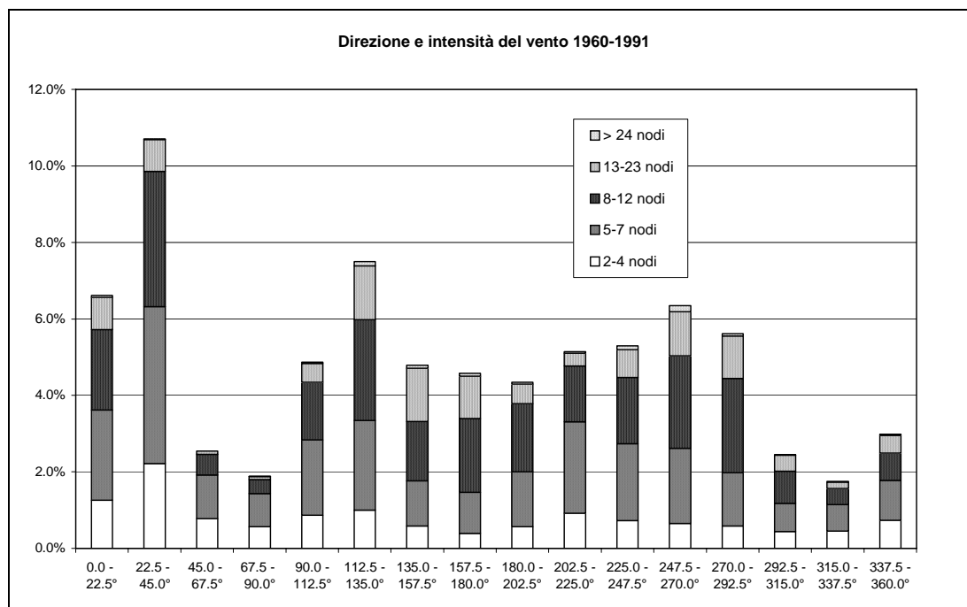
FIGURA 3 - CLASSI DI INTENSITÀ DEL VENTO (NODI) PER CIASCUNA DIREZIONE DI PROVENIENZA - STAZIONE DI PRATICA DI MARE - PERIODO DI OSSERVAZIONE 1960-1991
