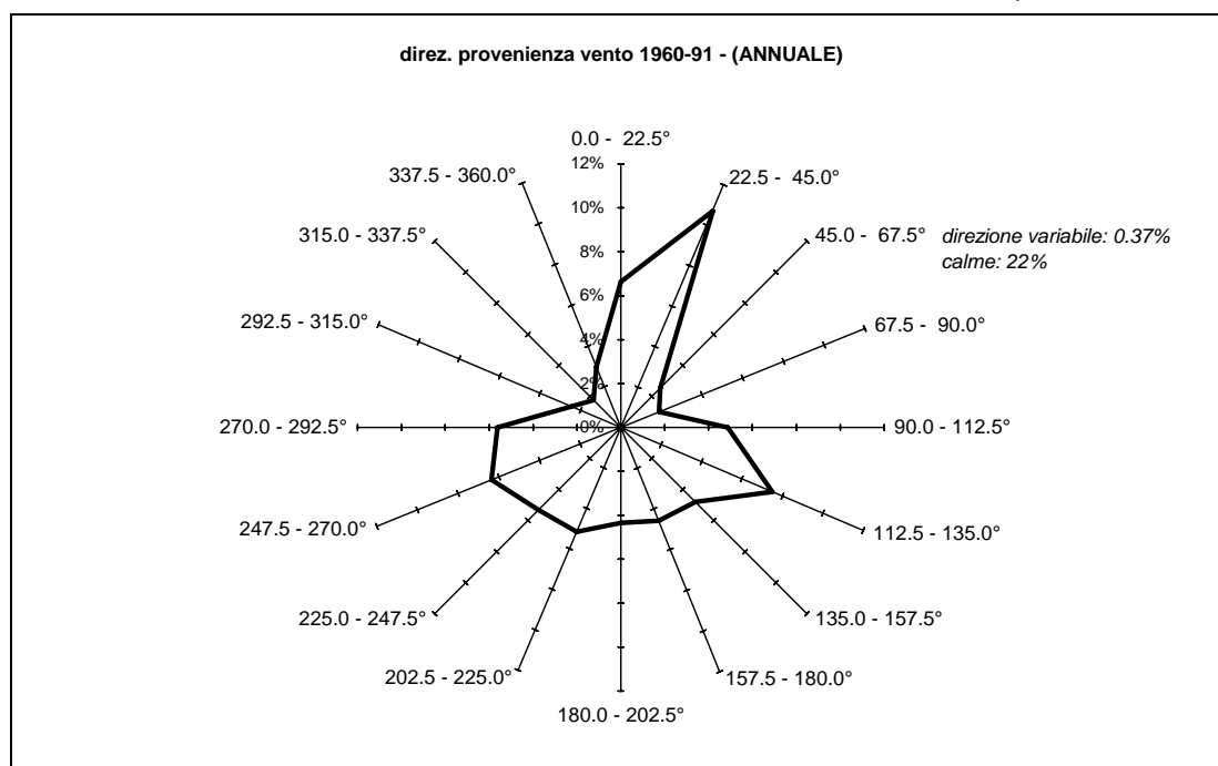
FIGURA 2 - DIREZIONE DI PROVENIENZA DEL VENTO STAZIONE DI PRATICA DI MARE (FONTE SERVIZIO METEOROLOGICO AERONAUTICA MILITARE - PERIODO DI OSSERVAZIONE 1960-1991)
