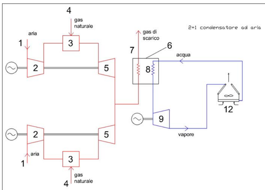
1 Aria comburente; 2 Compressore; 3 Combustore; 4 Gas combustibile; 5 Turbina a gas (espansore); 6 Caldaia a recupero; 7 Scarico fumi al camino; 8 Generatore di vapore; 9 Turbina a vapore; 12 Condensatore ad aria
