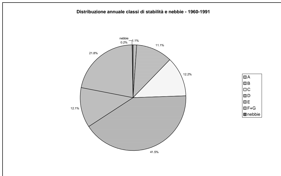
FIGURA 4 – CLASSI DI STABILITÀ: DISTRIBUZIONE DELLE FREQUENZE ANNUALI STAZIONE DI PRATICA DI MARE (ANNI 1960-1991)
