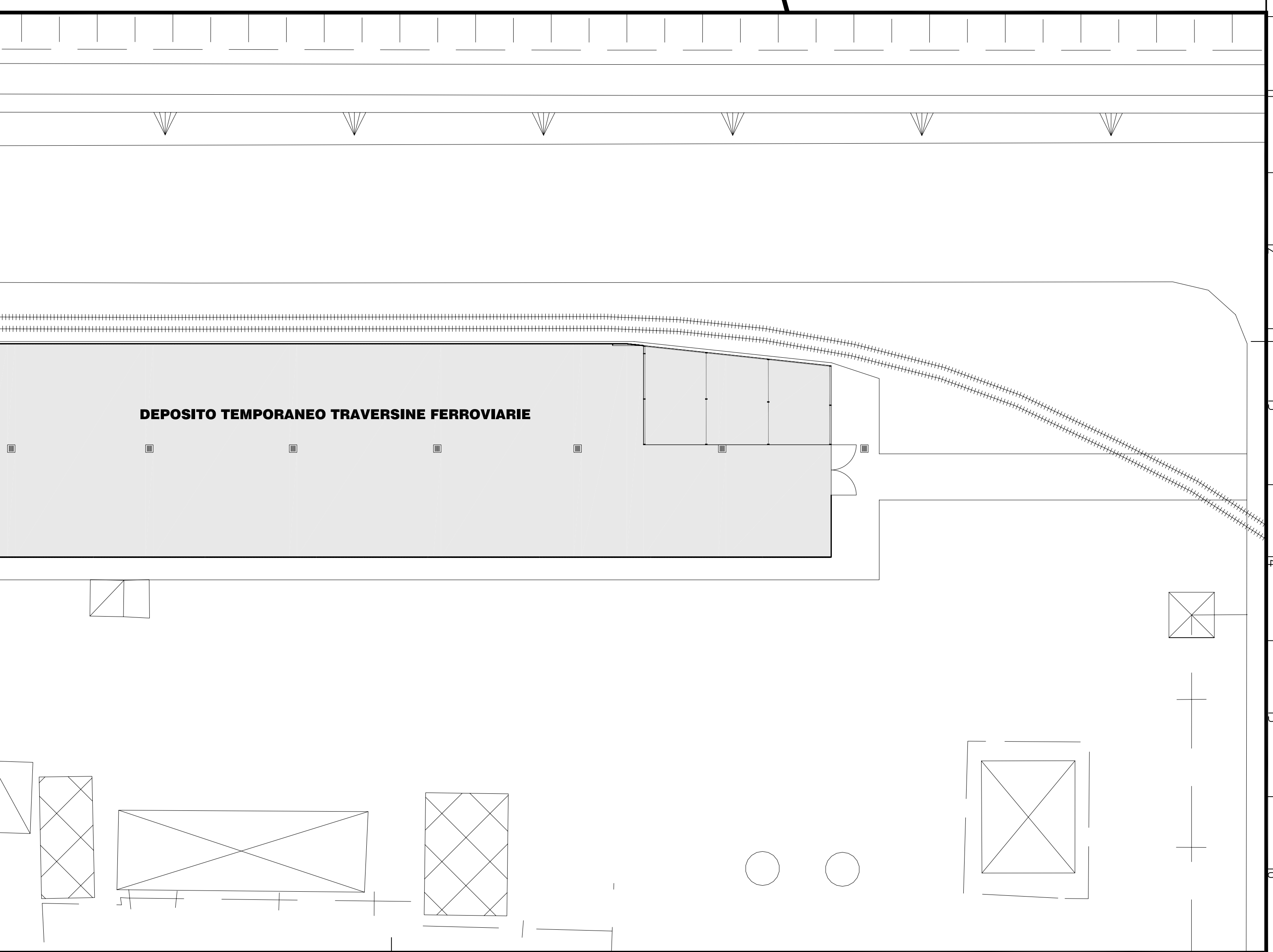
PLANIMETRIA UBICAZIONE SCALA 1:400
