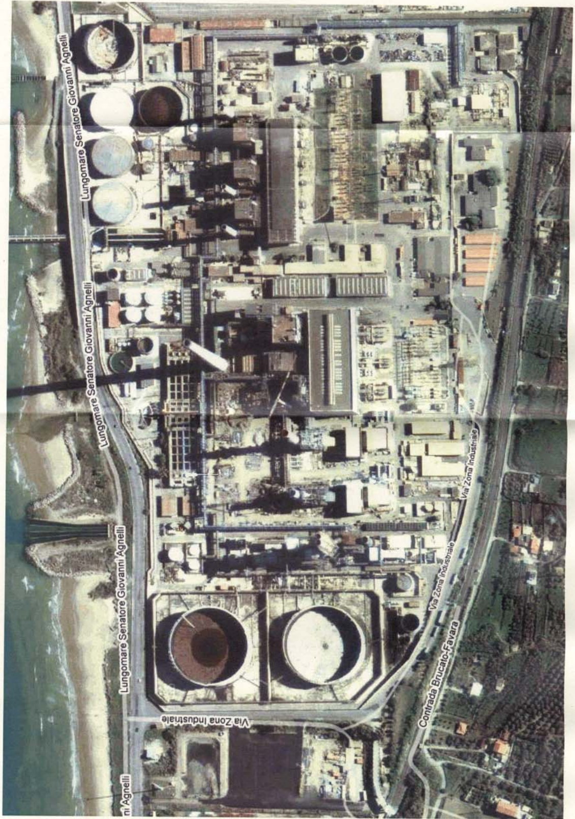
FIGURA 5 - VISTA DA SATELLITE DELLA CENTRALE DI TERMINI IMERESE
