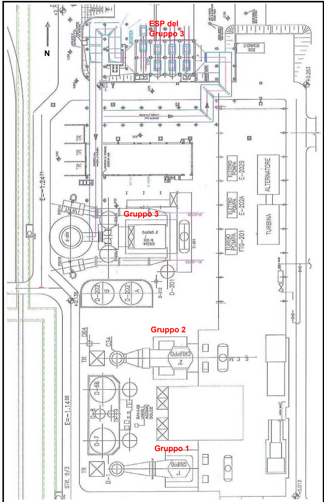
Figura 1.1a Schema in pianta dei 3 gruppi della centrale SA1Nord (SA1N/1, SA1N/2, SA1N/3)
