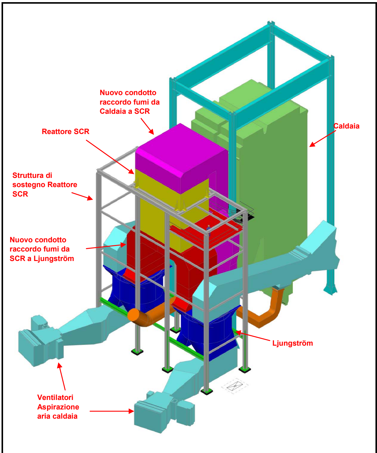
Figura 5.1.2b Modello 3D degli interventi previsti
