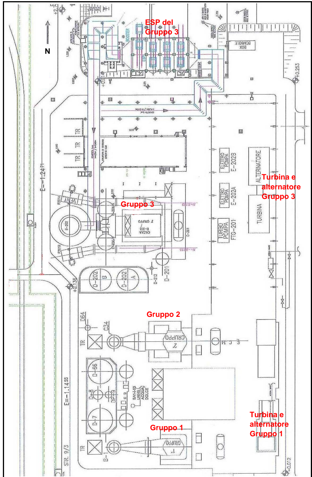
Schema in Pianta dei 3 gruppi della Centrale SA1Nord (SA1N/1, SA1N/2, SA1N/3)
