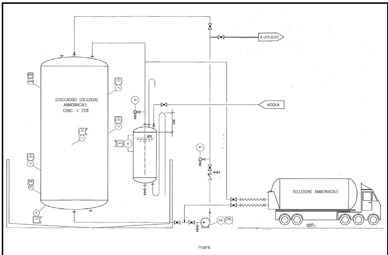
Figura 5.1.2c Ricezione e stoccaggio soluzione ammoniacale
