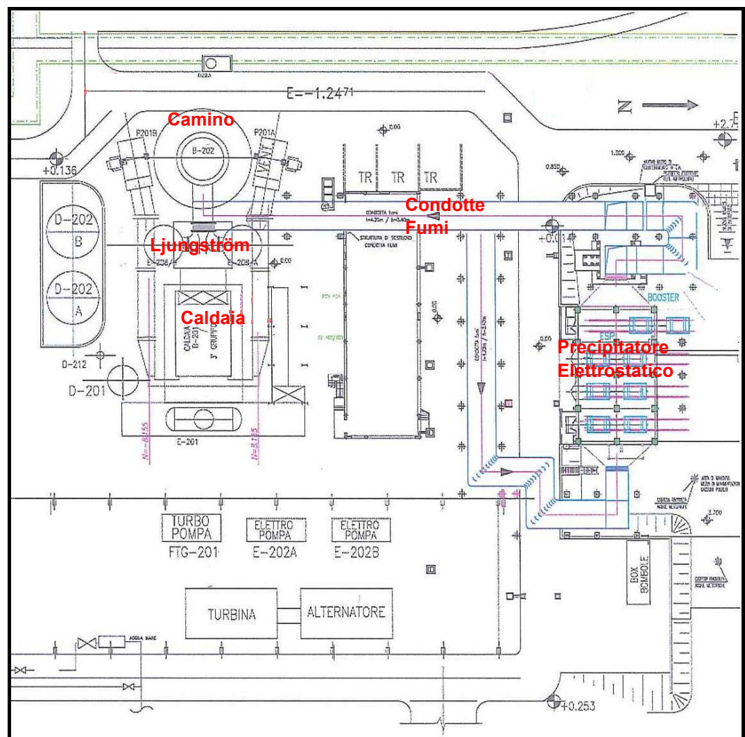
Figura 4.1a Disposizione nel Sito delle apparecchiature che costituiscono il gruppo SA1N/3
