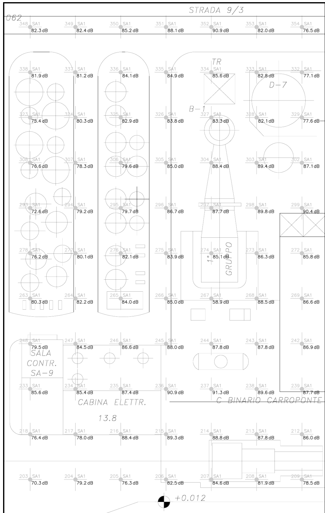
Figura 6.6.2a Ubicazione delle Postazioni di Misura in Prossimità della Caldaia del Gruppo SA1N/1
