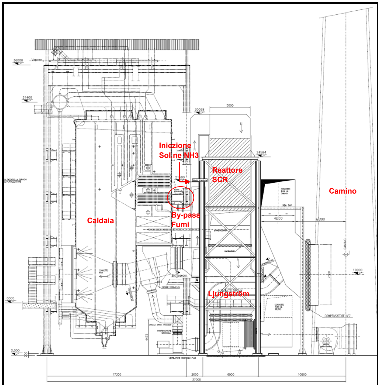
Figura 5.1.2a Posizionamento del reattore SCR nel gruppo SA1N/3
