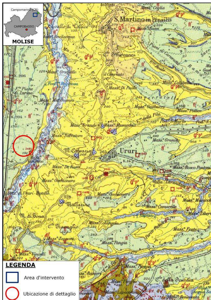
Figura 3 – Stralcio della Carta Geologica d'Italia in scala 1:100.000 (Foglio 155 "San Severo")
