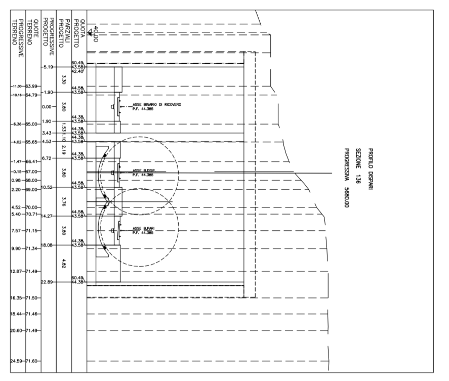
Imbocco Galleria S. Cecilia lato Ponte scala 1:500
