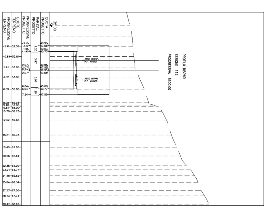
Imbocco Galleria S. Agata lato Messina scala 1:500
