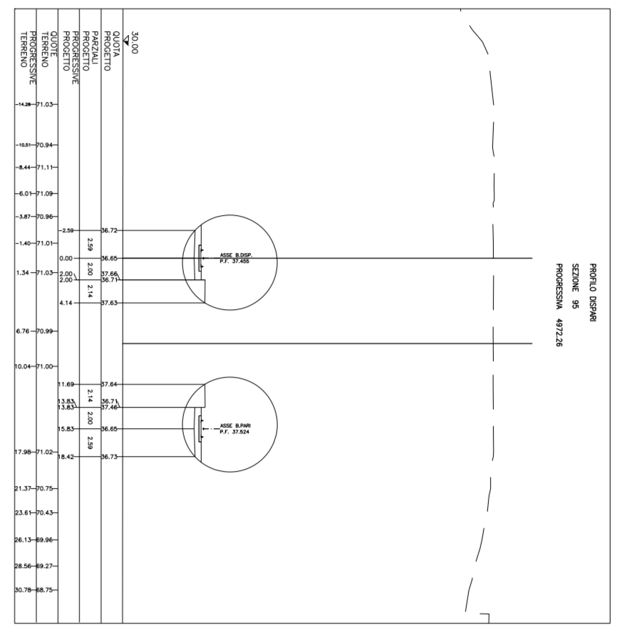
Galleria naturale S. Agata scala 1:500
