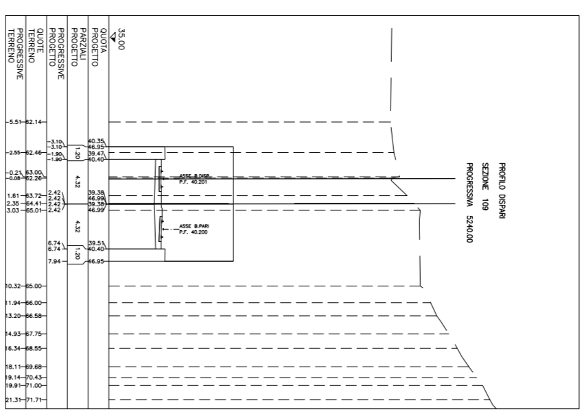
Galleria artificiale S. Agata scala 1:500
