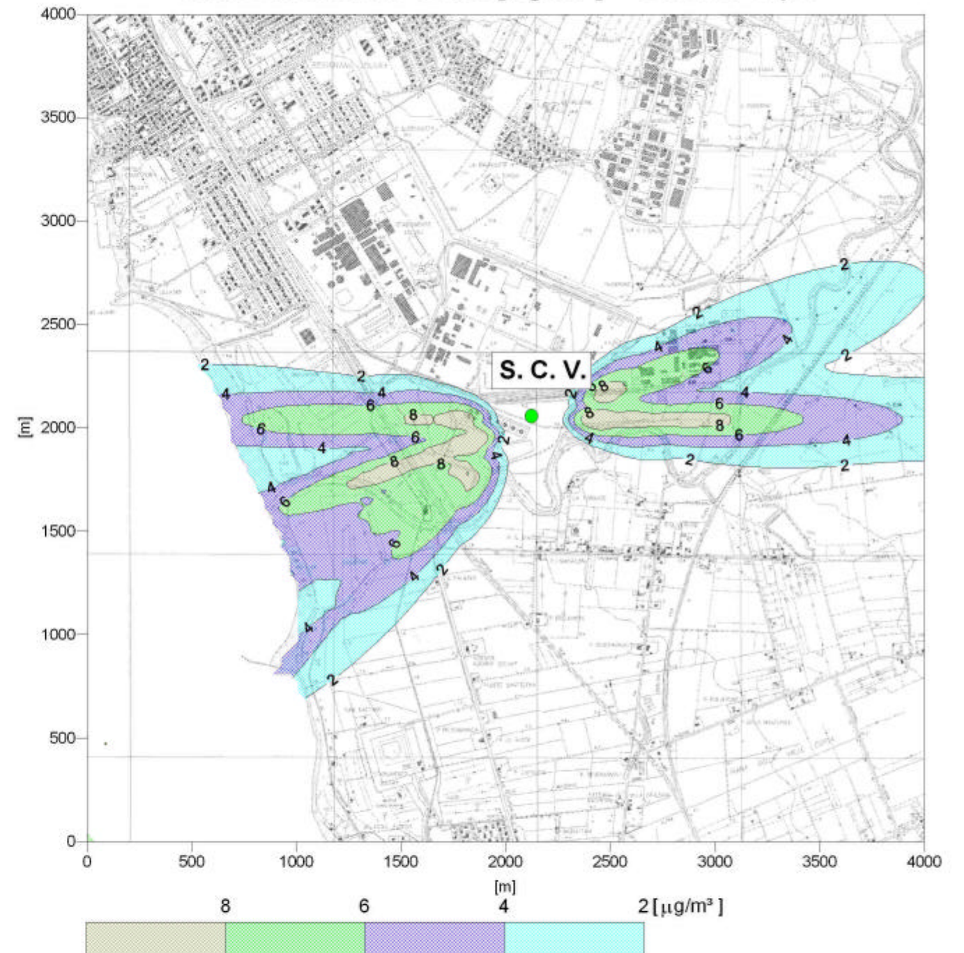
FIGURA 4.2 STUDIO DI IMPATTO AMBIENTALE SINTESI NON TECNICA VARIANTE PROGETTO ROSIGNANO ANALISI DI DISPERSIONE DI INQUINANTI INVILUPPO DELLE CONCENTRAZIONI MASSIME ORARIE DI NOx E CO IN ATMOSFERA AL LIVELLO DEL SUOLO GIORNO TIPO PREPARATO PER EDISON S.p.A. MILANO
