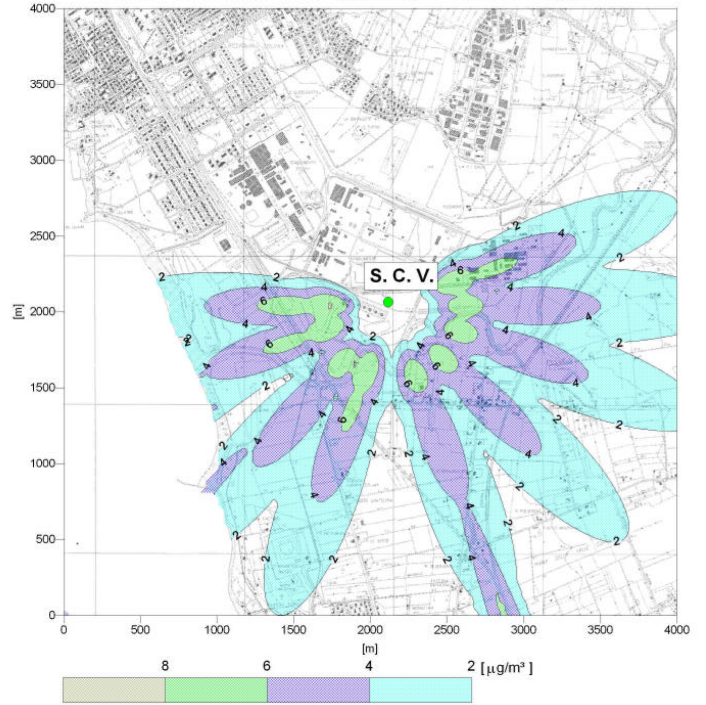
FIGURA 4.3 STUDIO DI IMPATTO AMBIENTALE SINTESI NON TECNICA VARIANTE PROGETTO ROSIGNANO ANALISI DI DISPERSIONE DI INQUINANTI INVILUPPO DELLE CONCENTRAZIONI MASSIME ORARIE DI NOx E CO IN ATMOSFERA AL LIVELLO DEL SUOLO GIORNO PEGGIORE PREPARATO PER EDISON S.p.A. MILANO
