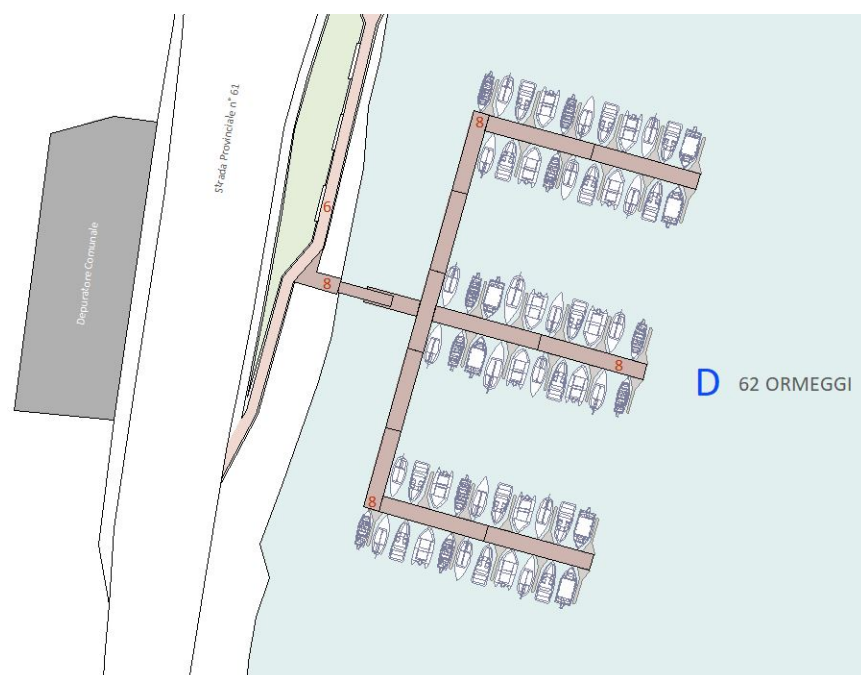
Pontile in progetto nell’ansa di Brusimpiccolo, presso la camminata spondale esistente.
