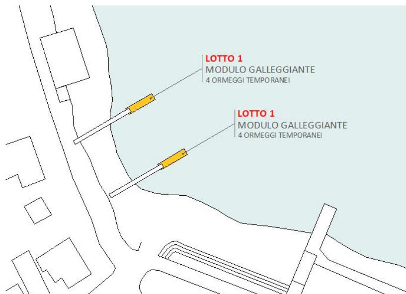
Struttura per ormeggio imbarcazioni temporanee nell'area Nord di Brusimpiano
