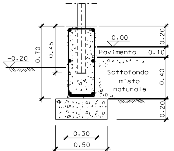
SEZIONE TIPO MURETTO
