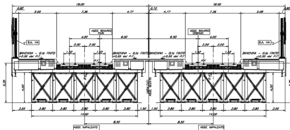
SEZIONE TIPICA CAMPATA 50m Scala 1:100
