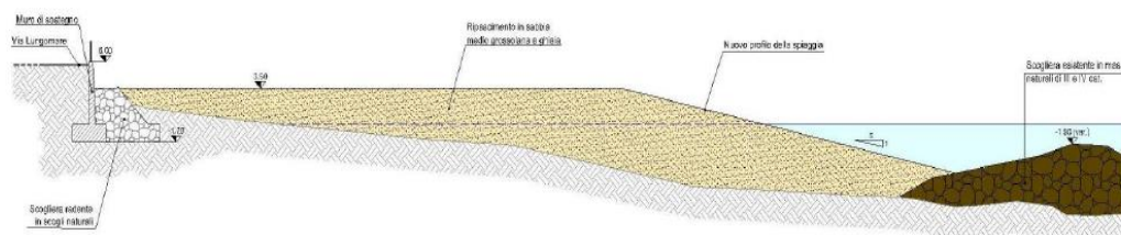
Figura 6 - Sezione tipologica ripascimento
