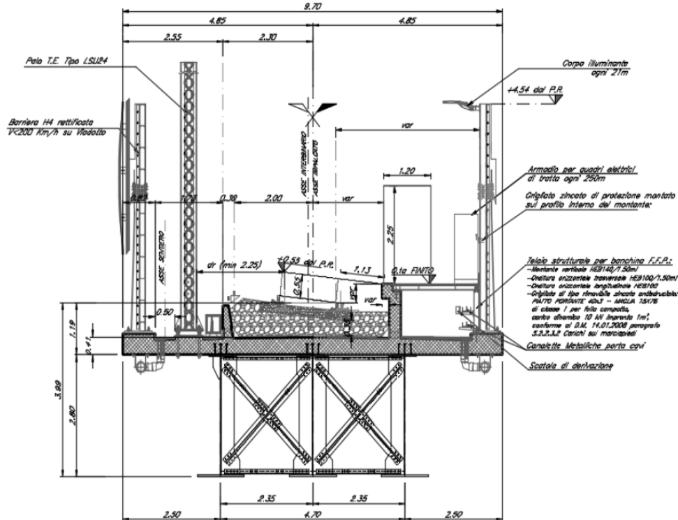
SEZIONE TRASVERSALE TIPOLOGICA BINARIO PARI CAMPATA IN ACCIAIO Scala 1:50
