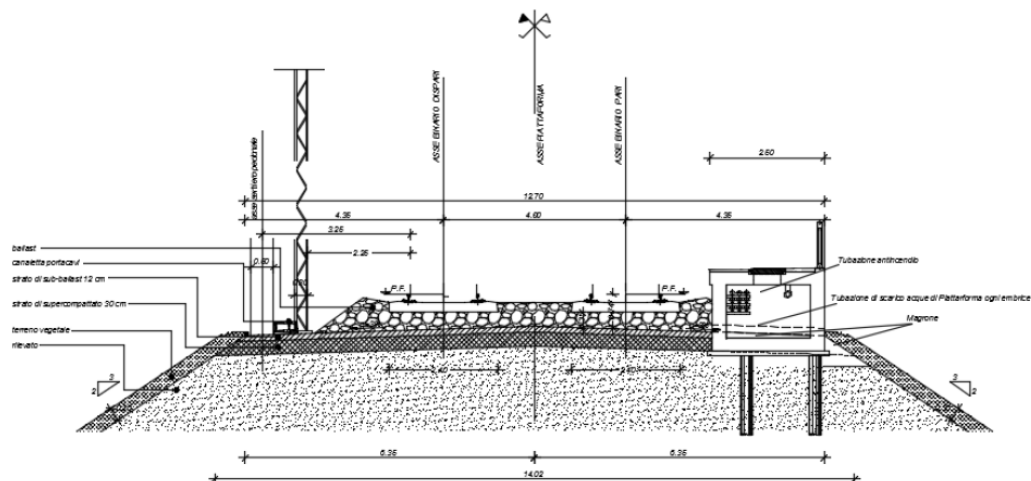
Figura 9 – Sezione Tipo in Rilevato con marciapiedi FFP/galleria equivalente
