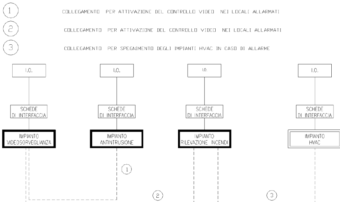
Figura 7: Schema delle interfacce con gli altri impianti
