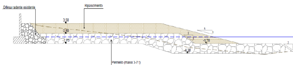
Figura 5 - Profilo longitudinale pennello
