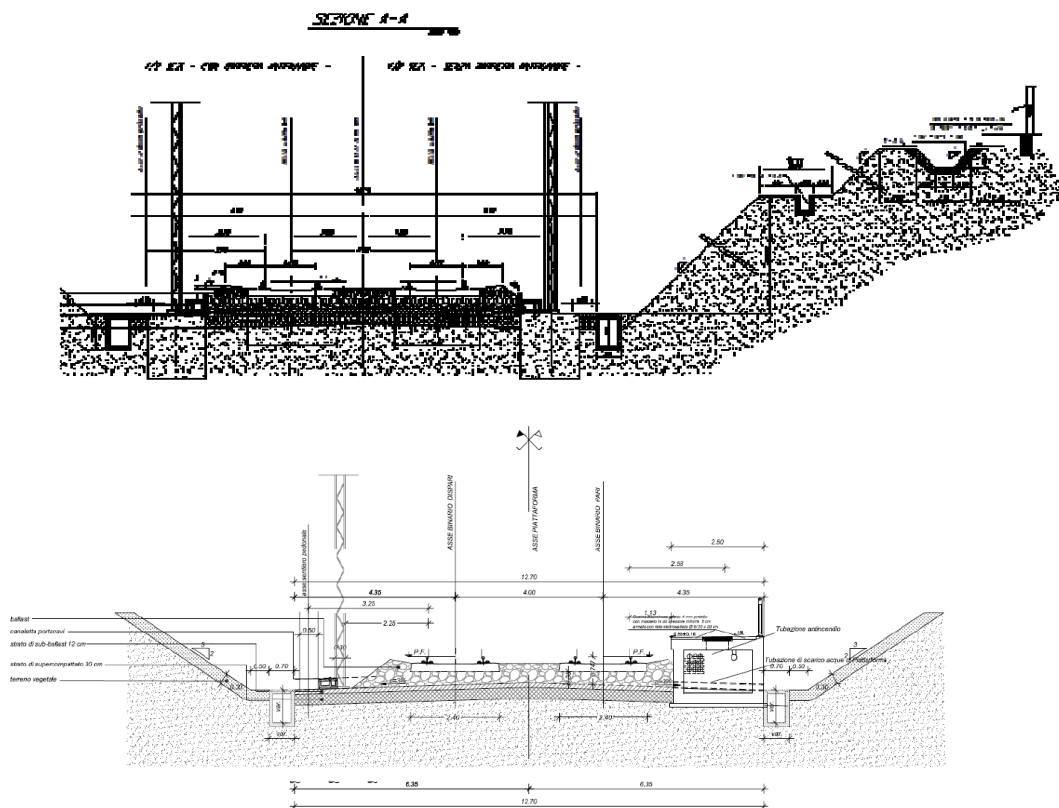
Figura 12 Sezione Tipo in Trincea con Marciapiede FFP/galleria equivalente
