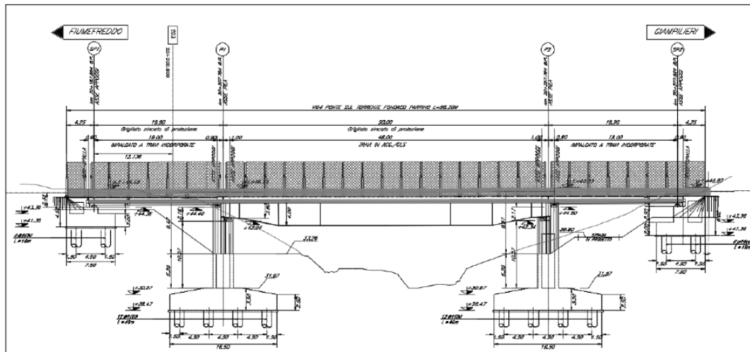
PROSPETTO BINARIO PARI Scala 1:200
