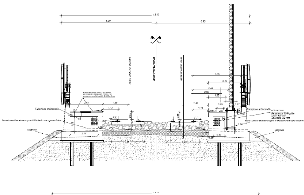
Figura 10 Sezione Tipo in Rilevato con marciapiedi FFP/galleria equivalente e Barriere Antirumore
