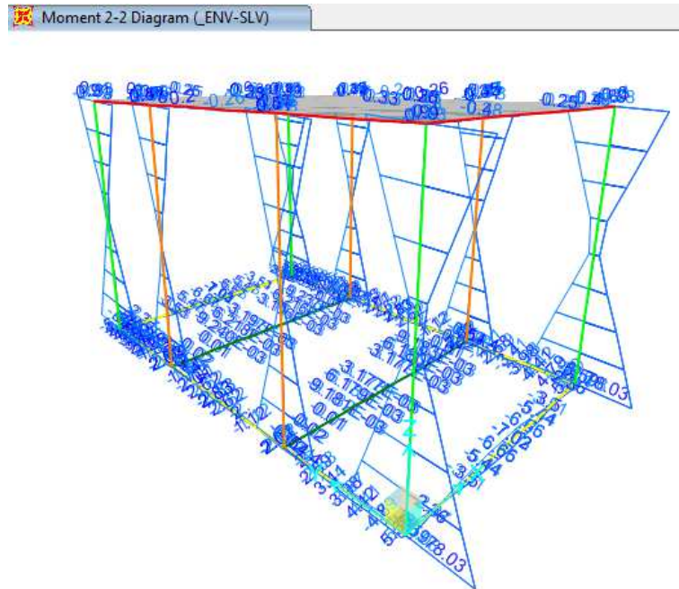
Figura 9-1. Inviluppo SLV – Momento flettente M2
