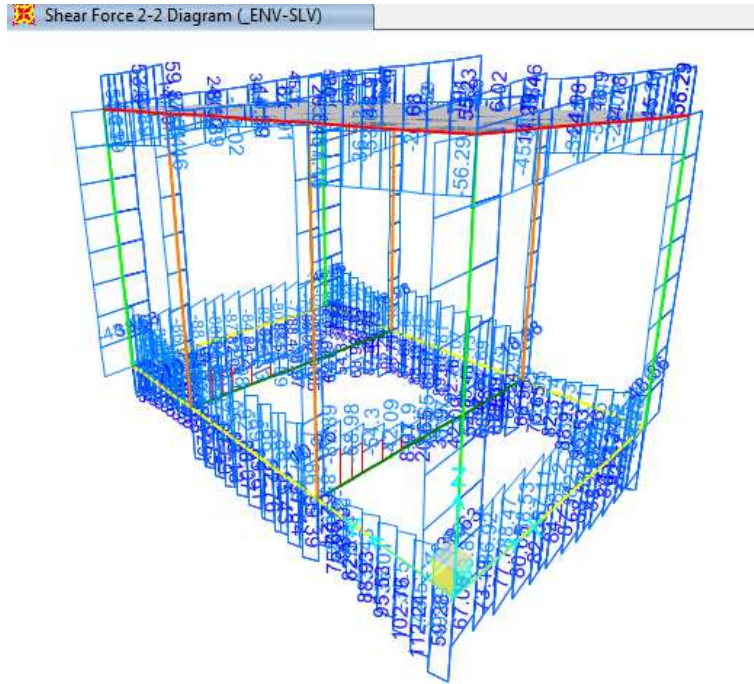
Figura 9-1. Involuppo SLV – Taglio V2
