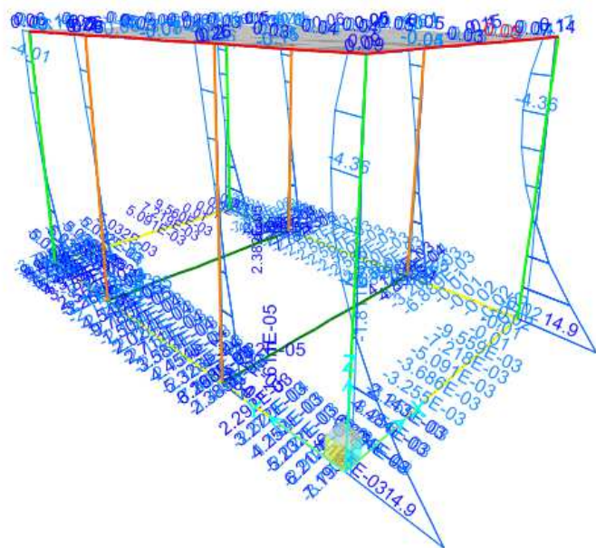
Figura 9-1. Involuppo SLU – Momento flettente M2
