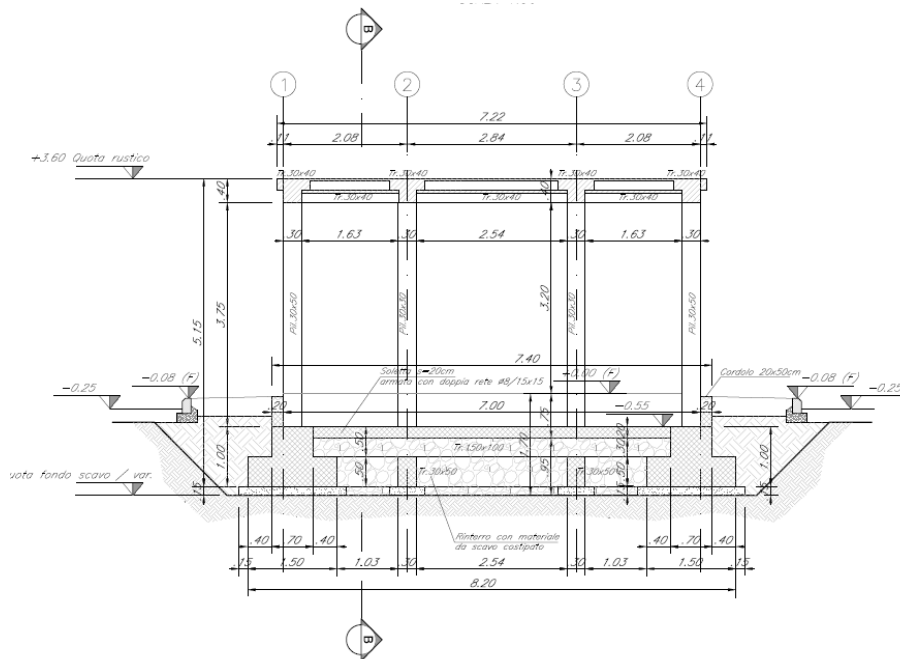
Figura 1-3. Sezione A
