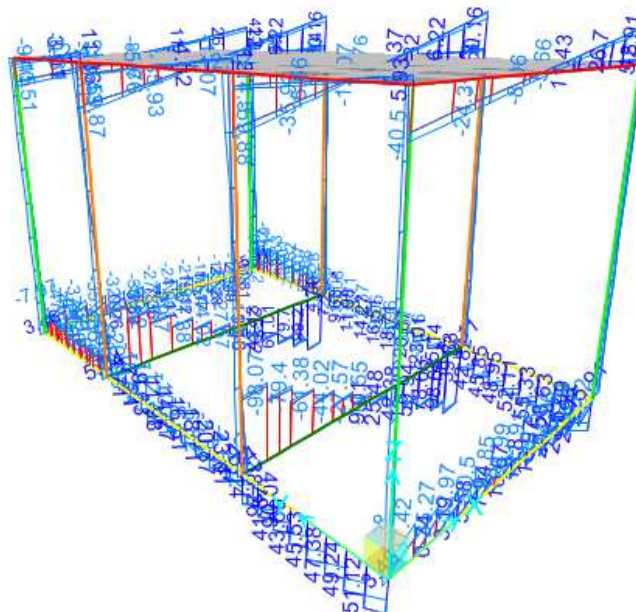
Figura 9-1. Involuppo SLU – Taglio V2
