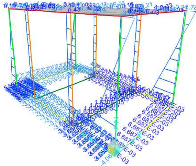
Figura 9-1. Involuppo SLU – Taglio V3
