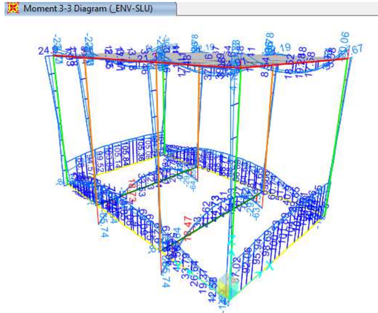
Figura 9-1. Inviluppo SLU – Momento flettente M3
