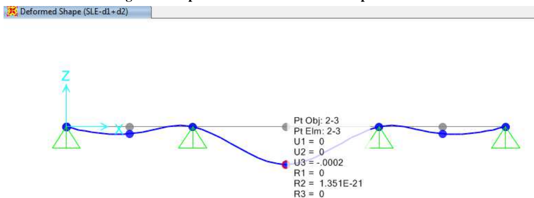
Figura 9-1. Spostamento elastico dovuto ai permanenti
