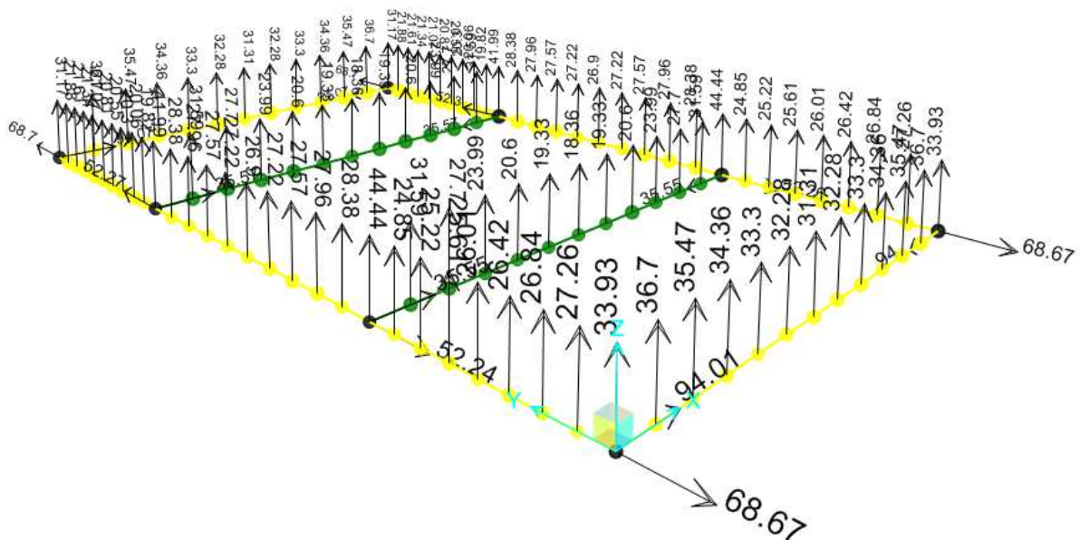
Figura 1-2. Pressioni agenti SLV [KN/m]
