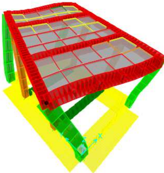
Figura 7-4 Terzo modo di vibrazione (Torsionale)
