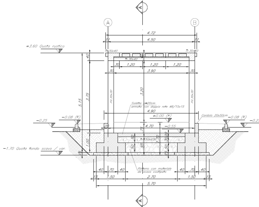
Figura 1-4. Sezione B
