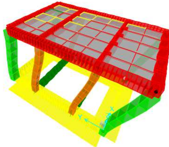
Figura 7-2 Primo modo di vibrazione (Traslazionale in Y)
