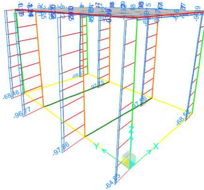
Figura 9-1. Involuppo SLU – Sforzo Normale
