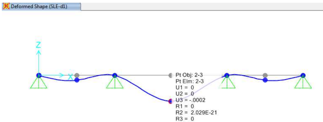
Figura 9-1. Spostamento elastico dovuto ai permanenti
