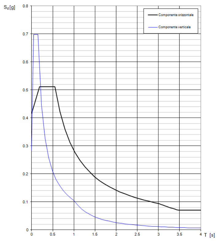
Parametri e punti dello spettro di risposta orizzontale per lo stato SLV Spettri di risposta (componenti orizz. e vert.) per lo stato limite: SLV
