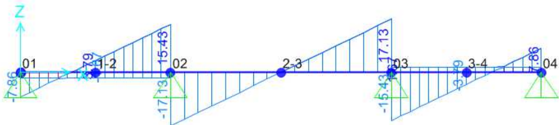
Figura 9-1. Diagramma del taglio
