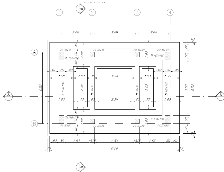
Figura 1-1. Carpenteria fondazioni.
