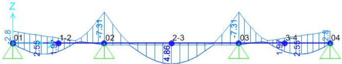
Figura 9-1. Diagramma del momento
