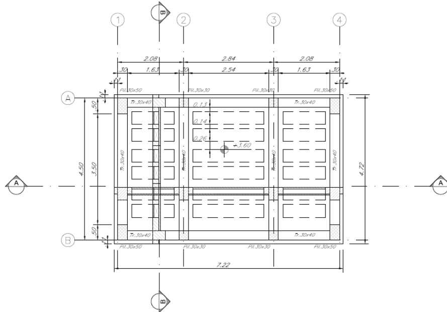
Figura 1-2. Carpenteria copertura.
