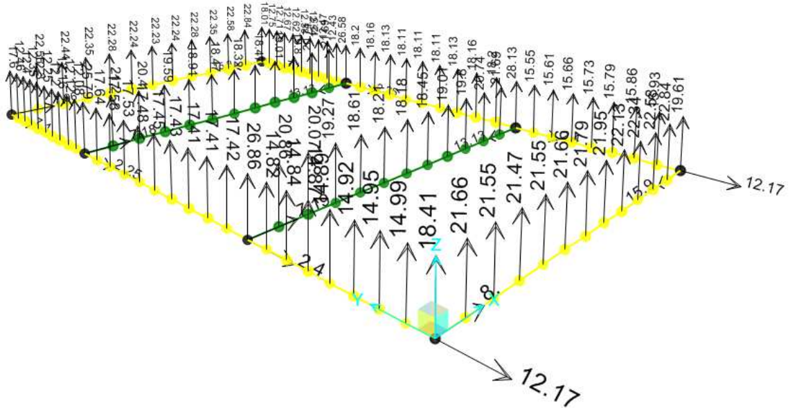
Figura 1-1. Pressioni agenti SLU [KN/m]
