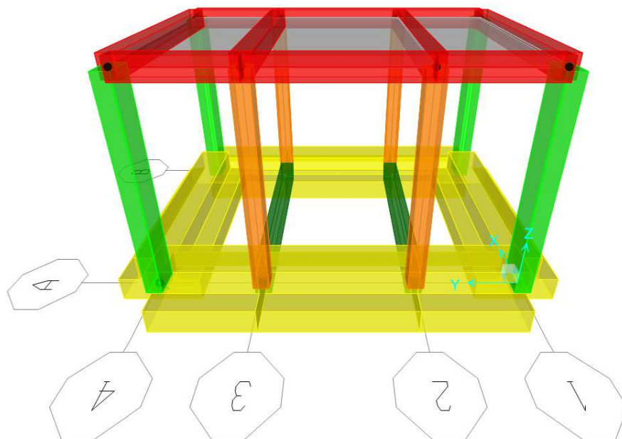
Figura 1-1. Vista estrusa del modello 3D
