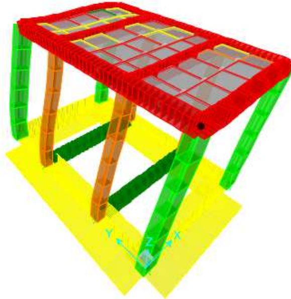
Figura 7-3 Secondo modo di vibrazione (Traslazionale in X)
