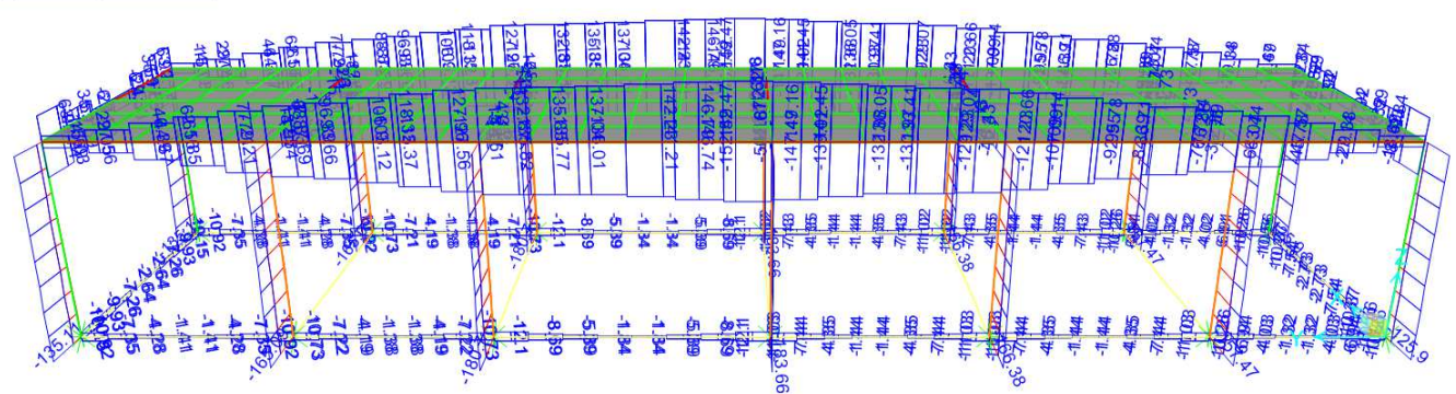
Axial Force Diagram (ENV-SLV)
