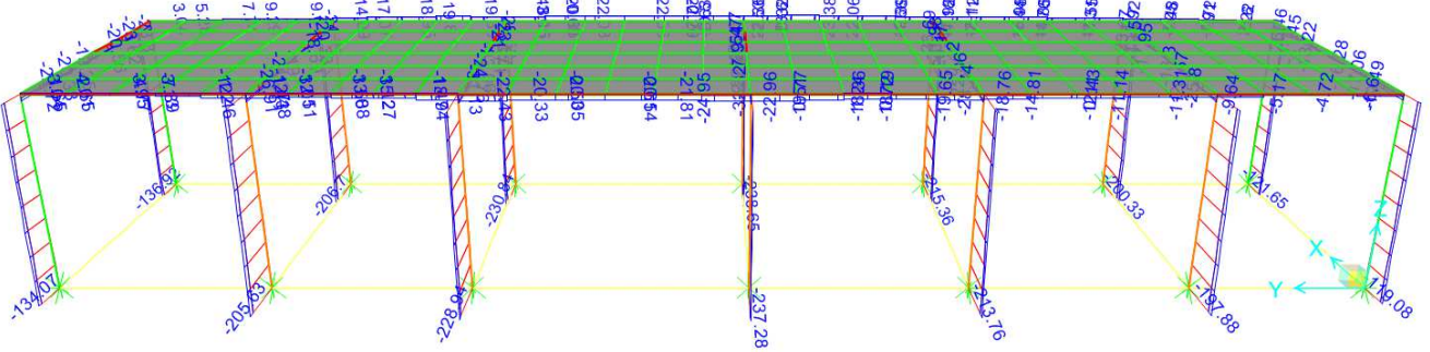
Figura 9-1. Involuppo SLU – Sforzo Normale
