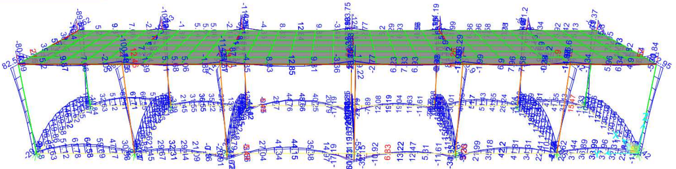
Moment 3-3 Diagram (ENV-SLU)
