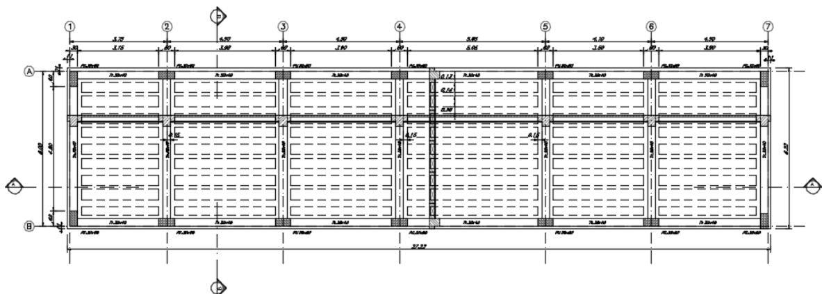
Figura 1-2. Carpenteria copertura.
