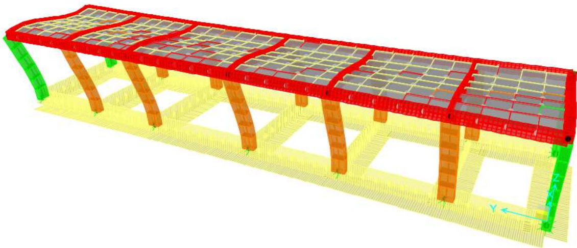
Figura 7-2 Primo modo di vibrazione (Traslazionale in X)
