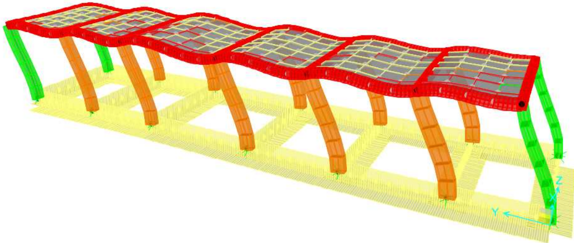
Figura 7-4 Terzo modo di vibrazione (Traslazionale in Y)
