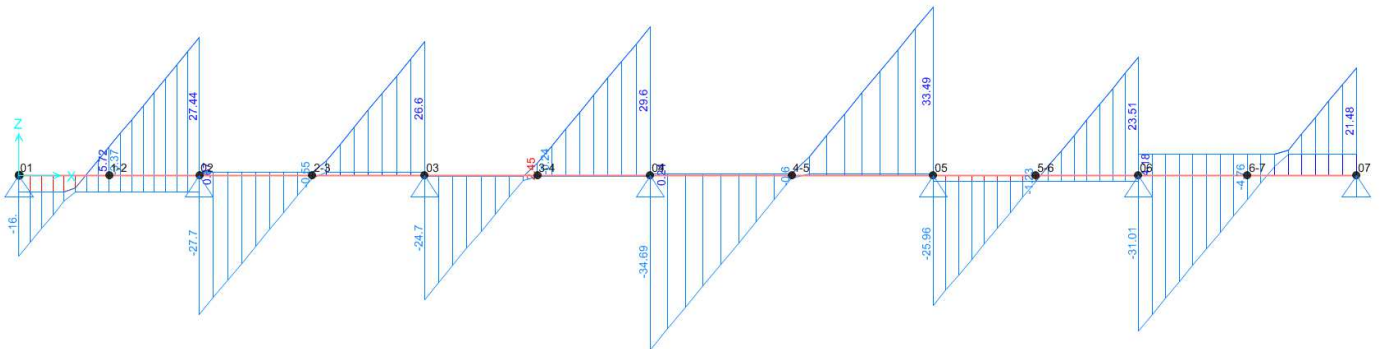
Figura 9-1. Diagramma del taglio
