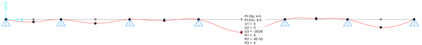
Figura 9-1. Spostamento elastico dovuto ai permanenti
