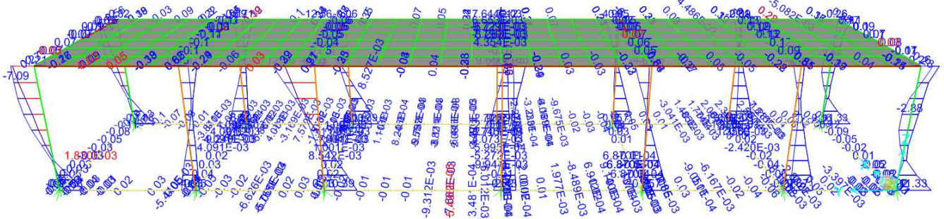
Figura 9-1. Involuppo SLU – Momento flettente M2
