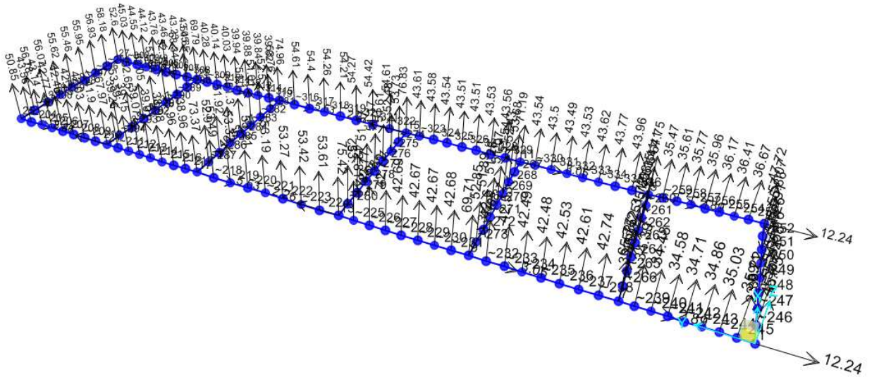
Figura 1-1. Pressioni agenti SLU [KN/m]
