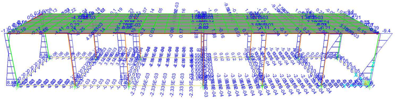
Figura 9-1. Involuppo SLU – Taglio V3
