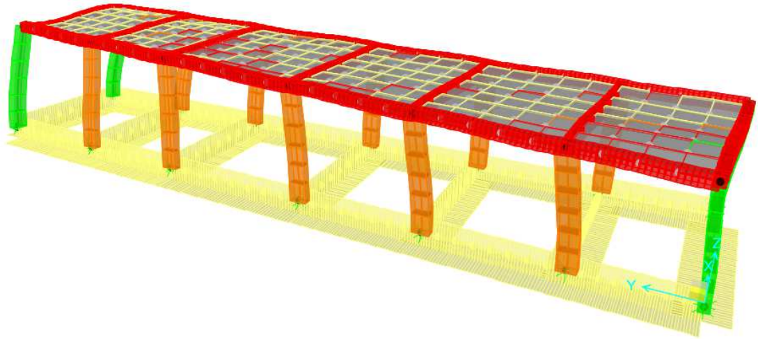
Figura 7-3 Secondo modo di vibrazione (Torsionale)
