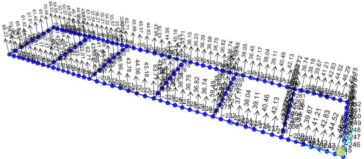
Figura 1-3. Pressioni agenti SLV_y [kN/m]
