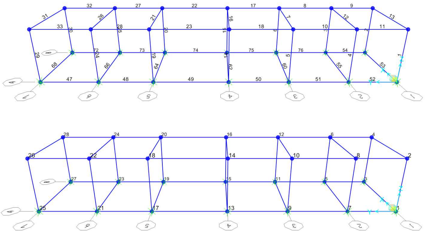
Figura 7-1 Modello di calcolo – Numerazione aste e nodi
