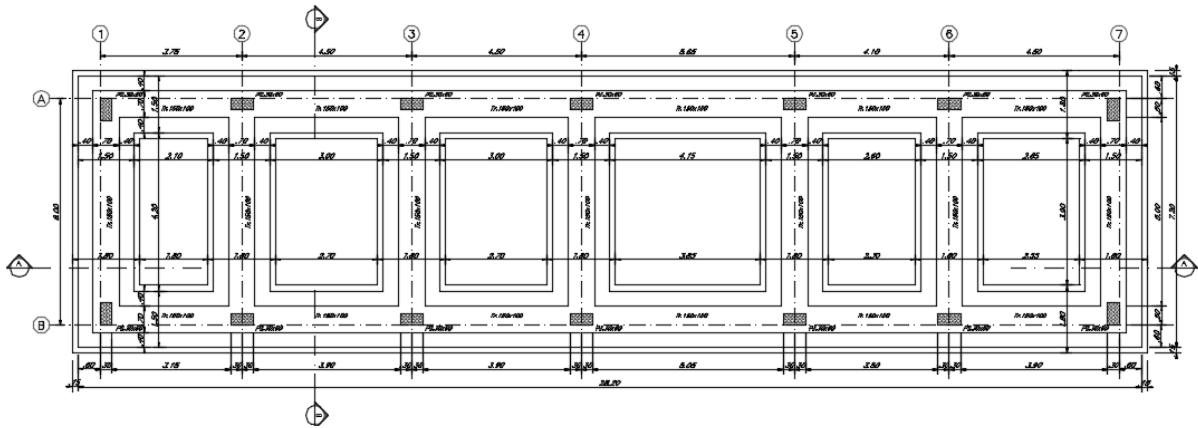
Figura 1-1. Carpenteria fondazioni.
