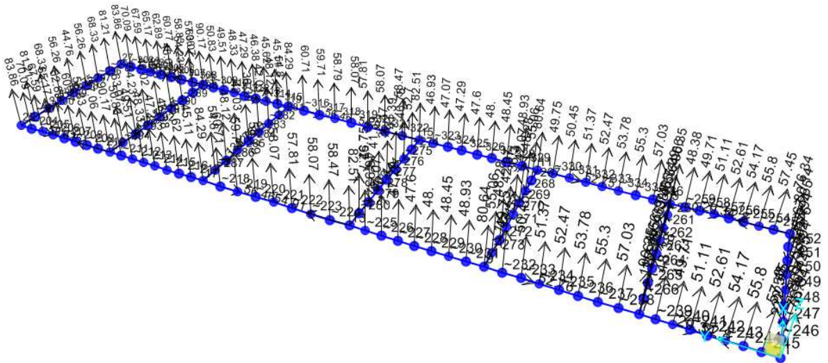
Figura 1-2. Pressioni agenti SLV_x [KN/m]
