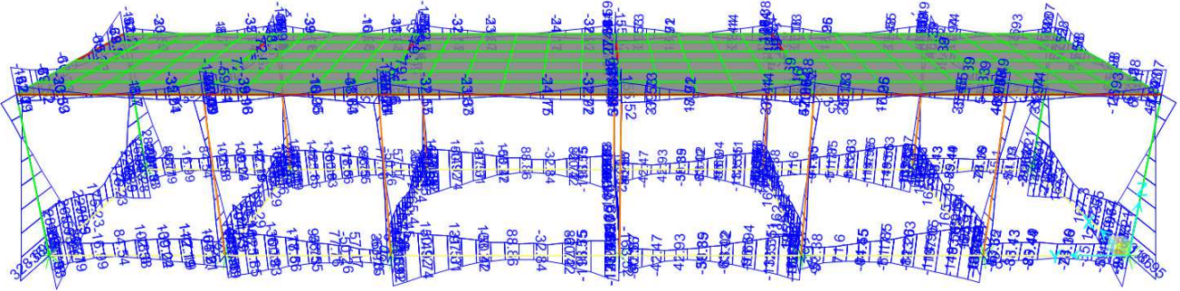
Figura 9-1. Involuppo SLV – Momento flettente M3
