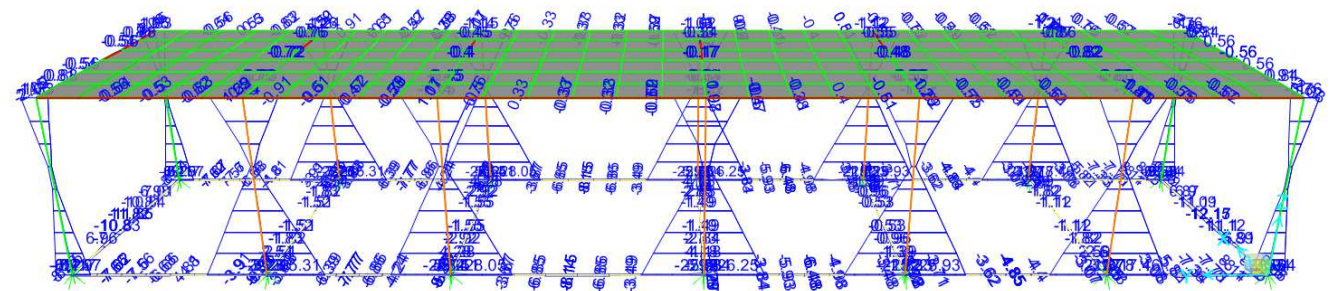
Figura 9-1. Involuppo SLV – Momento flettente M2
