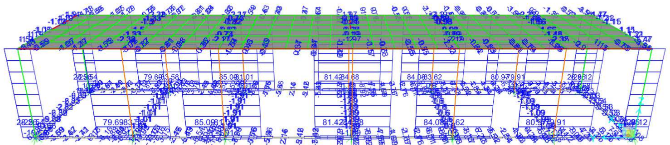
Figura 9-1. Involuppo SLV – Taglio V3
