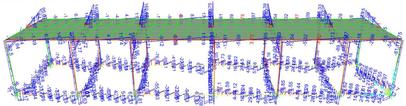
Shear Force 2-2 Diagram (ENV-SLU)
