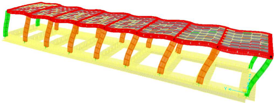
Figura 7-4 Terzo modo di vibrazione (Traslazionale in Y)
