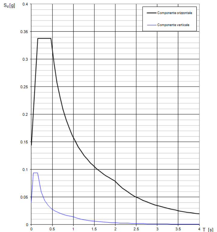
Parametri e punti dello spettro di risposta orizzontale per lo stato limBLO Spettri di risposta (componenti orizz. e vert.) per lo stato limite: SLO
