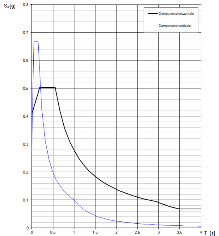
Parametri e punti dello spettro di risposta orizzontale per lo stato limite SLV Spettri di risposta (componenti orizz. e vert.) per lo stato limite: SLV
