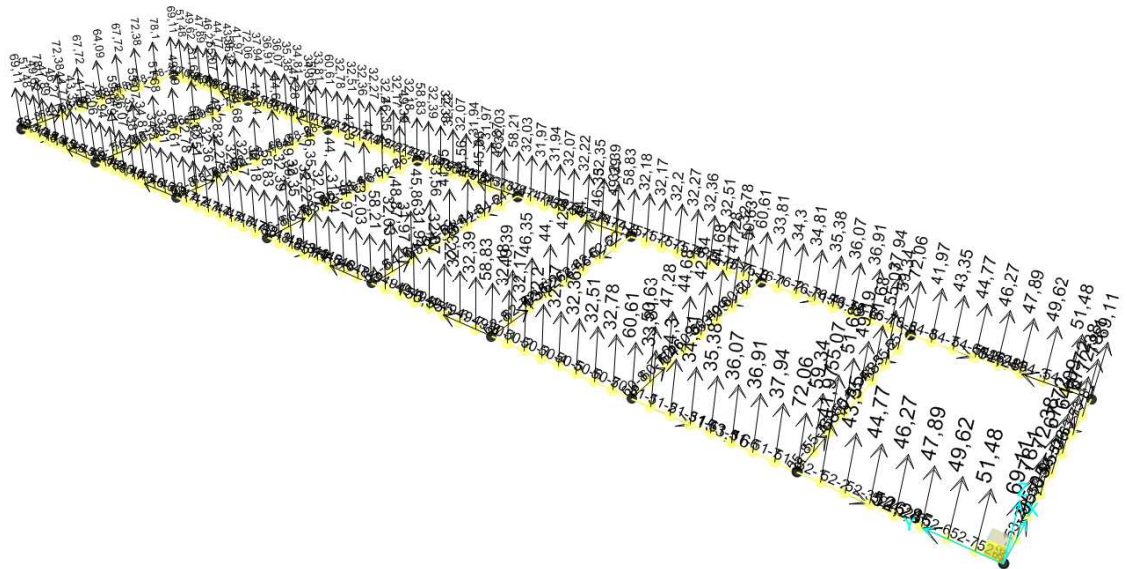
Figura 1-3. Pressioni agenti SLV_y [kN/m]
