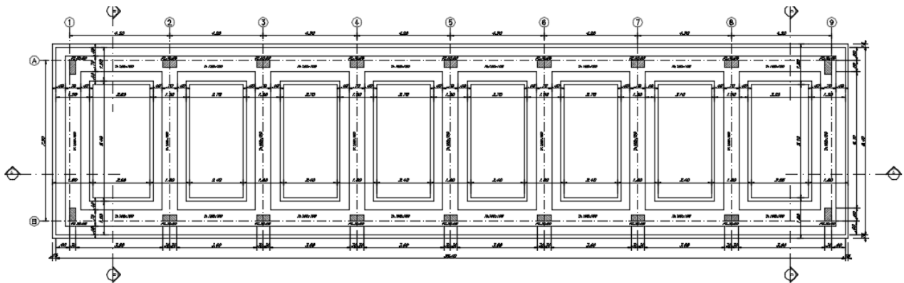
Figura 1-1. Carpenteria fondazioni.
