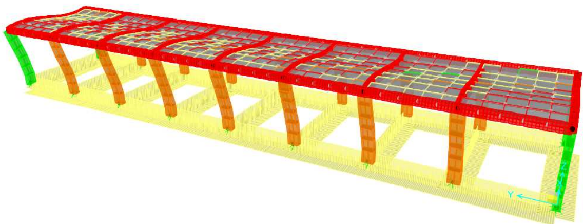
Figura 7-2 Primo modo di vibrazione (Traslazionale in X)
