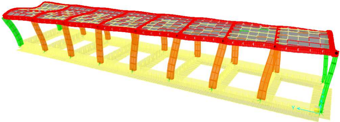
Figura 7-3 Secondo modo di vibrazione (Torsionale)
