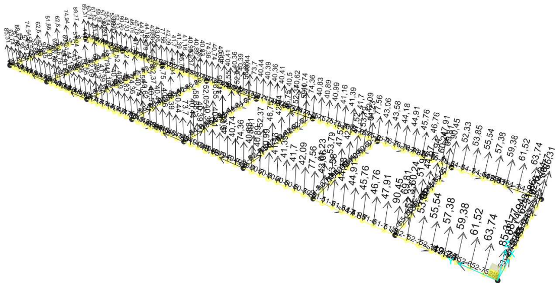
Figura 1-2. Pressioni agenti SLV_x [kN/m]
