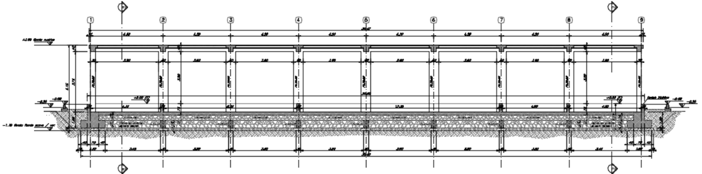
Figura 1-3. Sezione A
