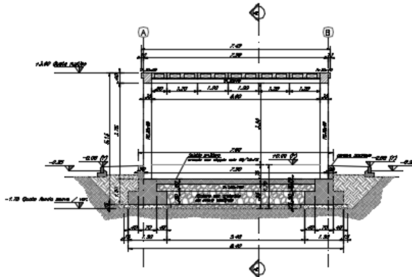
Figura 1-4. Sezione B
