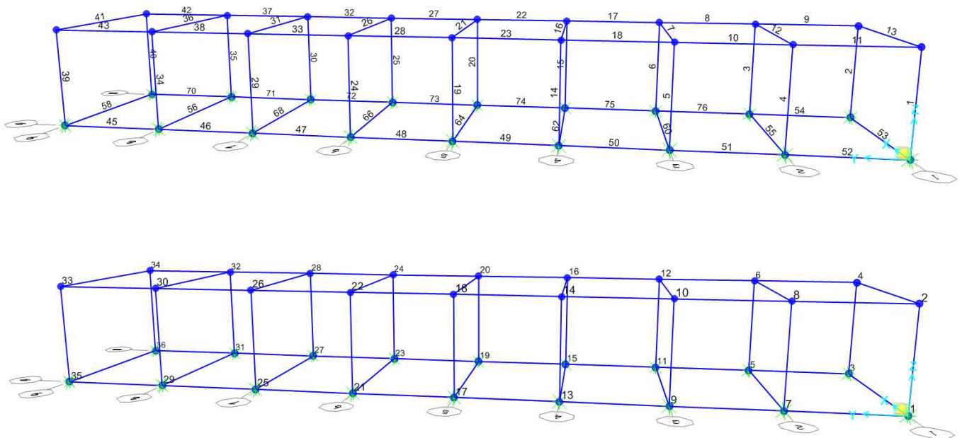
Figura 7-1 Modello di calcolo – Numerazione aste e nodi
