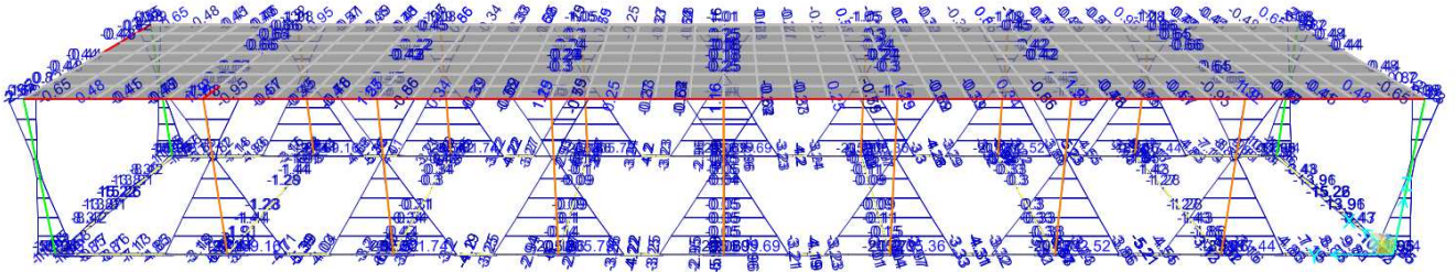
Figura 9-1. Involuppo SLV – Momento flettente M2
