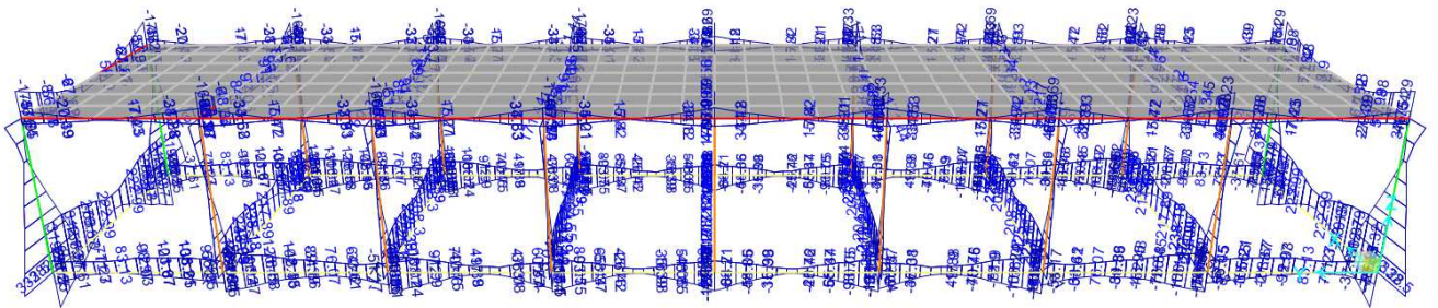
Figura 9-1. Involuppo SLV – Momento flettente M3
