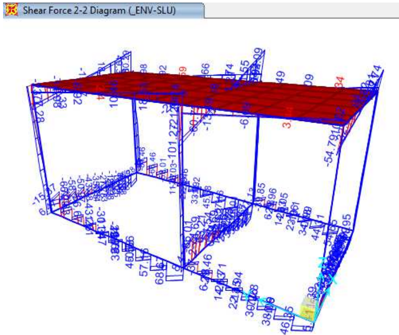
Figura 9-1. Involuppo SLU – Taglio V2
