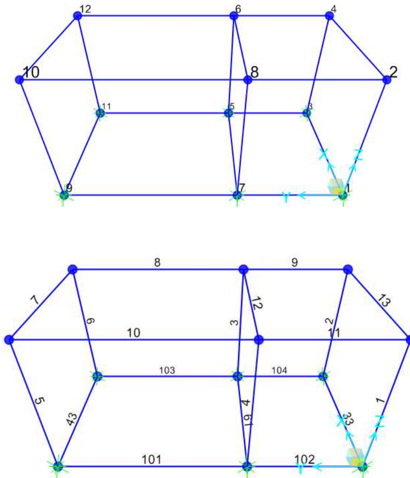
Figura 7-1 Modello di calcolo – Numerazione aste e nodi
