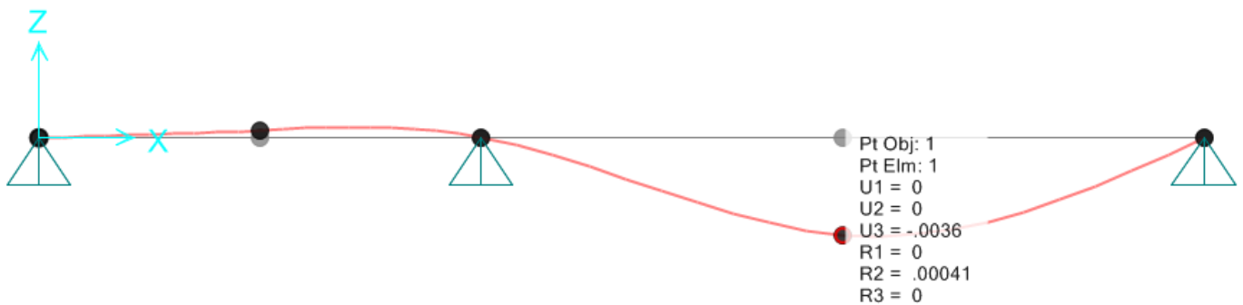
Figura 9-1. Spostamento elastico dovuto ai permanenti
