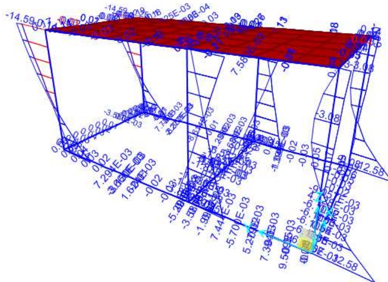
Figura 9-1. Involuppo SLU – Momento flettente M2
