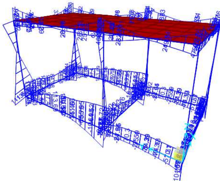
Figura 9-1. Involuppo SLV – Momento flettente M3
