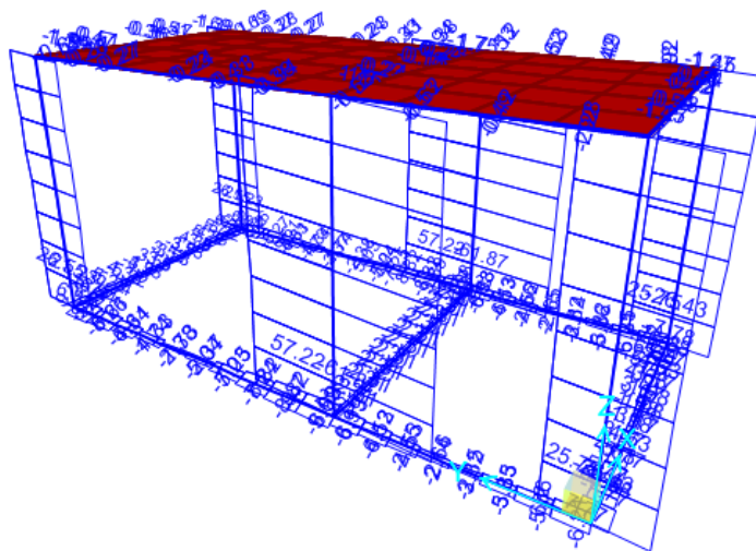
Figura 9-1. Involuppo SLV – Taglio V3
