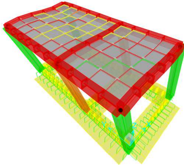
Figura 7-2 Primo modo di vibrazione (Traslazionale in X)
