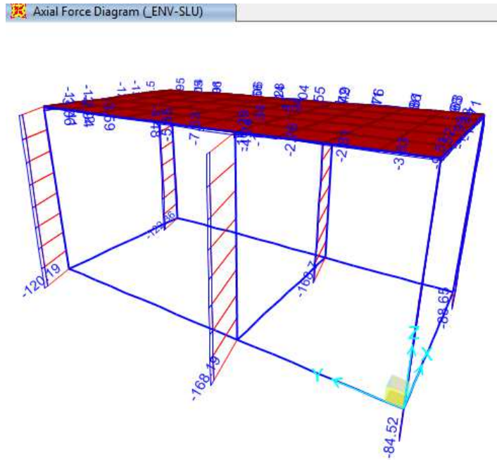
Figura 9-1. Involuppo SLU – Sforzo Normale
