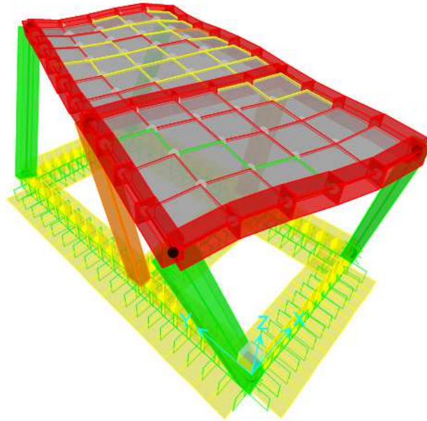
Figura 7-4 Terzo modo di vibrazione (Torsionale)
