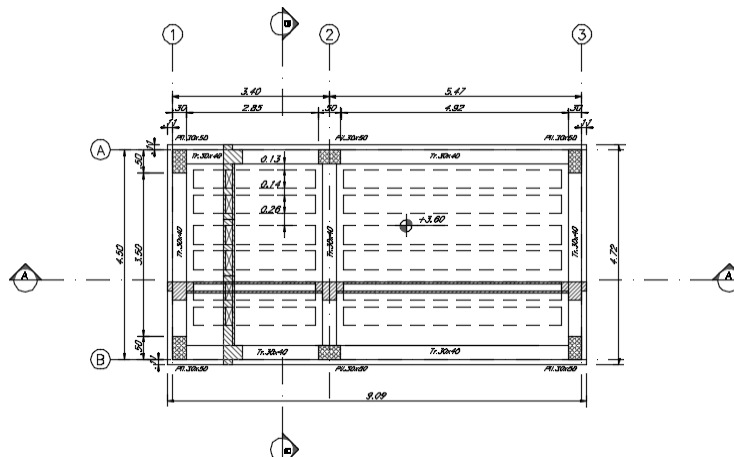
Figura 1-2. Carpenteria copertura.
