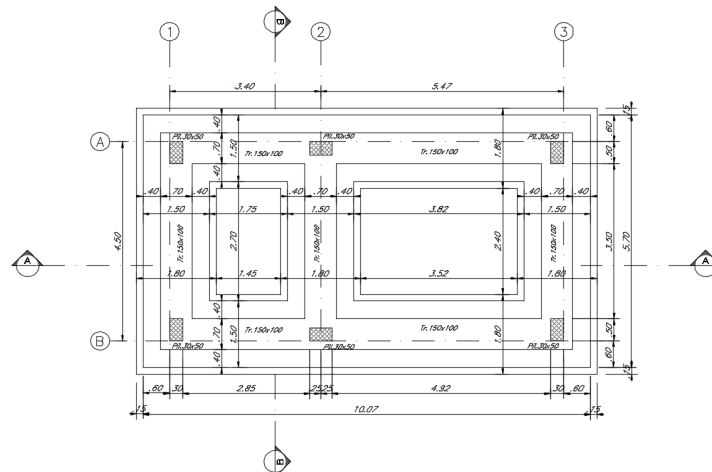
Figura 1-1. Carpenteria fondazioni.
