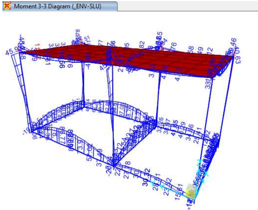
Figura 9-1. Involuppo SLU – Momento flettente M3
