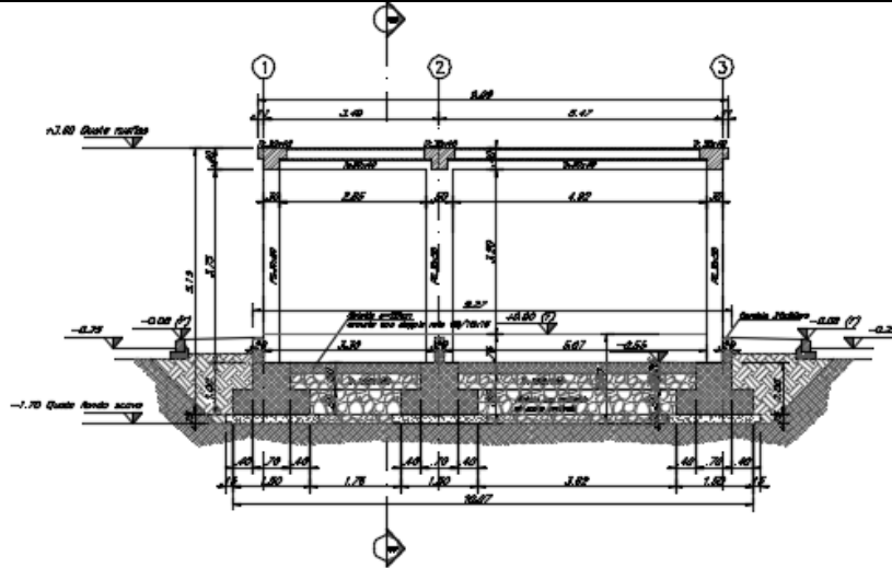
Figura 1-3. Sezione A
