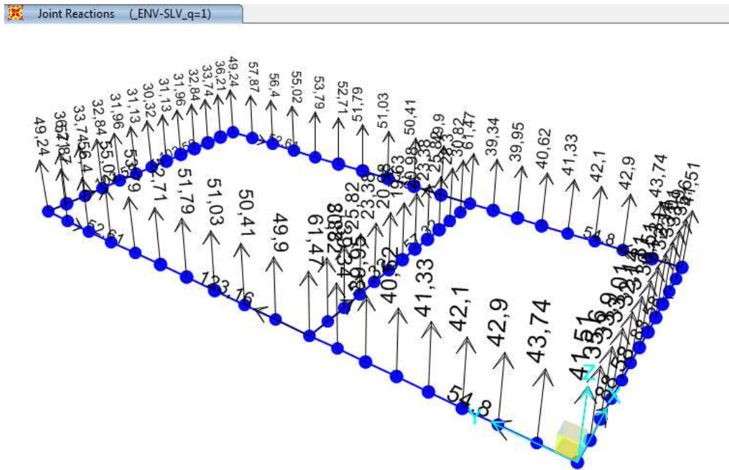
Figura 1-2. Pressioni agenti SLV [KN/m]
