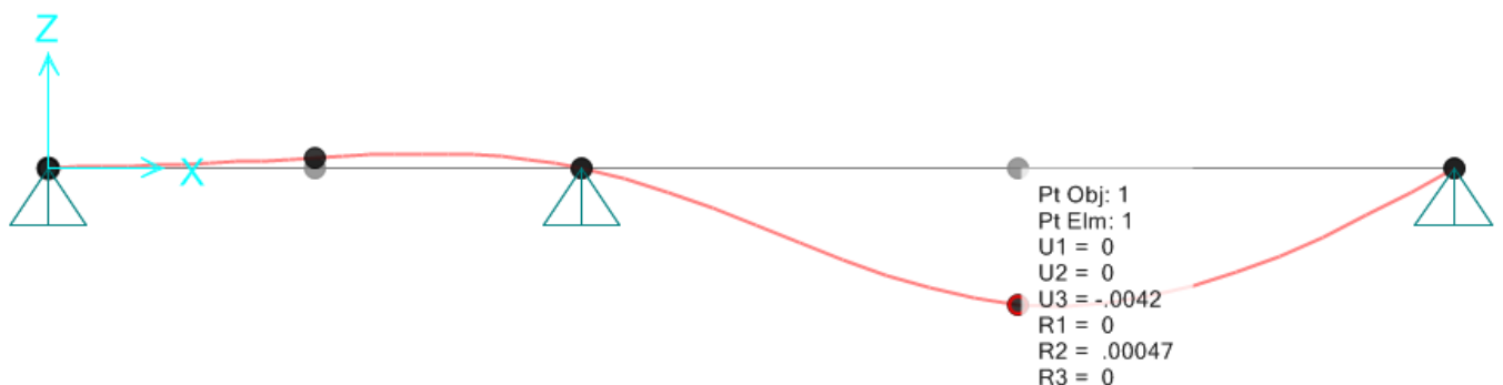
Figura 9-1. Spostamento elastico dovuto ai permanenti + variabili
