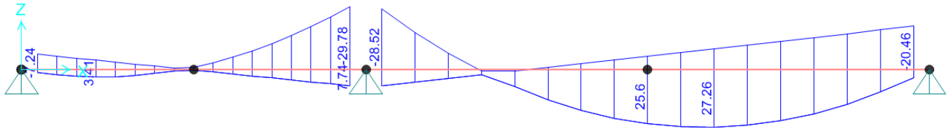
Figura 9-1. Diagramma del momento
