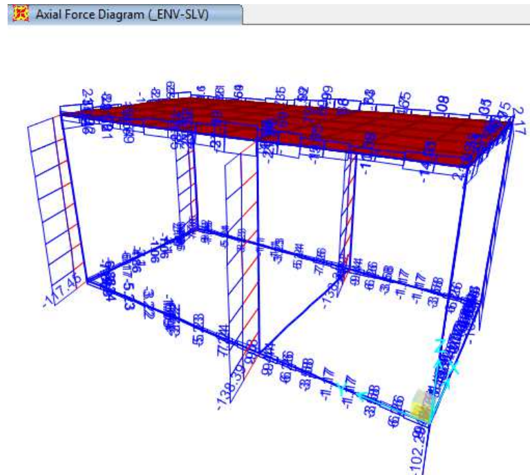
Figura 9-1. Involuppo SLV – Sforzo Normale
