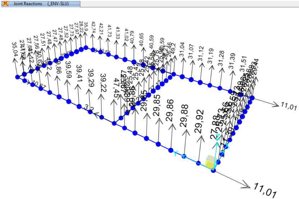
Figura 1-1. Pressioni agenti SLU [KN/m]
