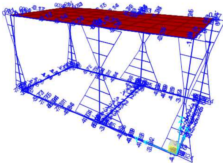
Figura 9-1. Involuppo SLV – Momento flettente M2
