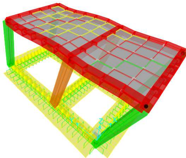
Figura 7-3 Secondo modo di vibrazione (Traslazionale in Y)
