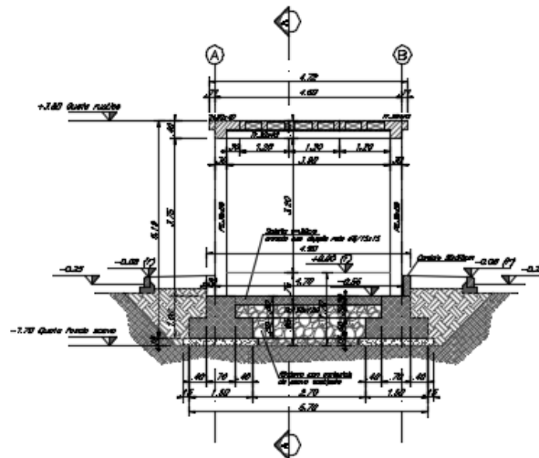
Figura 1-4. Sezione B
