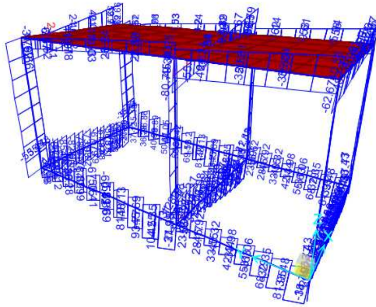
Figura 9-1. Involuppo SLV – Taglio V2
