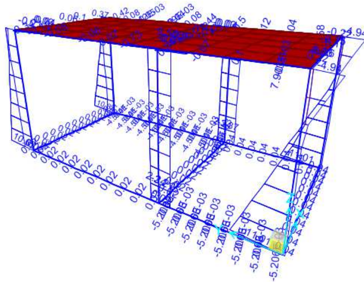
Figura 9-1. Involuppo SLU – Taglio V3
