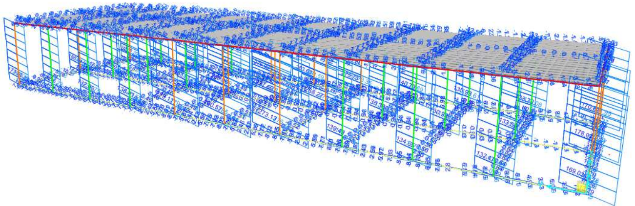
Figura 9-1. Involuppo SLV – Taglio V3
