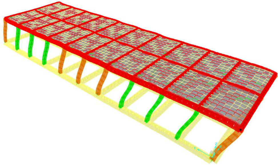
Figura 7-3 Secondo modo di vibrazione (Traslazionale in Y)
