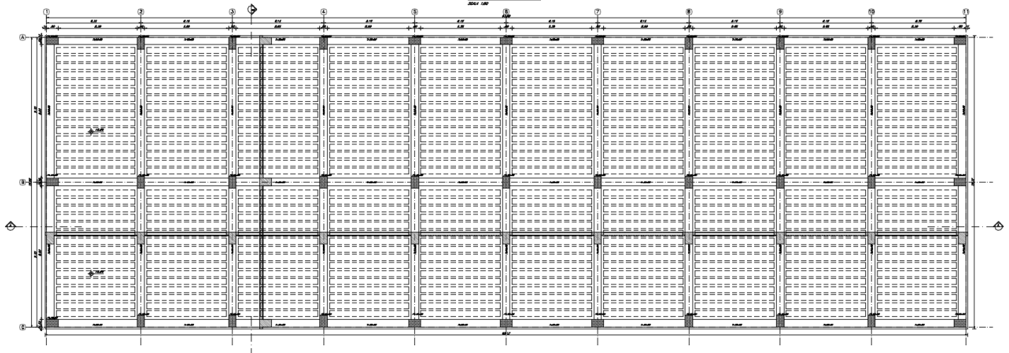
Figura 1-2. Carpenteria copertura.
