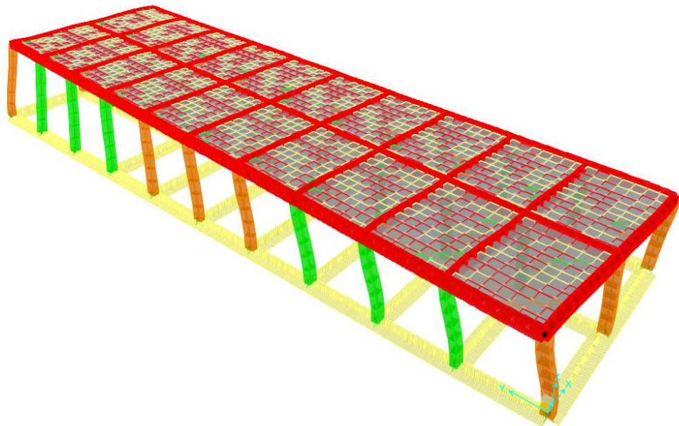
Figura 7-4 Terzo modo di vibrazione (Torsionale)
