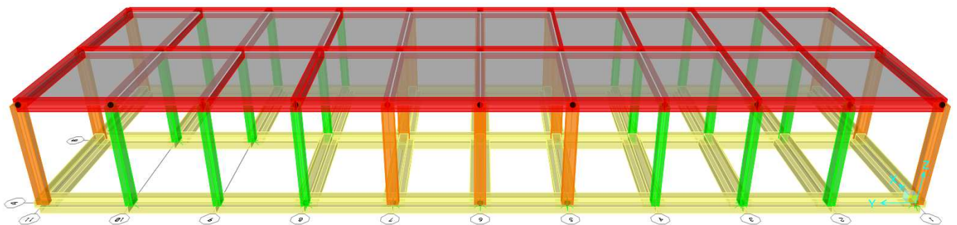
Figura 1-1. Vista estrusa del modello 3D
