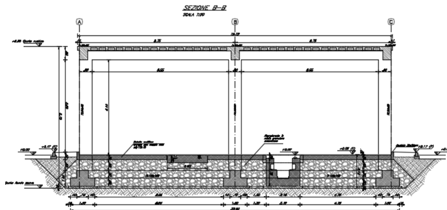
Figura 1-4. Sezione B
