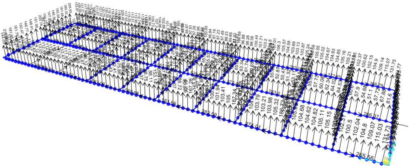
Figura 1-2. Pressioni agenti SLV [kN/m]
