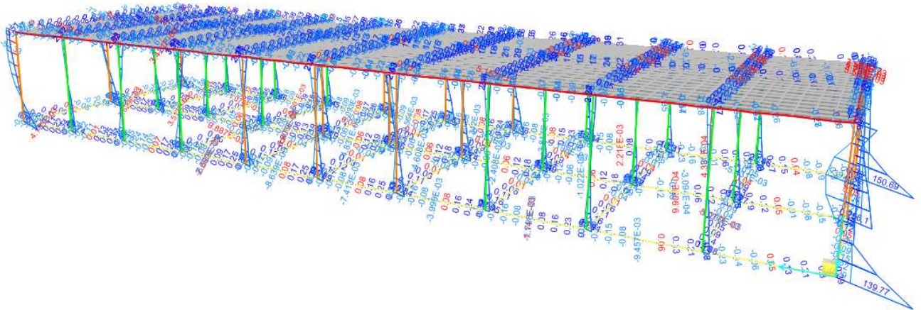
Figura 9-1. Involuppo SLU – Momento flettente M2
