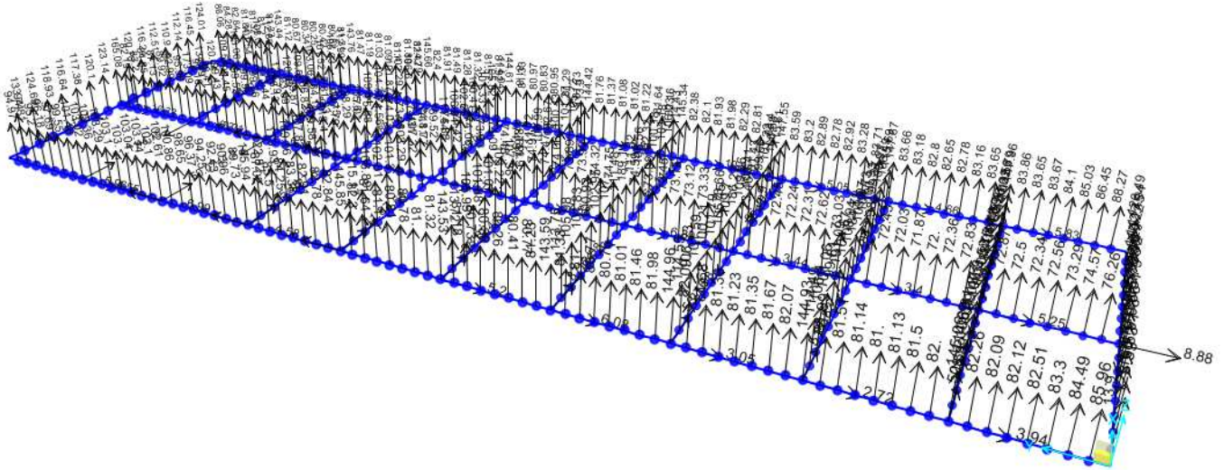
Figura 1-1. Pressioni agenti SLU [kN/m]
