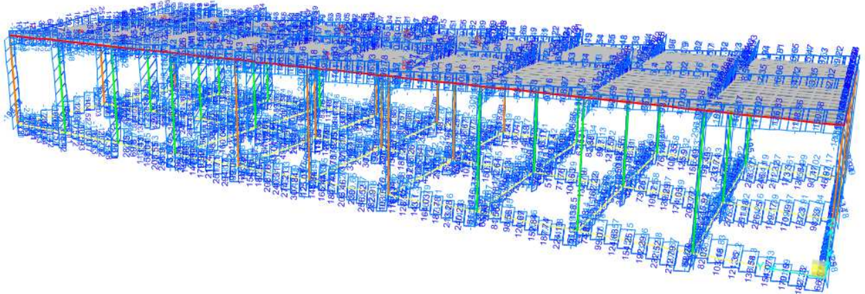
Figura 9-1. Involuppo SLV – Taglio V2
