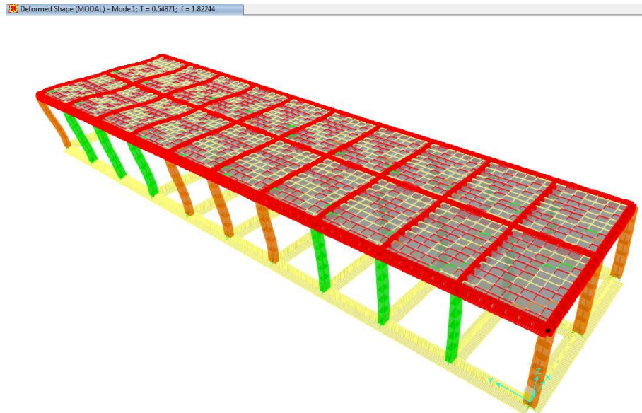
Figura 7-2 Primo modo di vibrazione (Traslazionale in X)
