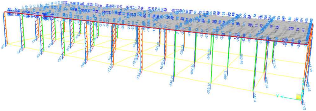
Figura 9-1. Involuppo SLU – Sforzo Normale
