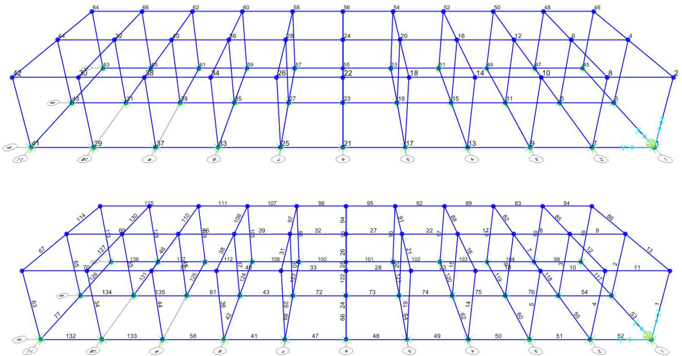
Figura 7-1 Modello di calcolo – Numerazione aste e nodi
