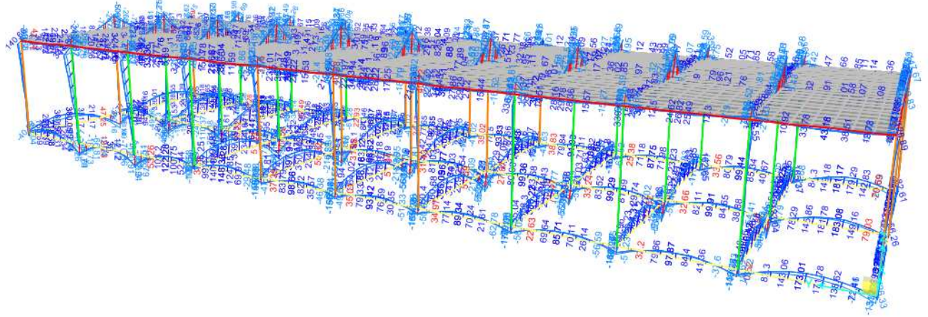
Figura 9-1. Involuppo SLU – Momento flettente M3
