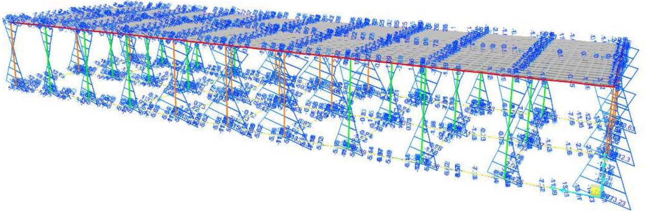
Figura 9-1. Involuppo SLV – Momento flettente M2
