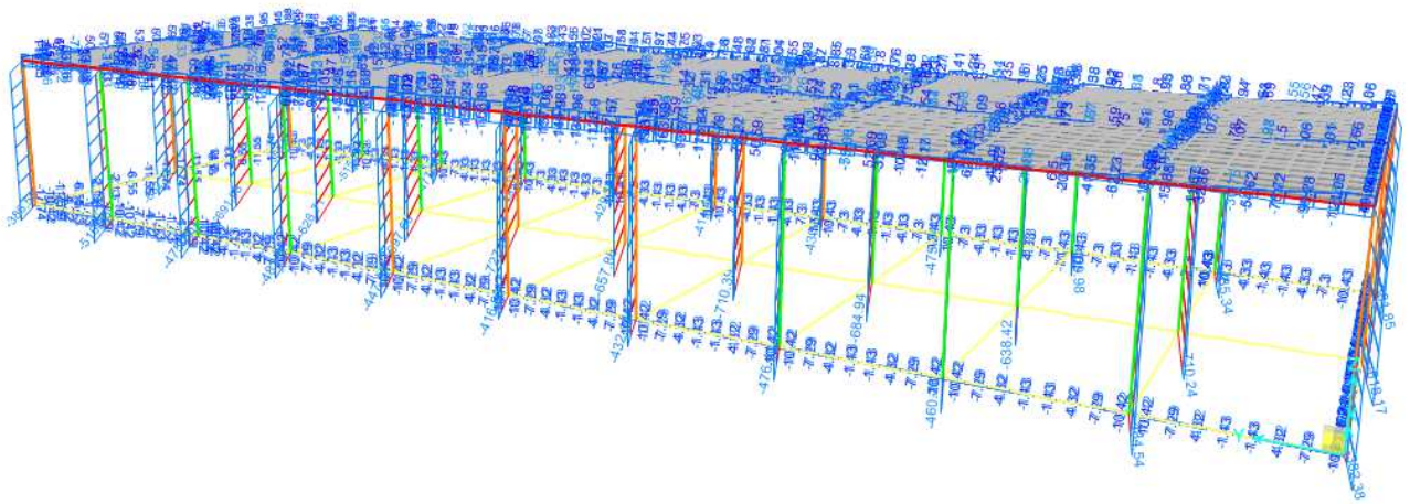
Figura 9-1. Involuppo SLV – Sforzo Normale
