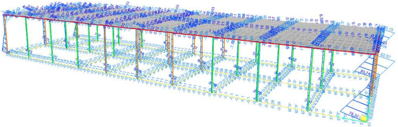
Figura 9-1. Involuppo SLU – Taglio V3
