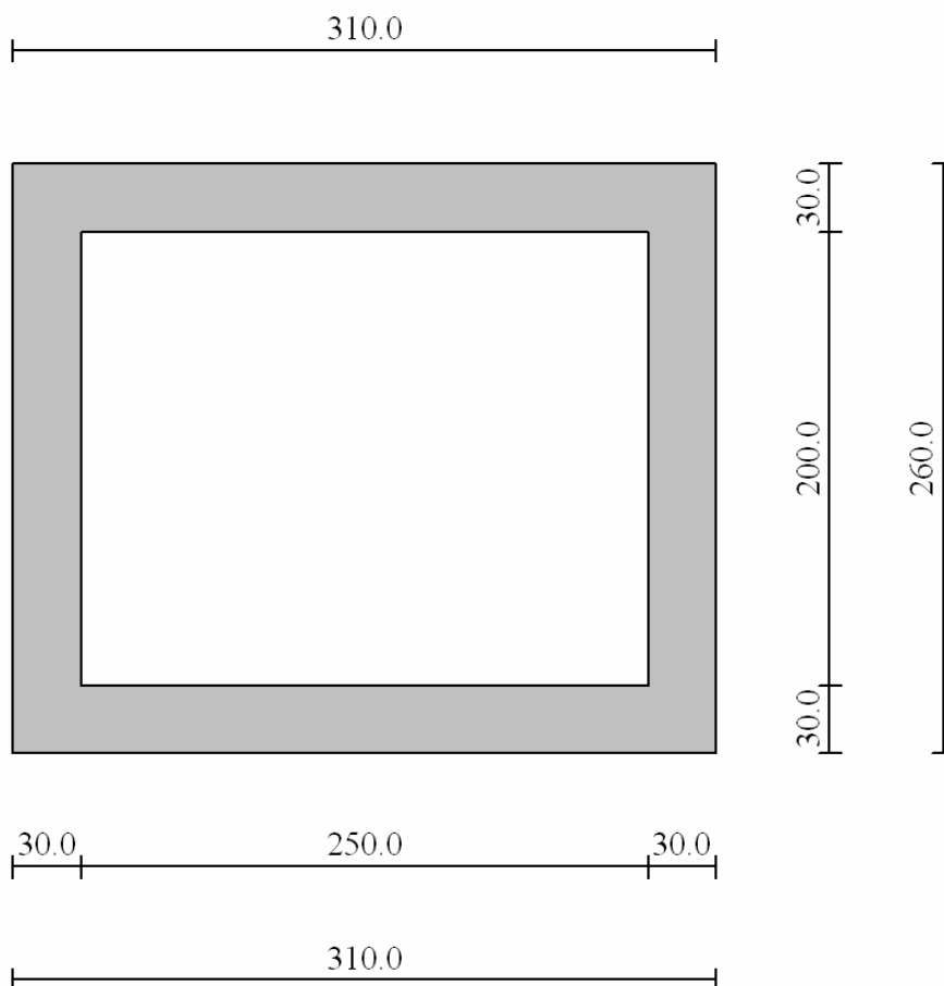
Figura 1.1: Sezione sottovia. Quote espresse in cm.
