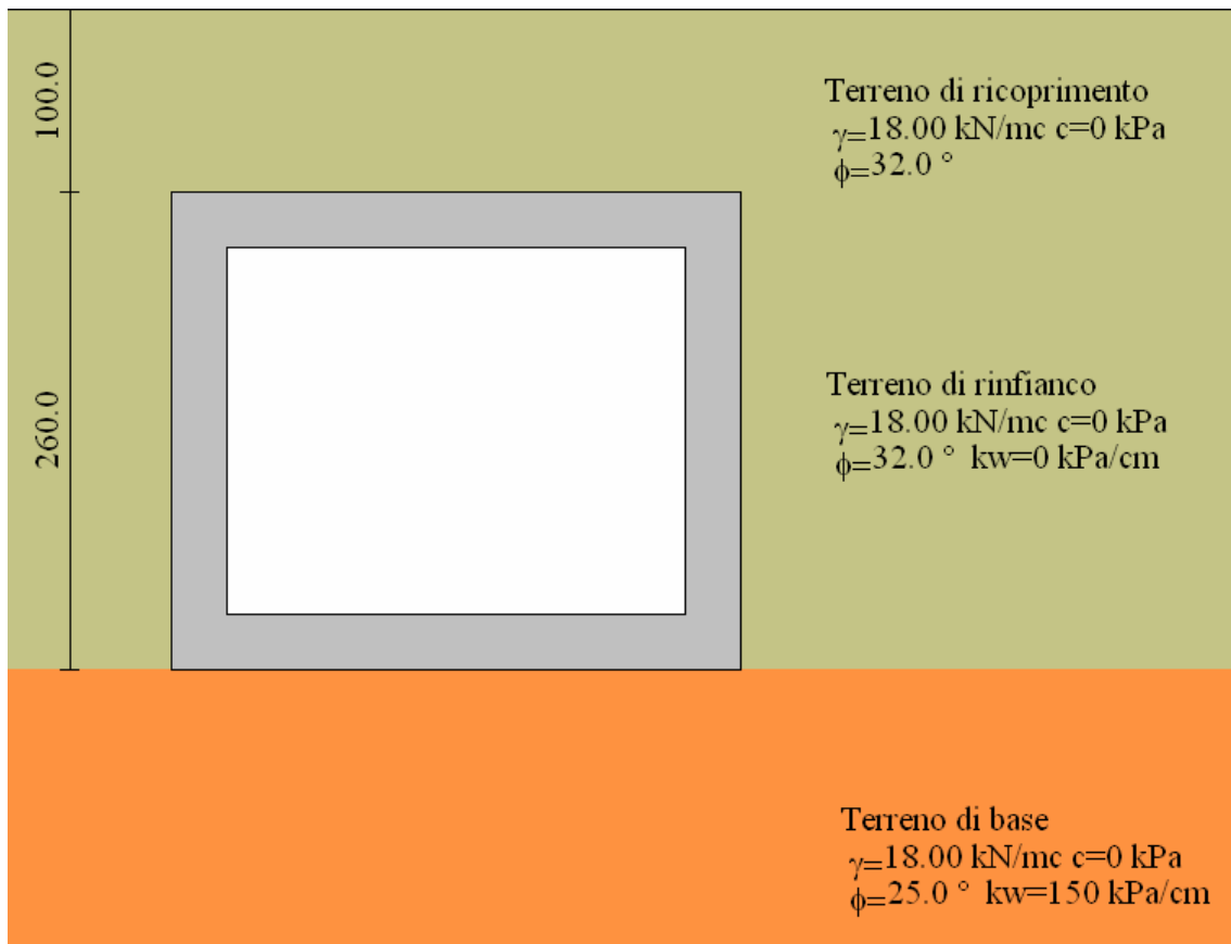
Figura 4.1: Modello geotecnico
