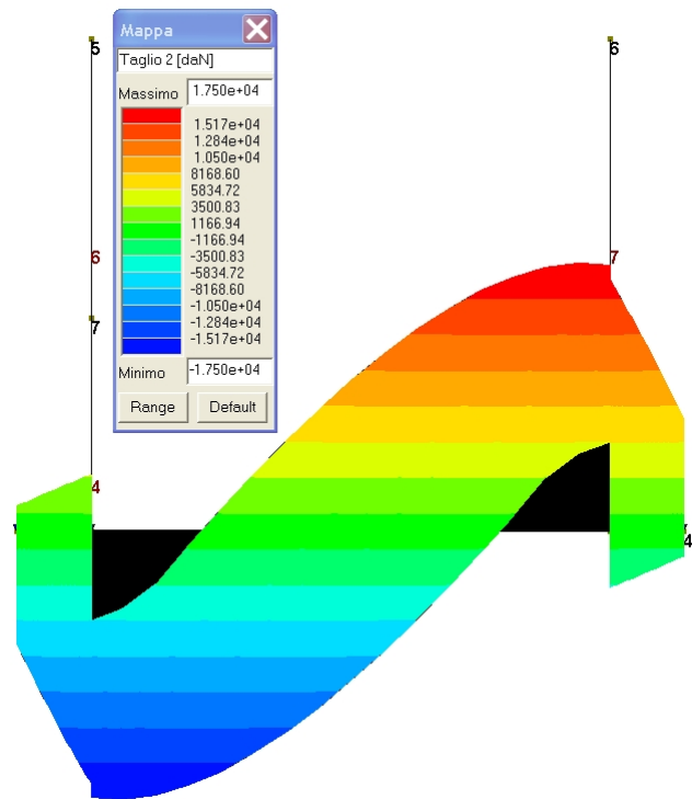
Inviluppo taglio
