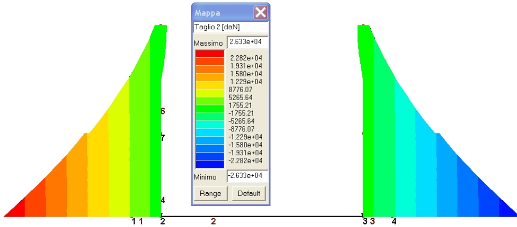
Inviluppo taglio
