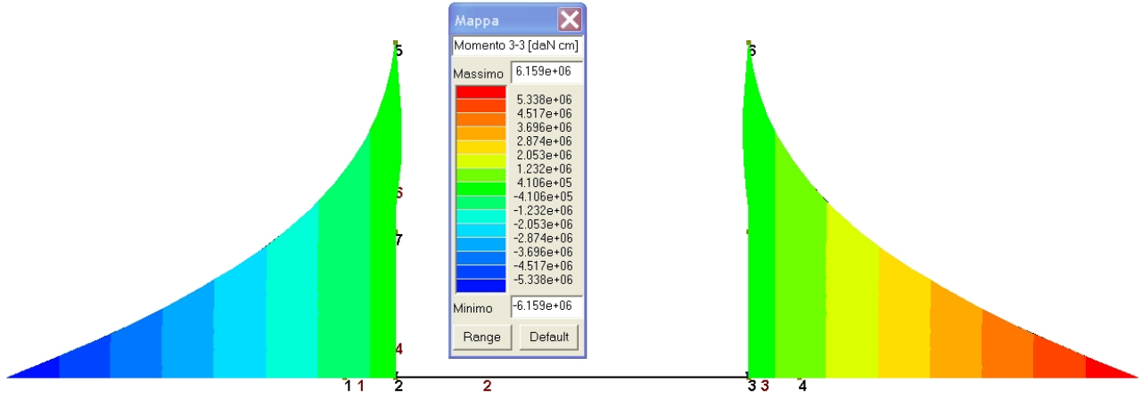
Inviluppo momento
