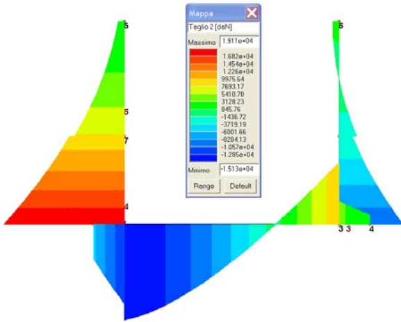
Taglio
