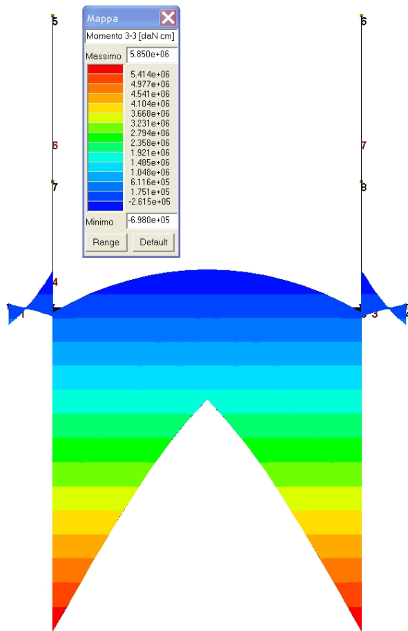
Inviluppo momento
