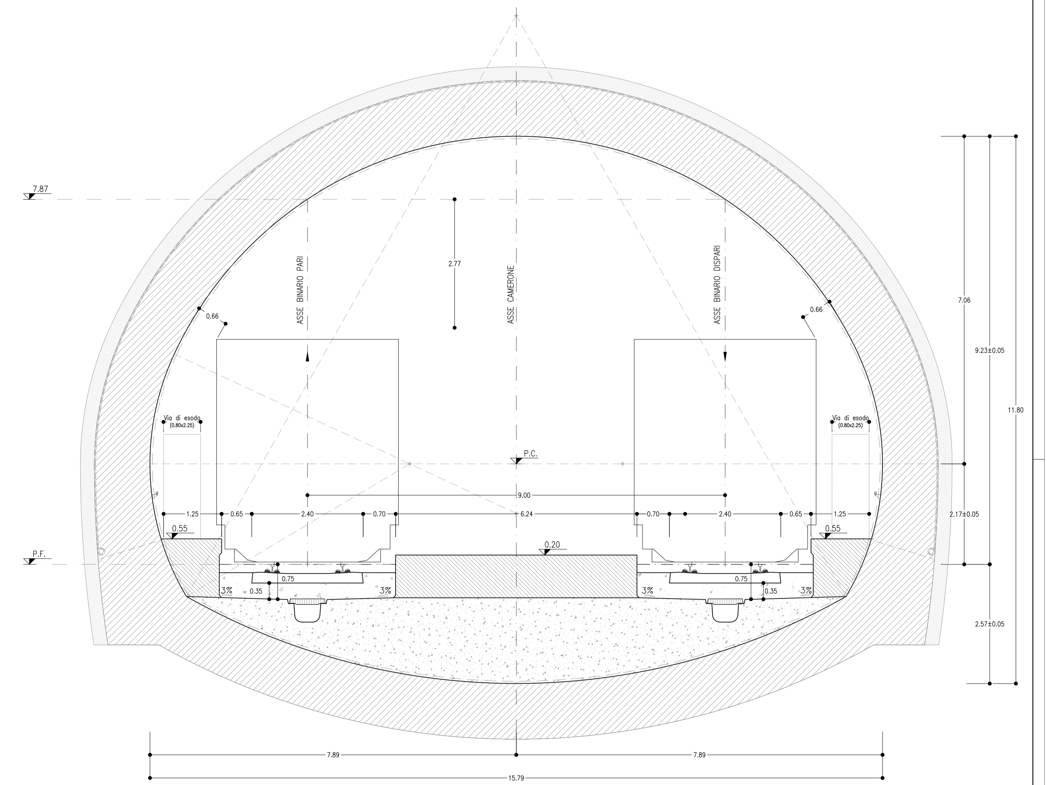
SEZIONE TIPO INTERASSE 7-9 SCALA 1:50
