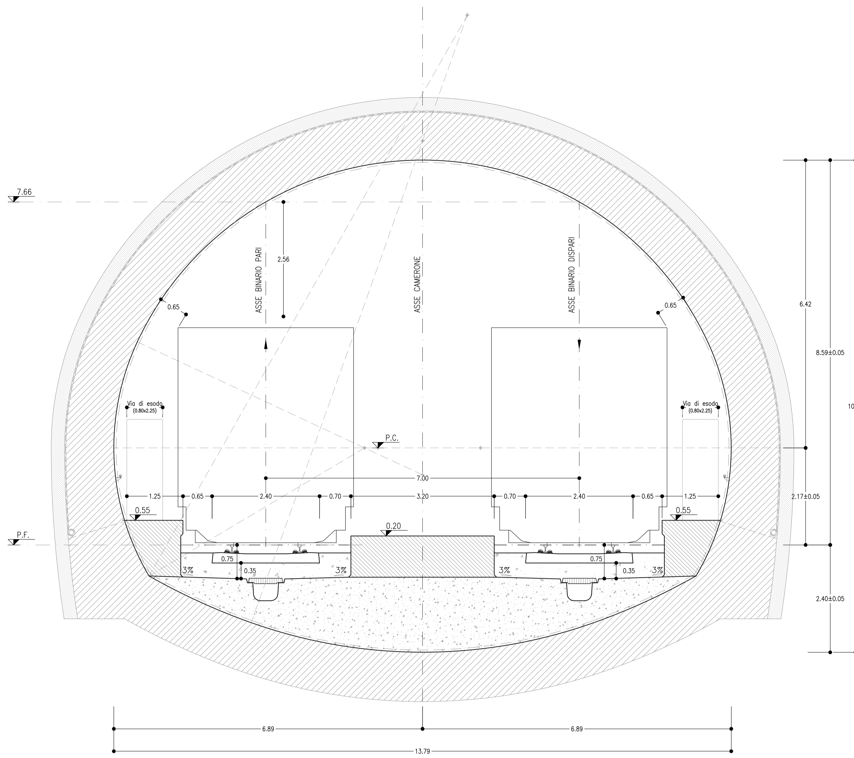
SEZIONE TIPO INTERASSE 5-7 SCALA 1:50
