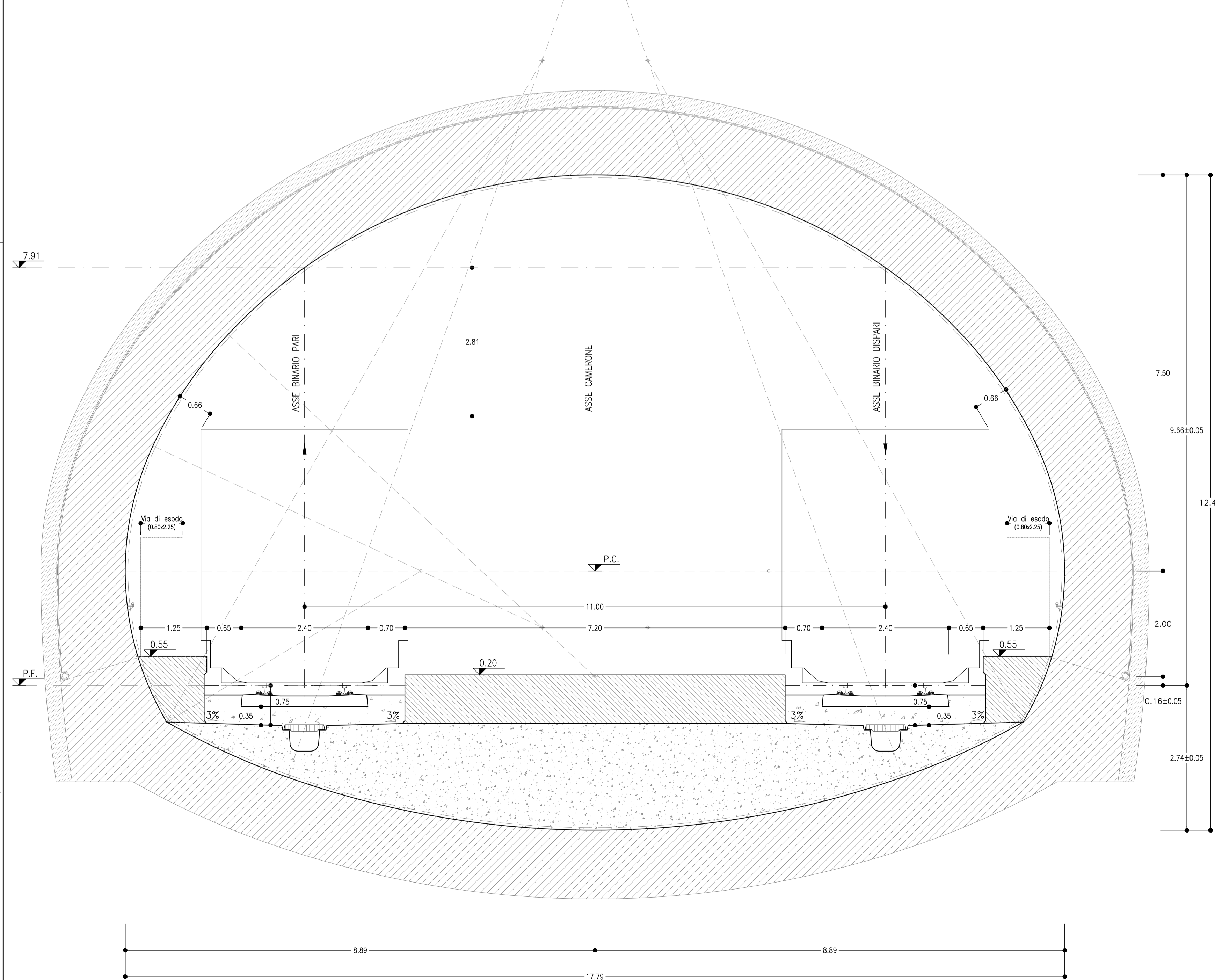
SEZIONE TIPO INTERASSE 9-11 SCALA 1:50
