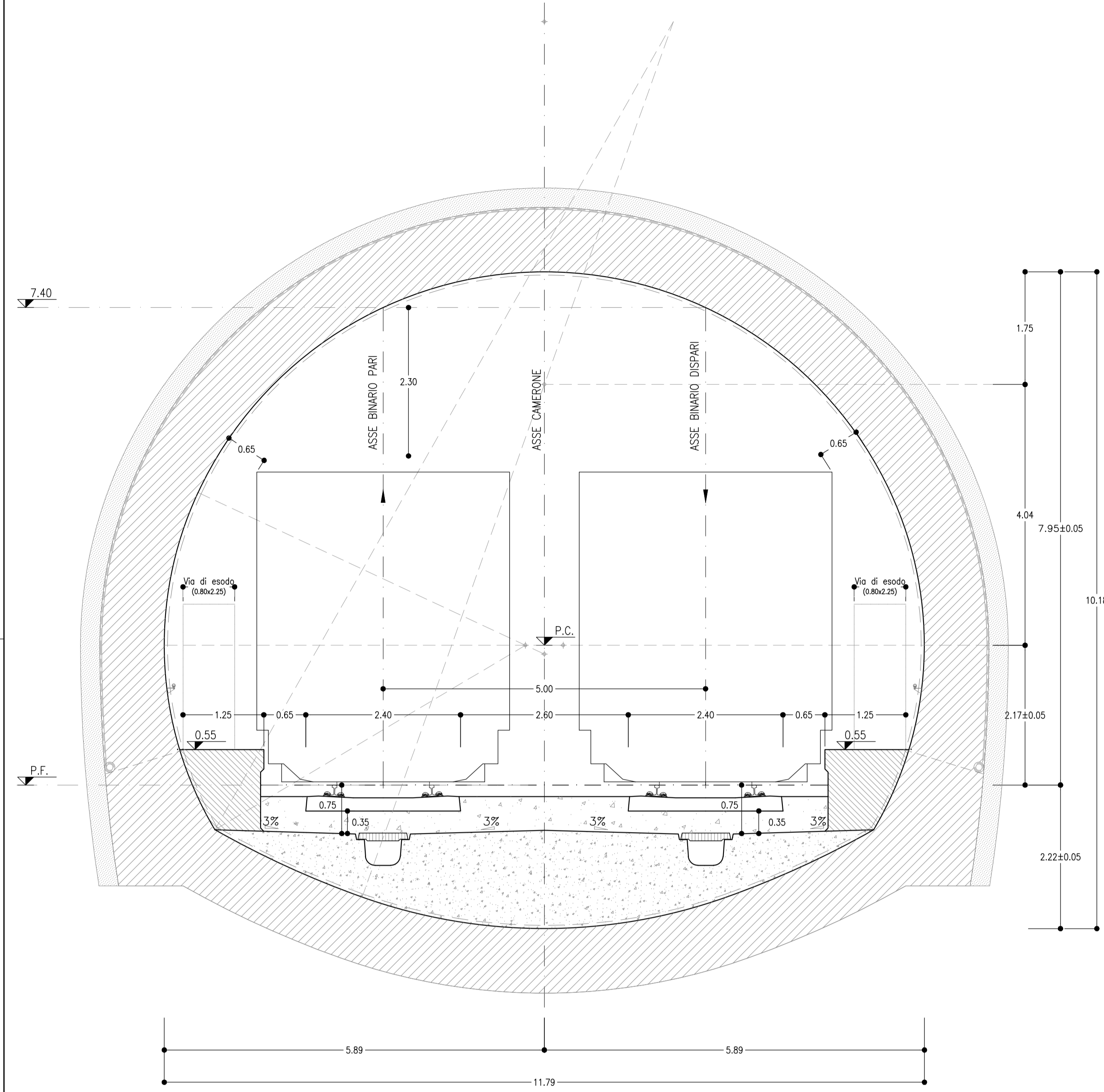
SEZIONE TIPO INTERASSE 4-5 SCALA 1:50
