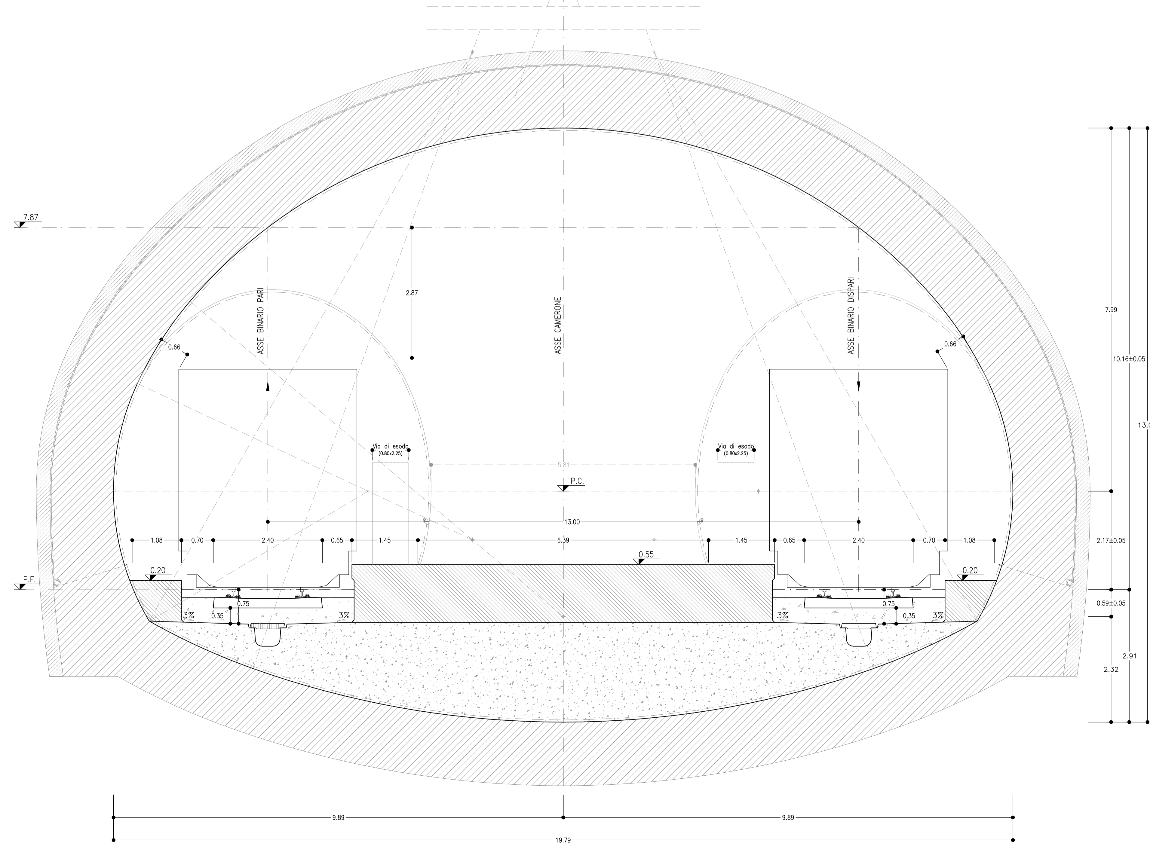
SEZIONE TIPO INTERASSE 11-13 SCALA 1:50
