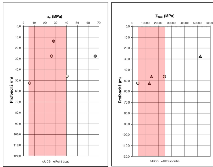
Figura 13 - Formazione PMAa: \sigma_{ci} e E_{tan,i} della matrice
