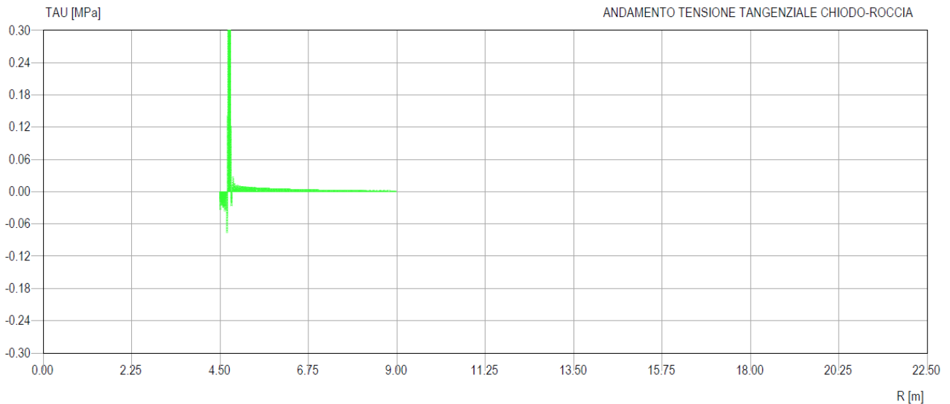
Figura 17 – Andamento delle tensioni lungo lo sviluppo dei bulloni radiali
