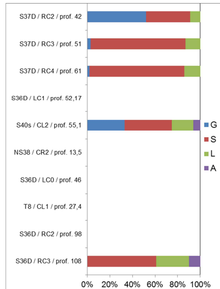
Figura 11 - PMAa: analisi granulometrica
