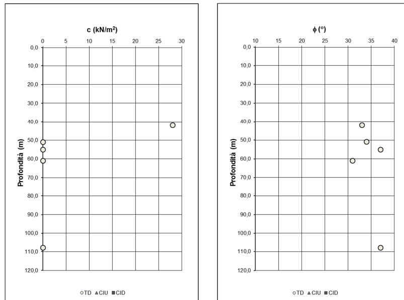
Figura 14 – Formazione PMAa: coesione drenata ed angolo di attrito
