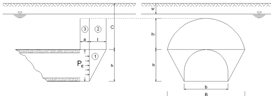
Figura 16. Stabilità del fronte secondo il Metodo di Tamez (1984).
