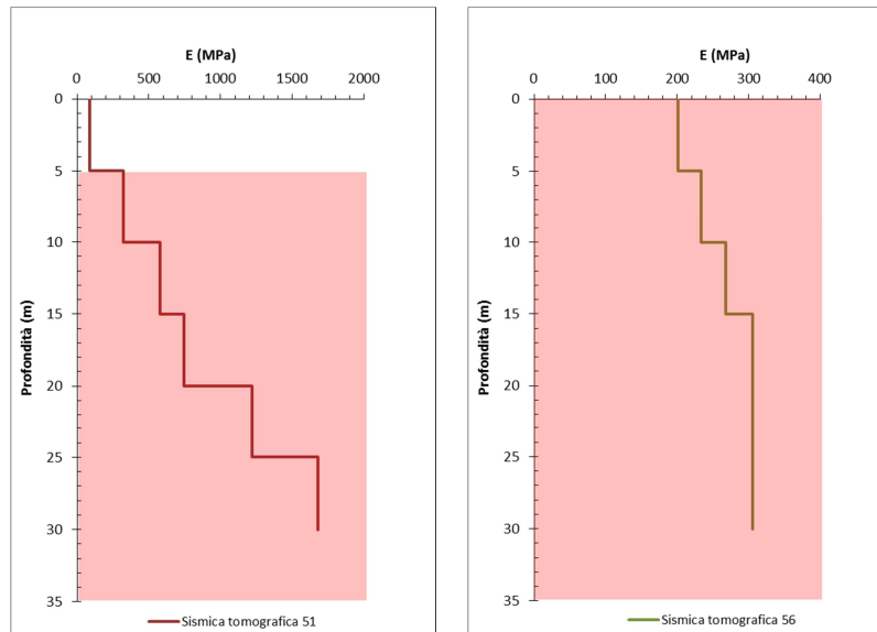
Figura 15 – Formazione PMAa: moduli elastici stimati dall’interpretazione delle indagini geofisiche
