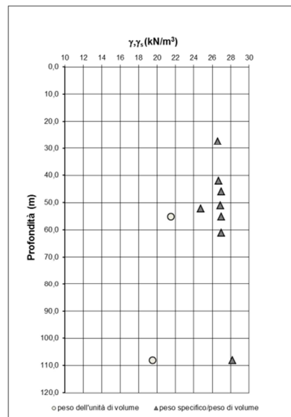
Figura 12 – Formazione PMAa: peso di volume \gamma
