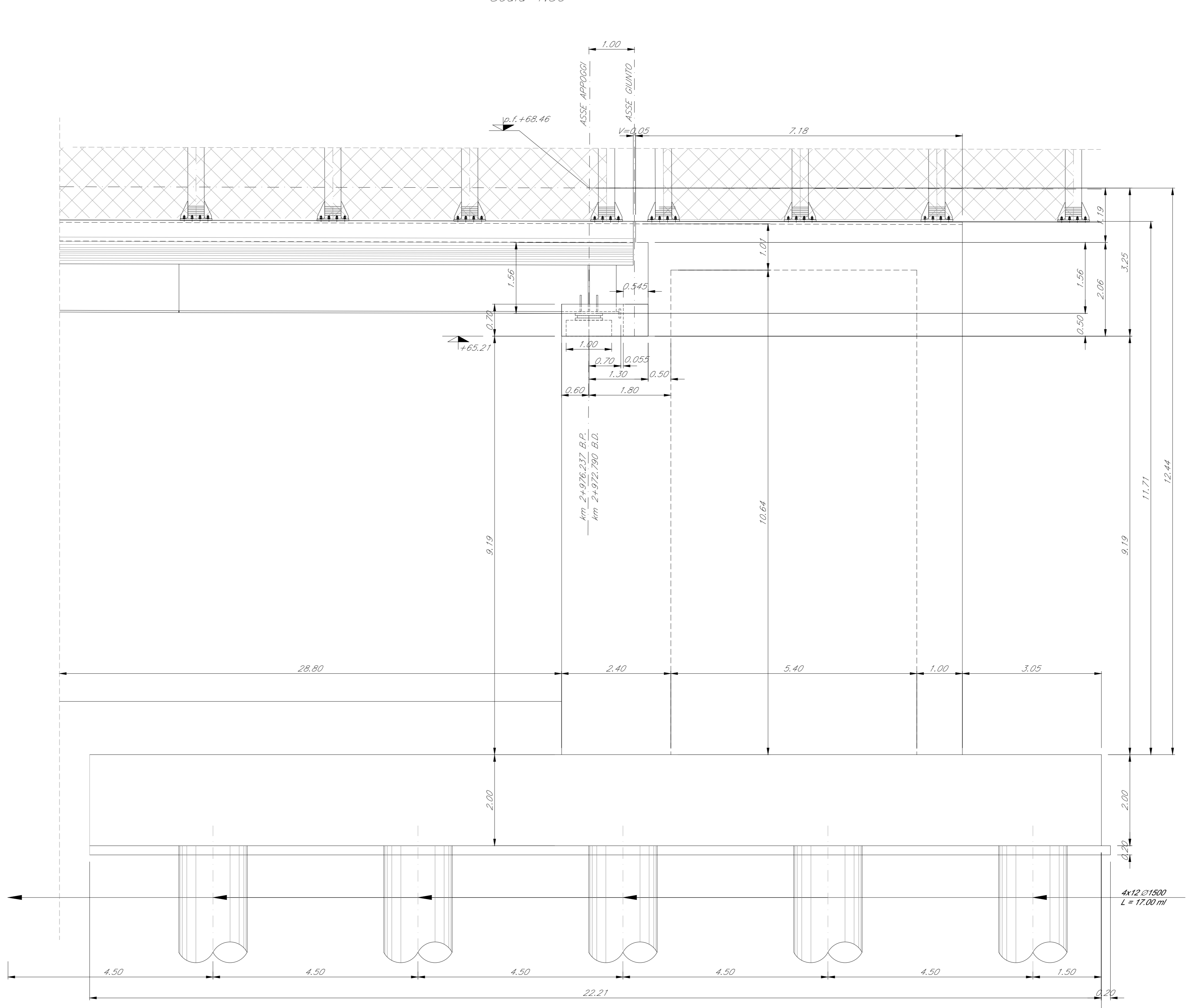
VISTA B-B Scala 1:50
