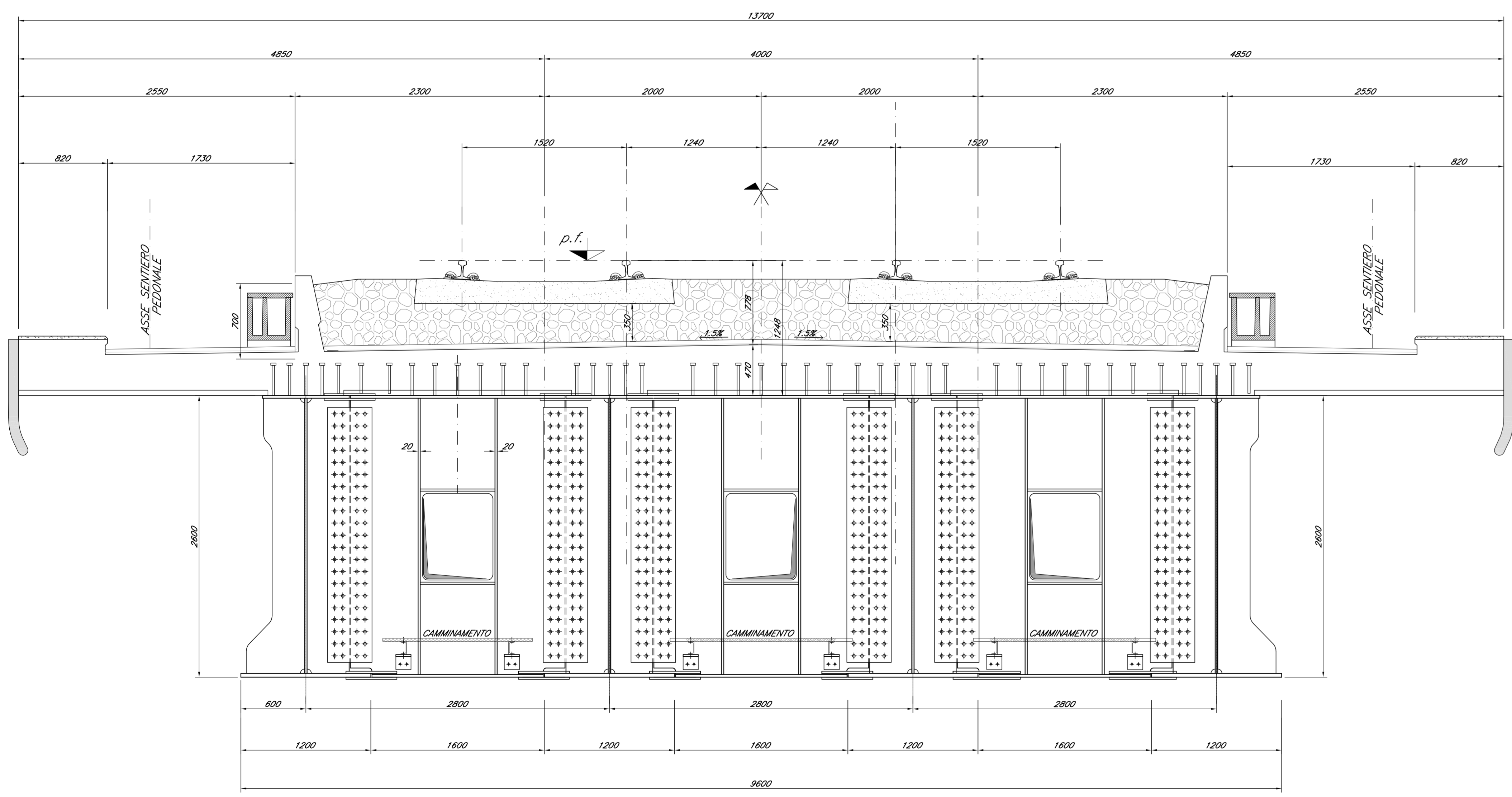
SEZIONE A-A DIAFRAMMA DI APPOGGIO Scala 1:20
