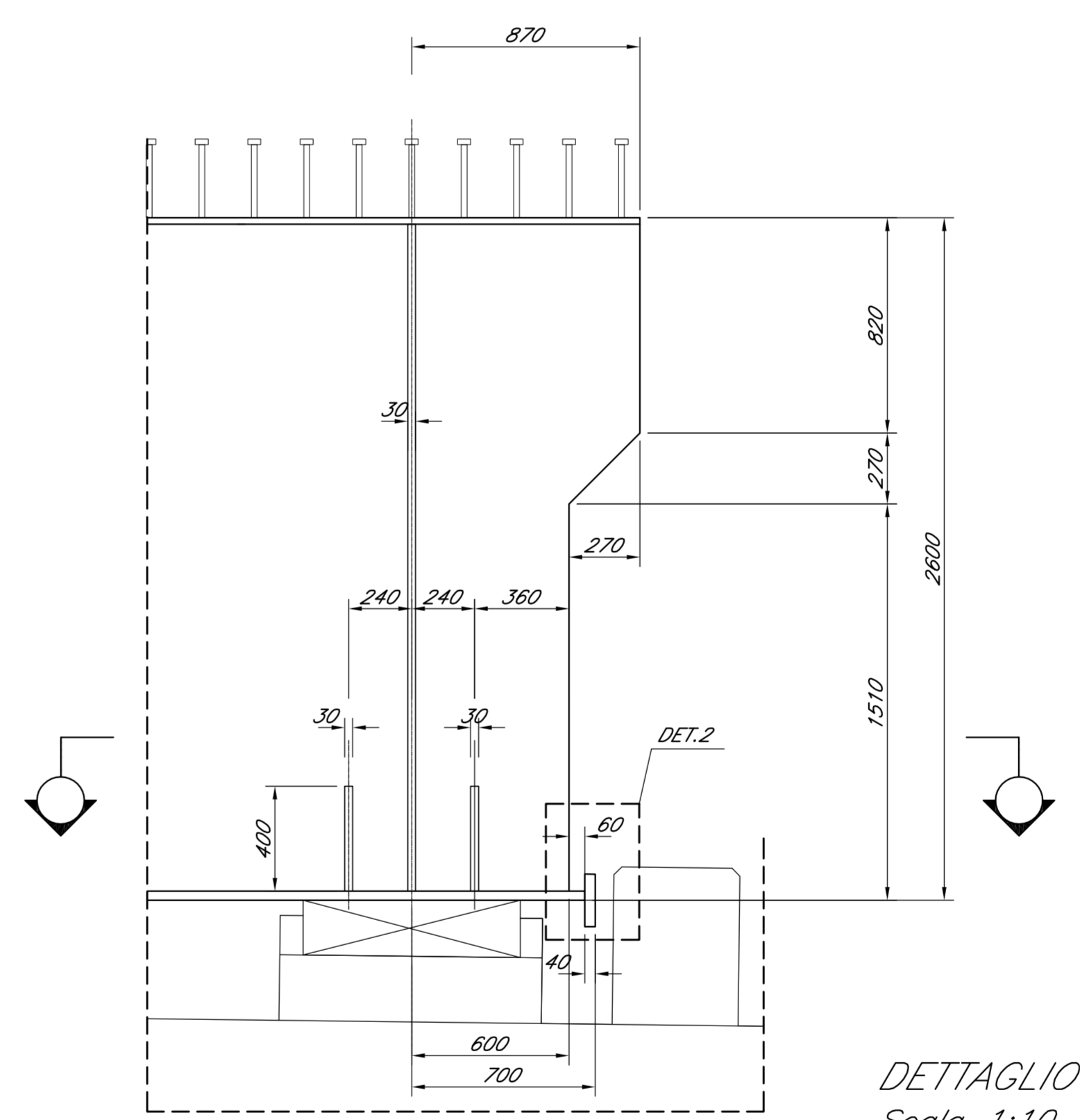
DETTAGLIO 1 Scala 1:20
