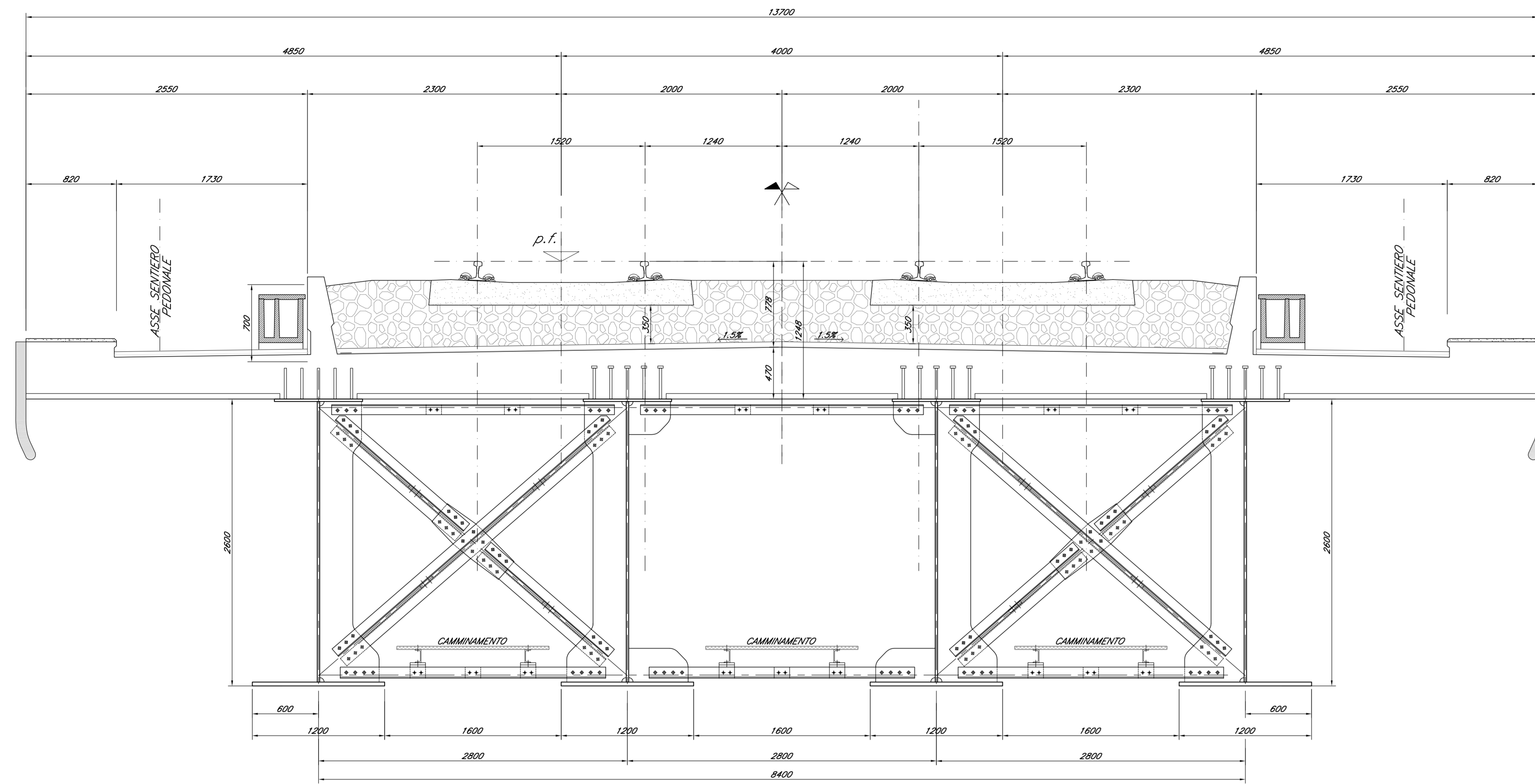
SEZIONE B-B DIAFRAMMA INTERMEDIO TIPO 1 Scala 1:20
