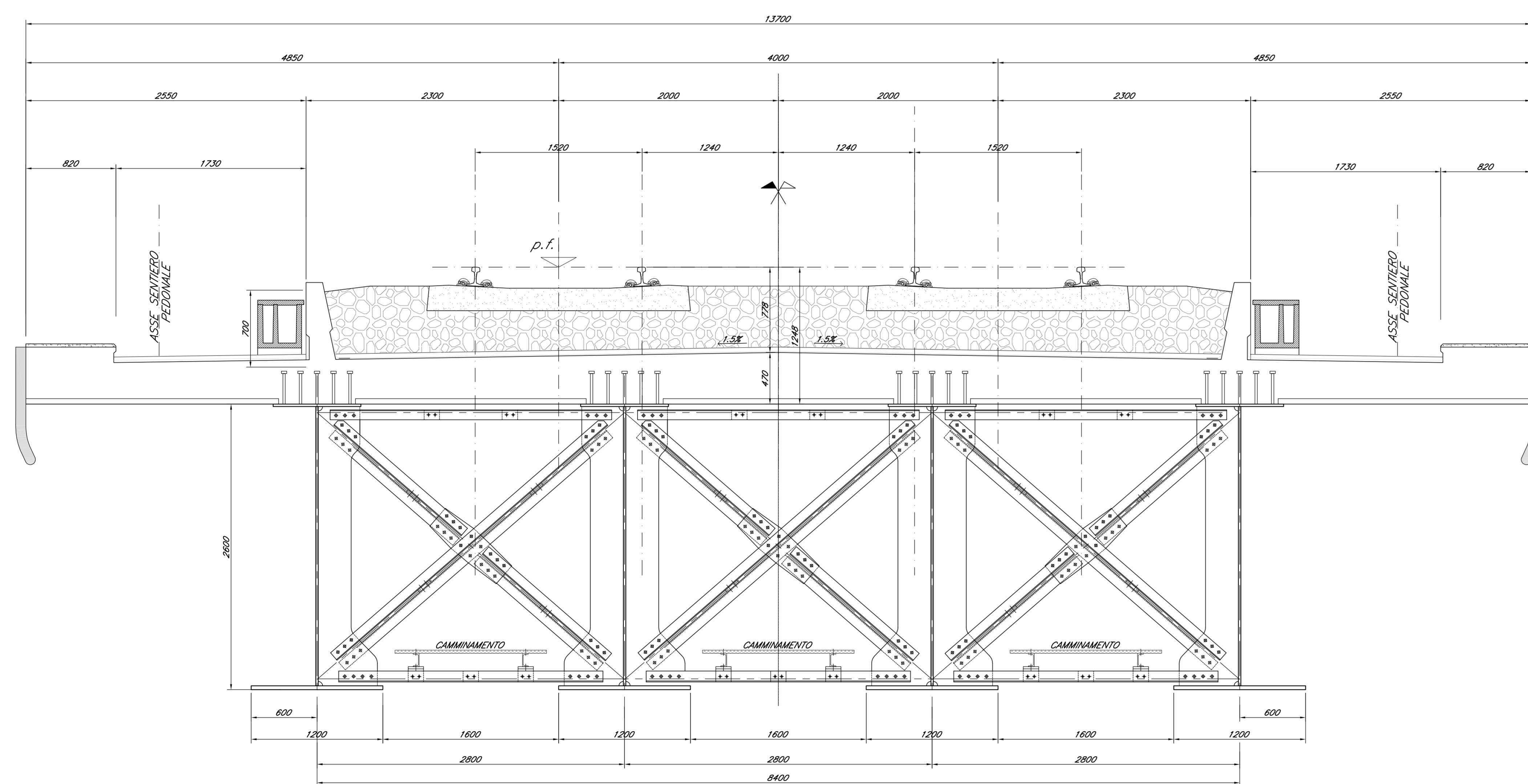
SEZIONE C-C DIAFRAMMA INTERMEDIO TIPO 2 Scala 1:20
