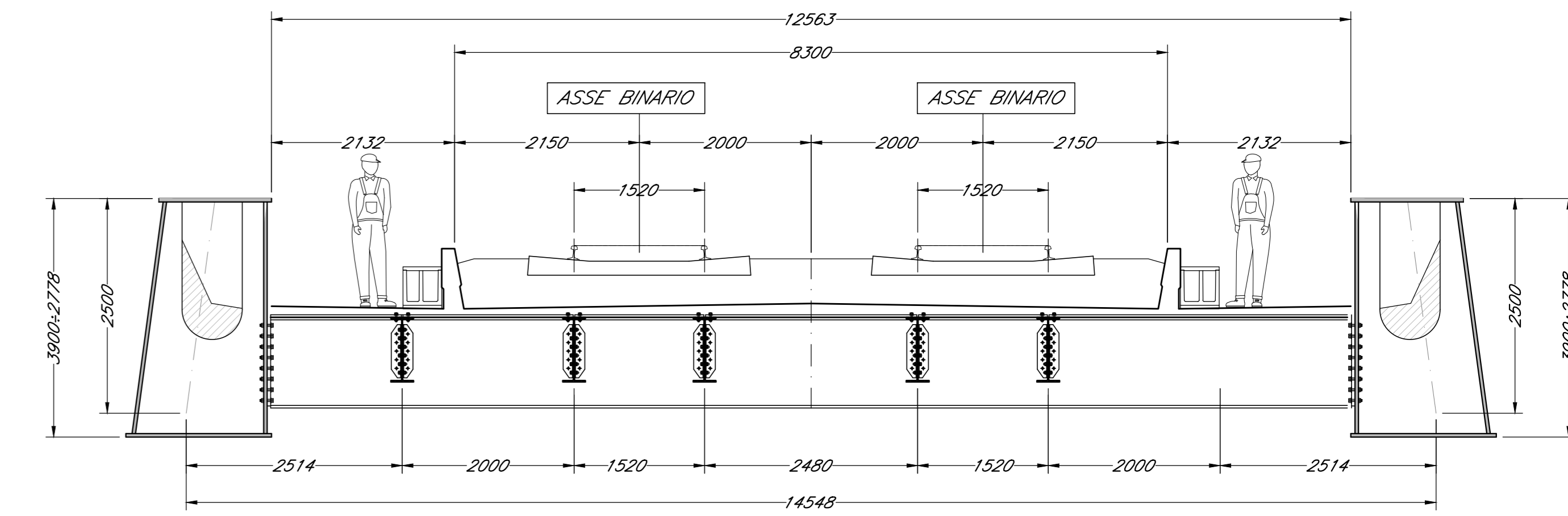
SEZIONE TRASVERSALE TIPOLOGICA (tratto sezione 1) Scala 1:100
