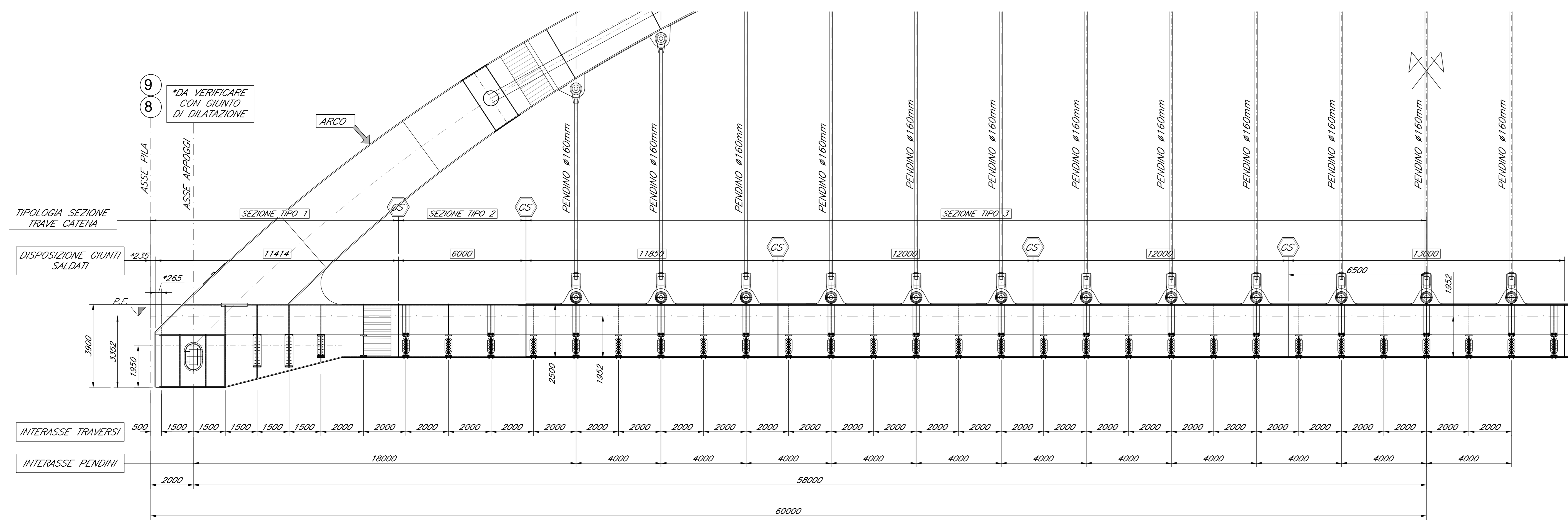
1/2 SEZIONE LONGITUDINALE IMPALCATO Scala 1:100
