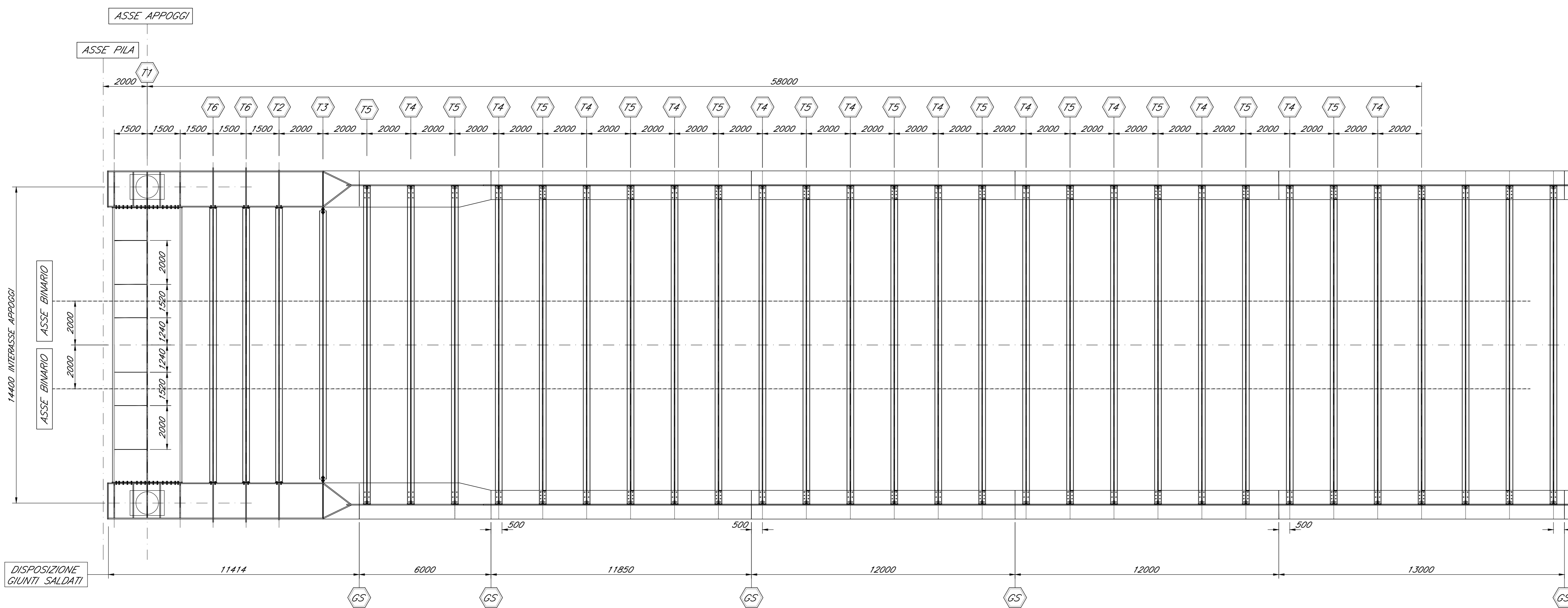
1/2PIANTA LIVELLO INTRADOSSO TRAVERSI Scala 1:100
