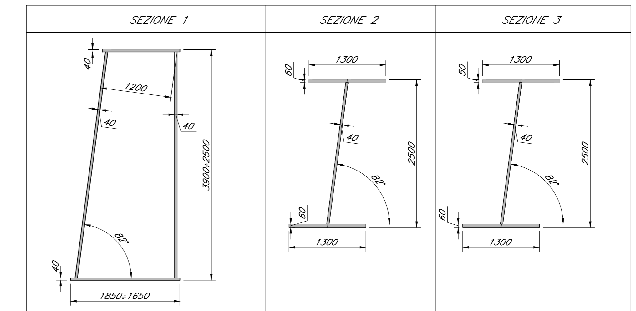
TIPOLOGIA CONCI TRAVE CATENA
