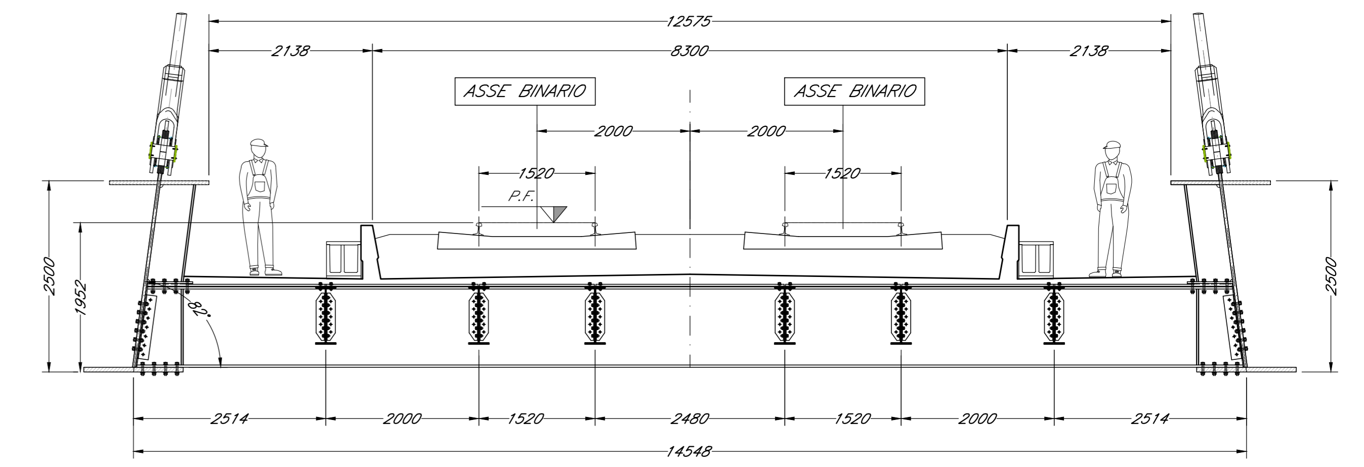
SEZIONE TRASVERSALE TIPOLOGICA (tratto sezione 3) Scala 1:100
