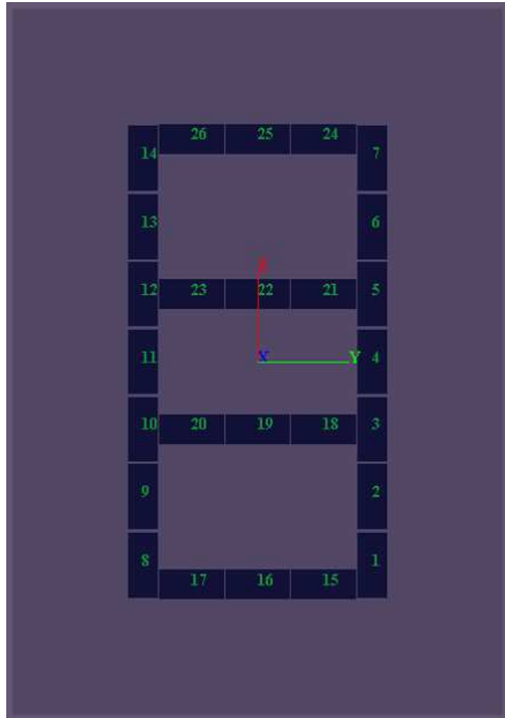
Figura 12: Vista planimetrica del modello GROUPv2016.
