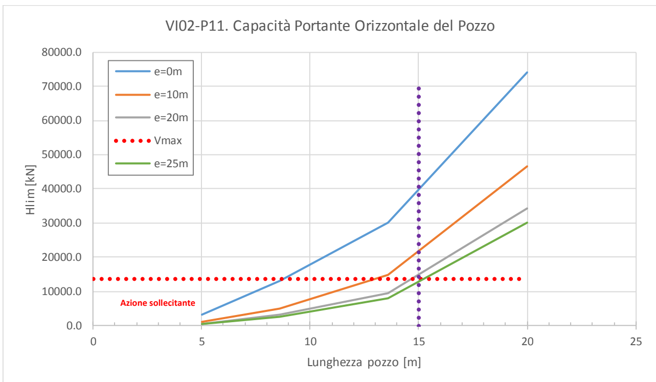
Figura 21: Diagrammi di capacità portante orizzontale del Pozzo.
