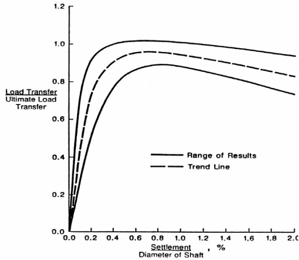
Figura 7: Argille. Curva di trasferimento laterale
