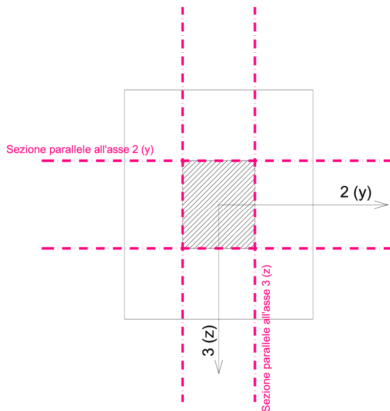
Figura 22: Sezioni in cui sono state determinate le sollecitazioni flessionali e di taglio.
