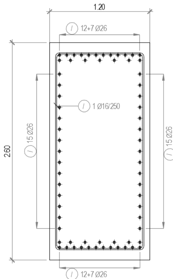
Figura 19: Armatura diaframmi.
