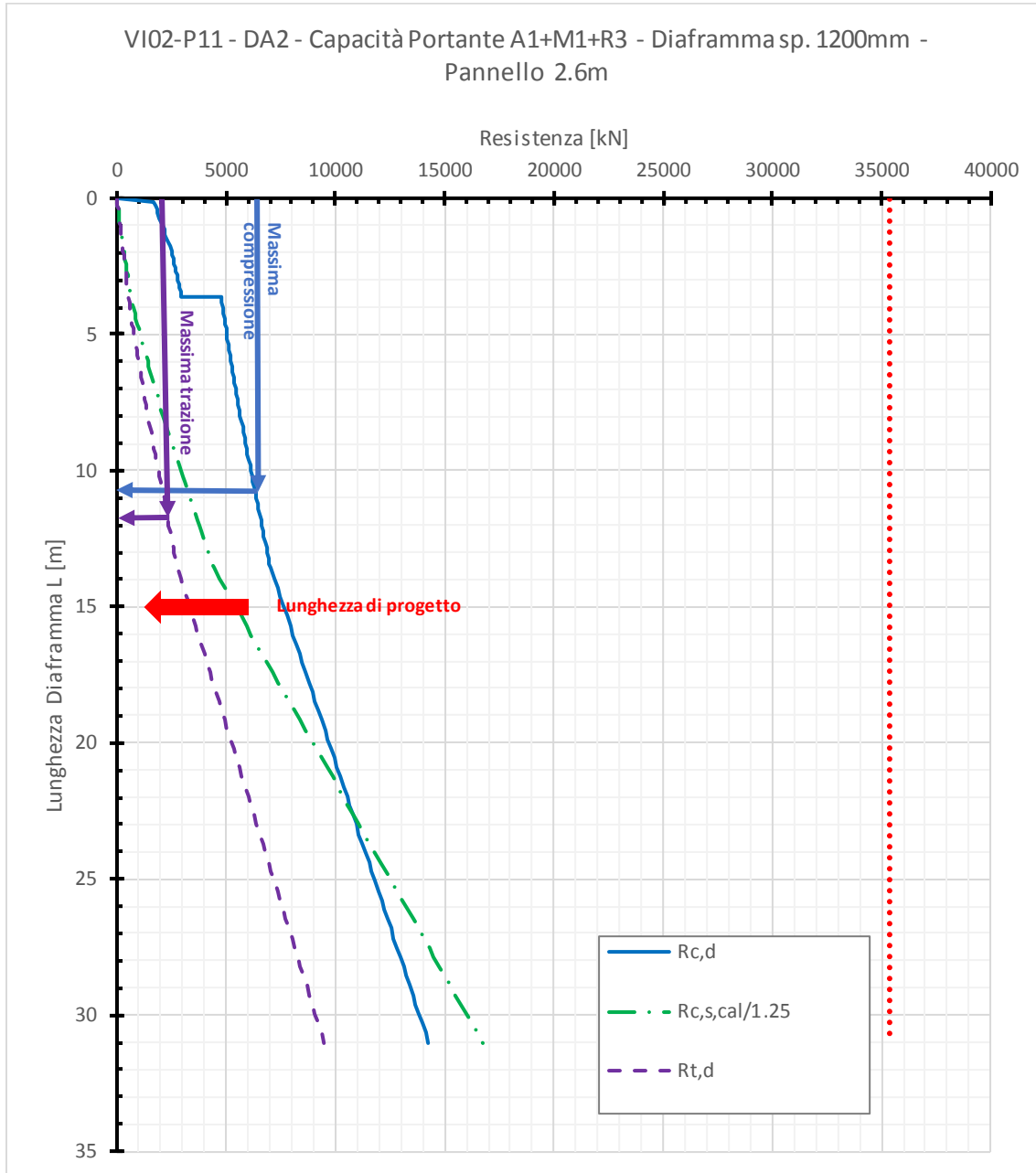
Figura 20: Capacità portante del diaframma singolo
