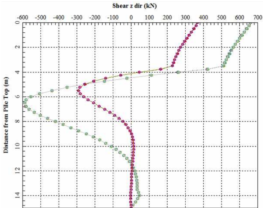
Figura 18: Combinazione sismica SLV: Andamento con la profondità del taglio.
