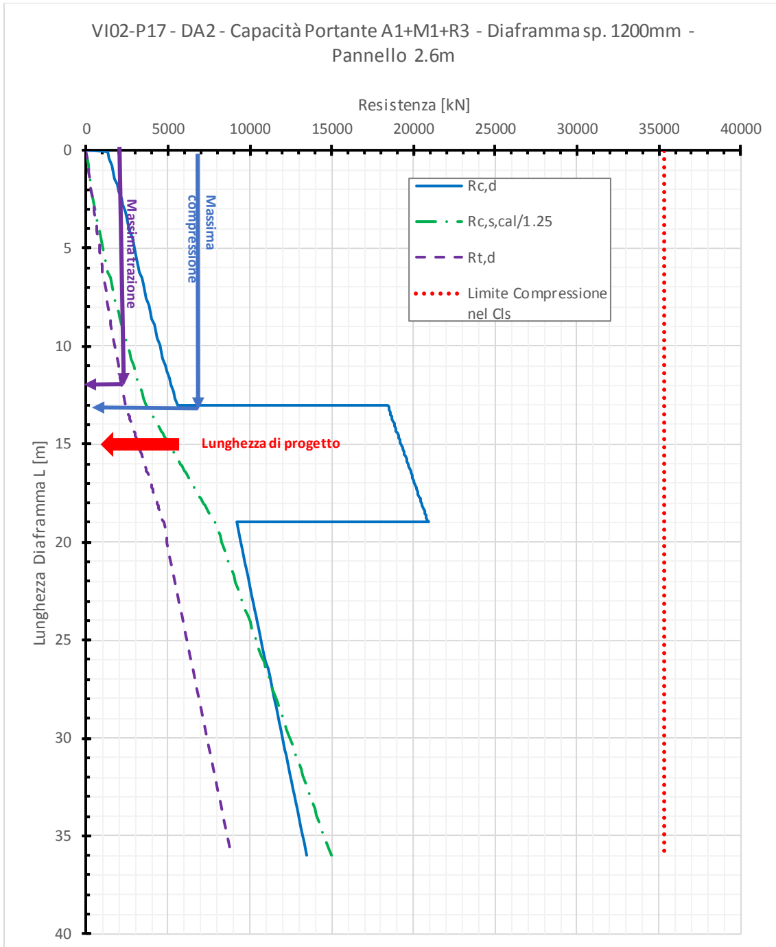
Figura 20: Capacità portante del diaframma singolo
