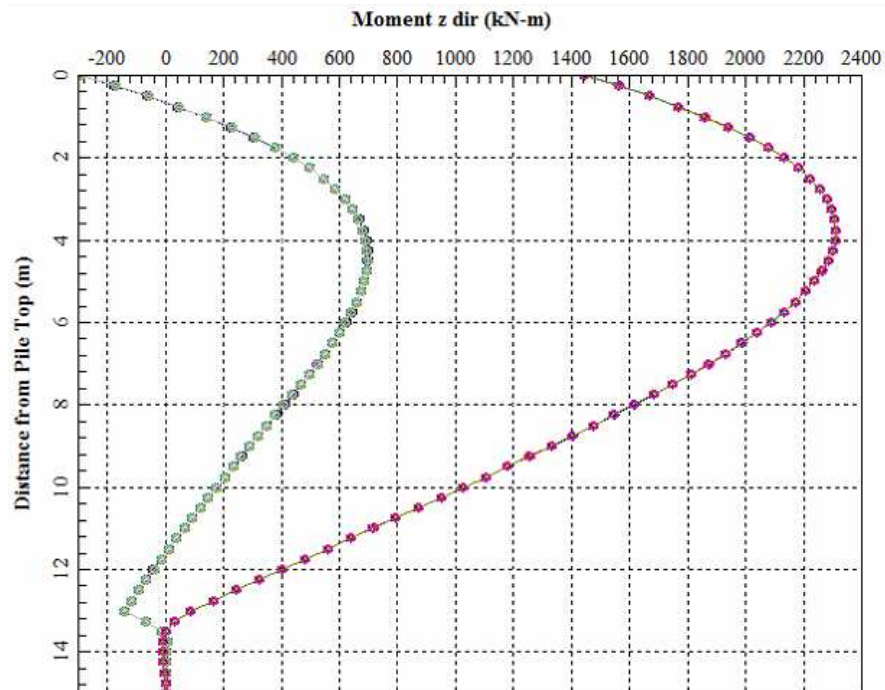
Figura 17: Combinazione sismica SLV: Andamento con la profondità del momento
