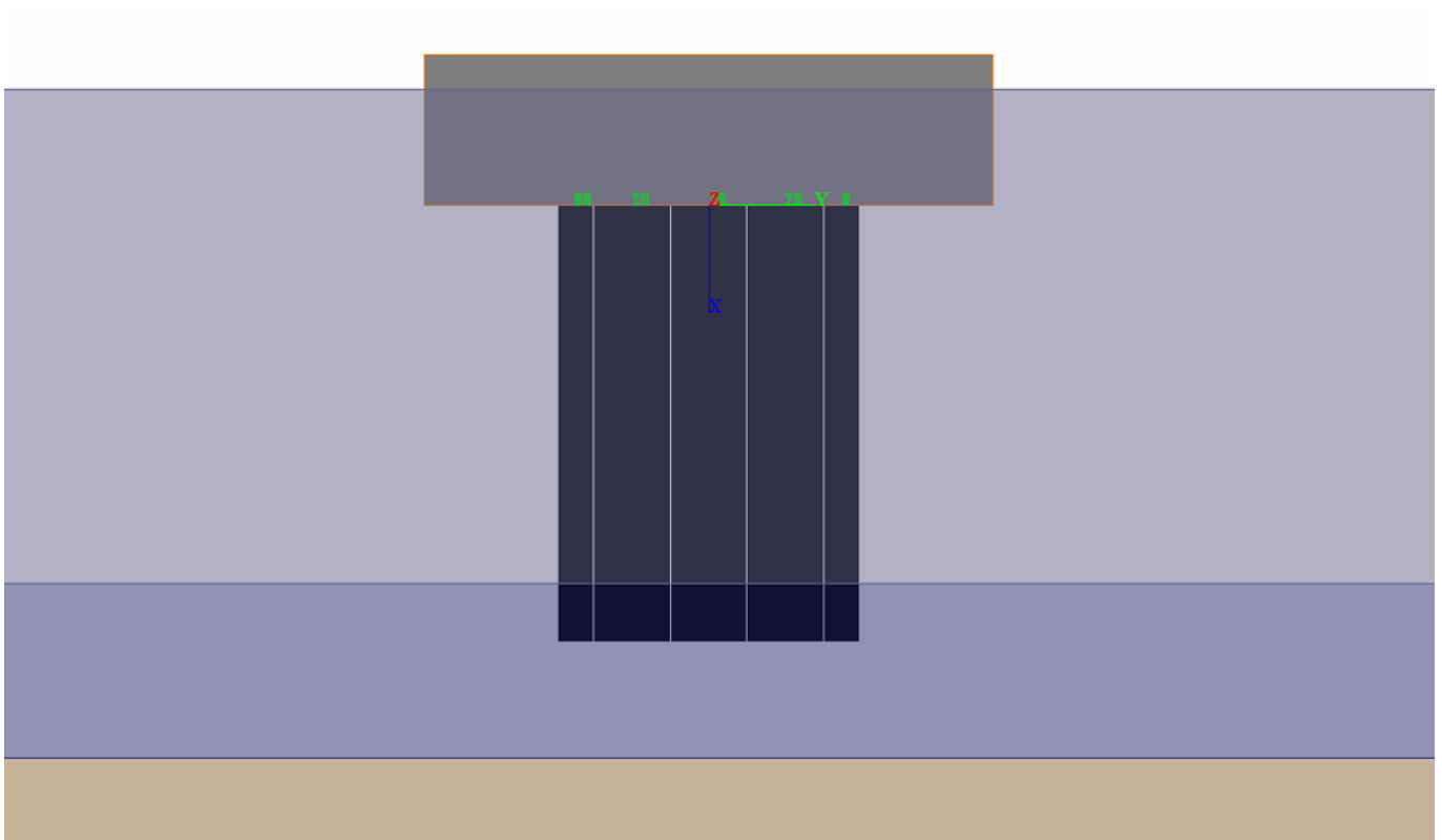
Figura 11: Vista frontale del modello GROUPv2016.
